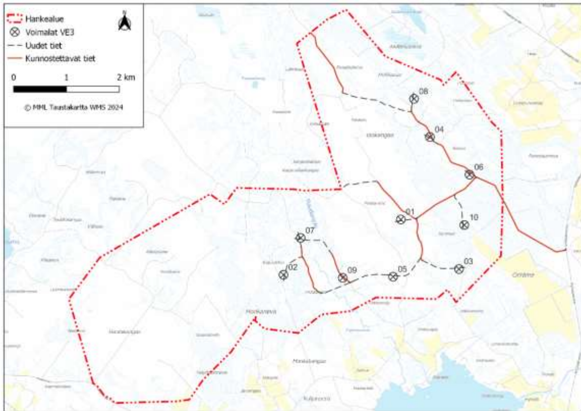
Kuva 4. Uusimaa tuulivoimapuiston alustava voimalasijoittelu vaihtoehdossa VE3.
