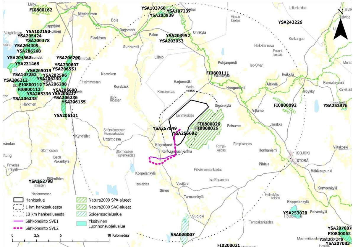
Kuva 2-1. Kasvillisuus- ja luontotyyppiselvityksen lähtötiedot (Ramboll 2024). Kuvassa esitetyt sähkönsiirto-reitti ovat vuoden 2024 luontoselvityksen aikaiset vaihtoehdot.
