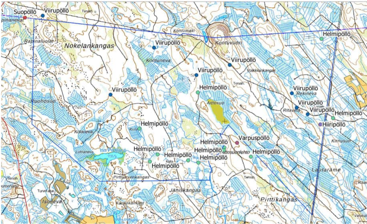
Kuva 20. Pöllöhavainnot.
