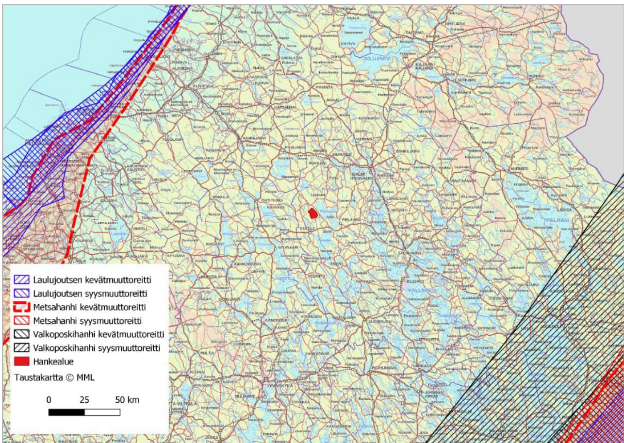
Kuva 62. Hankealueen sijoittuminen suhteessa lintujen valtakunnallisiin päämuuttoreitteihin (punainen = metsähanhen päämuuttoreitti, sininen = laulujoutsenen päämuuttoreitti ja musta = valkoposkihanhen päämuuttoreitti). Aineisto Toivanen ym. 2014.
