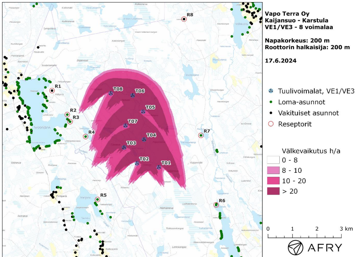
Kuva 9: Suunnitelman VE1/VE3 todennäköinen vuotuinen välkevaikutus ilman puuston vaikutusta.
