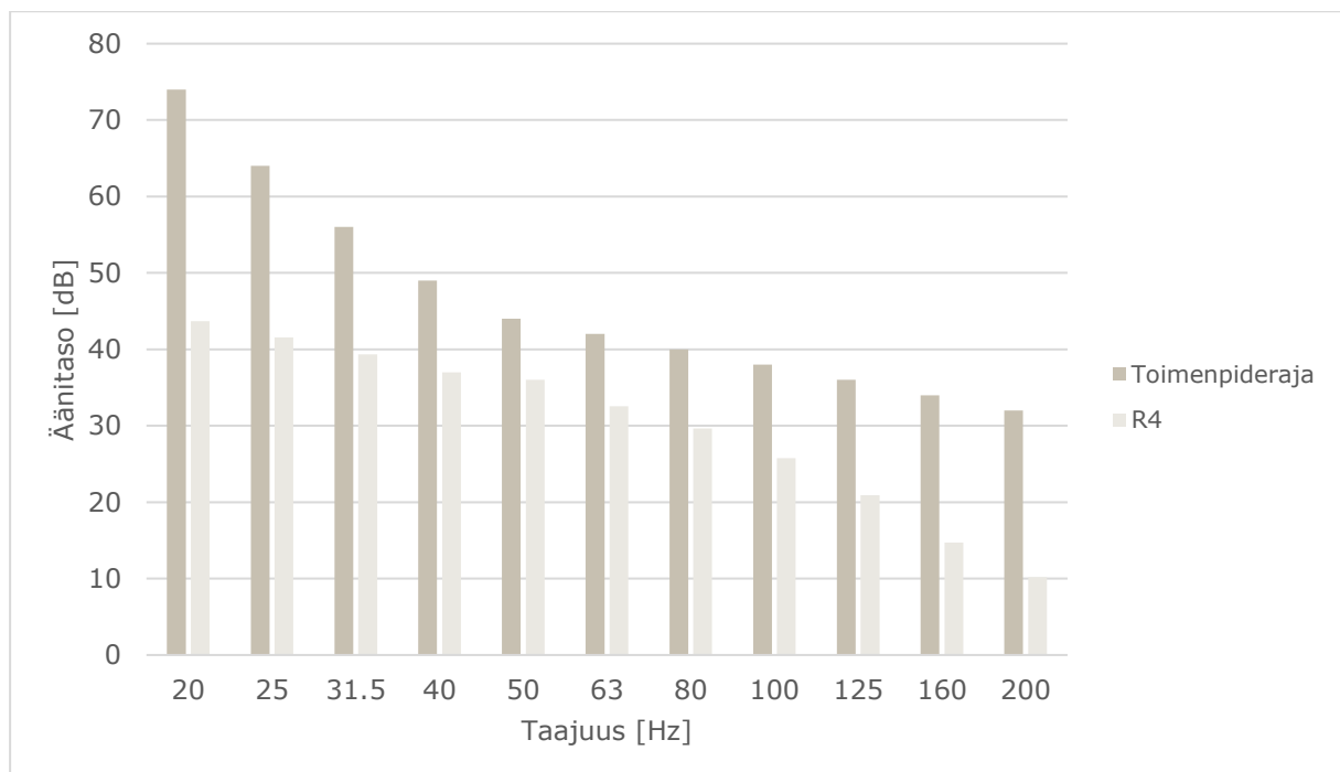
Kuva 8: Matalataajuisen sisämelun tasot reseptorin R4 kohdalla suunnitelmalla VE2.
