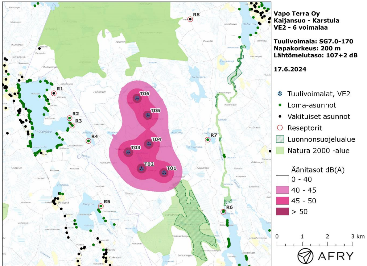
Kuva 6: Keskiäänitasot LAeq Kajiansuon tuulivoimapaiston suunnitelmalla VE2.
