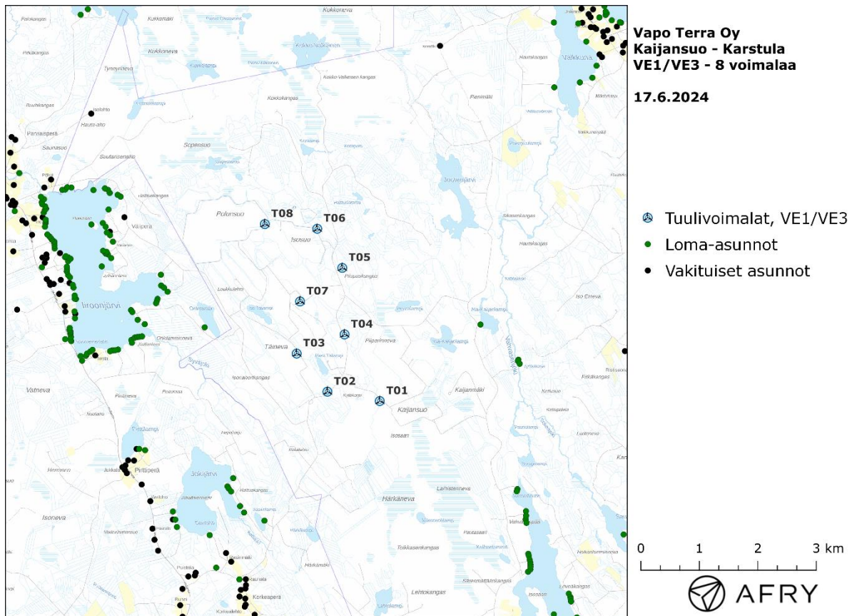
Kuva 1: Tuulivoimaloiden sijainnit Kaijansuon suunnitelmalla VE1/VE3.
