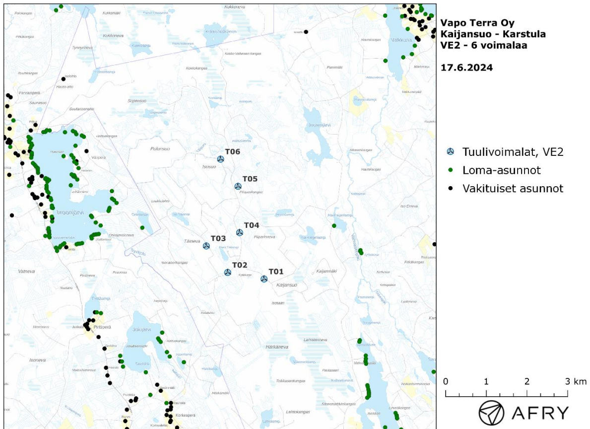
Kuva 2: Tuulivoimaloiden sijainnit Kaijansuon suunnitelmalla VE2.
