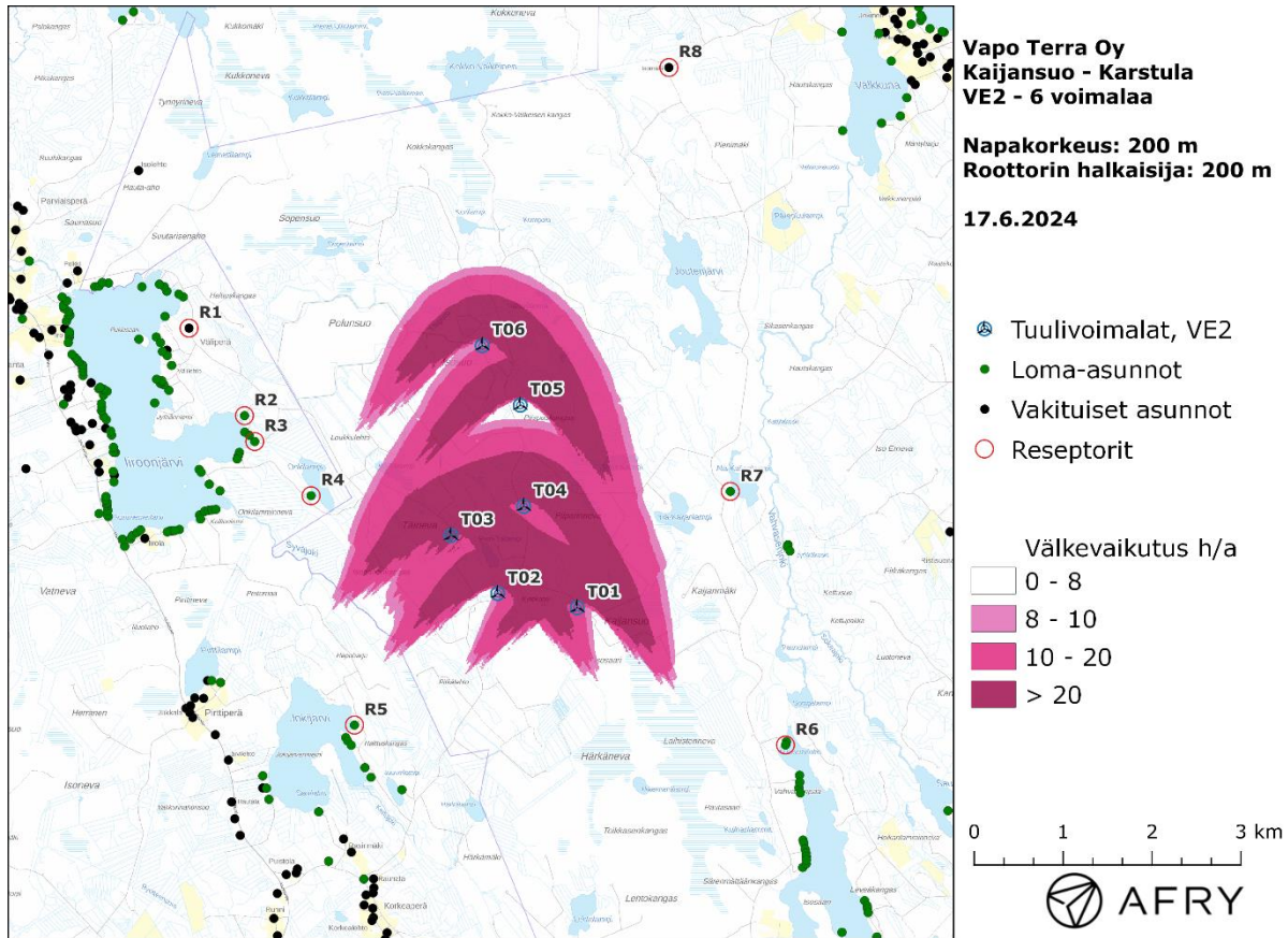
Kuva 10: Suunnitelman VE2 todennäköinen vuotuinen välkevaikutus ilman puuston vaikutusta.
