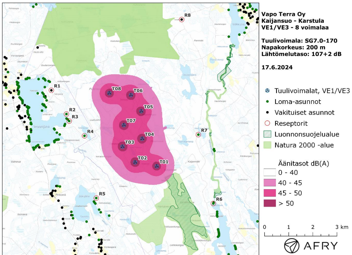
Kuva 5: Keskiäänitasot L_{Aeq} Kajiansuon tuulivoimapaiston suunnitelmalla VE1/VE3.
