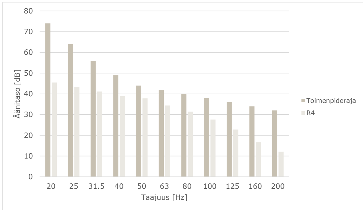
Kuva 7: Matalataajuisen sisämelun tasot reseptorin R4 kohdalla suunnitelmalla VE1/VE3.
