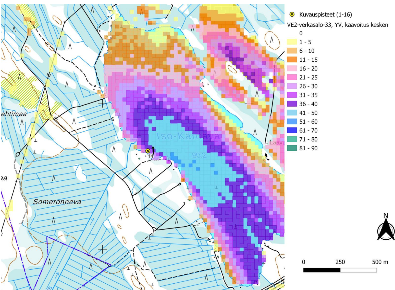
Kuva 113. Kuvauspiste 14. Verkasalon voimalat layout VE2 ja lähialueen hankkeet, joissa kaavoitus on kesken. Näkymäalueanalyysin laskentatulokset voimaloiden napakorkeudella mallinnettuna. (Oikea)
