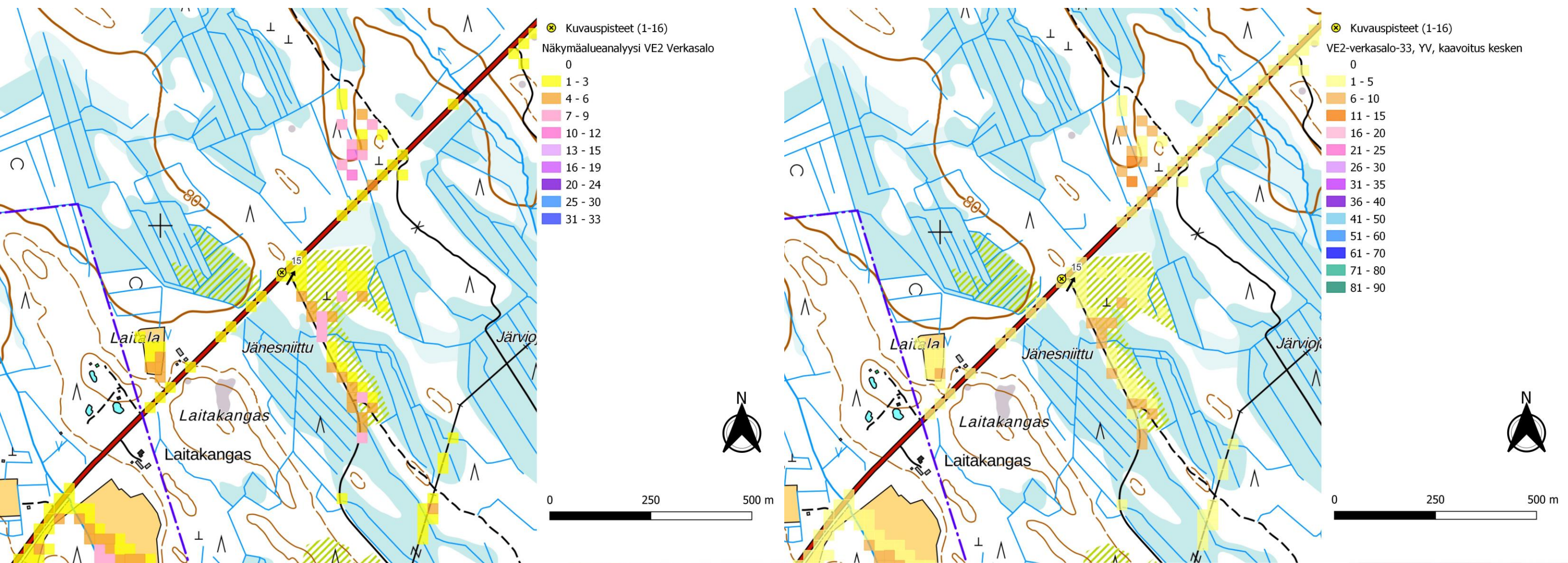
Kuva 120. Kuvauspiste 15. Verkasalon voimalat layout VE2. Näkymäalueanalyysin laskentatulokset voimaloiden napakorkeudella mallinnettuna. (Vasen)
