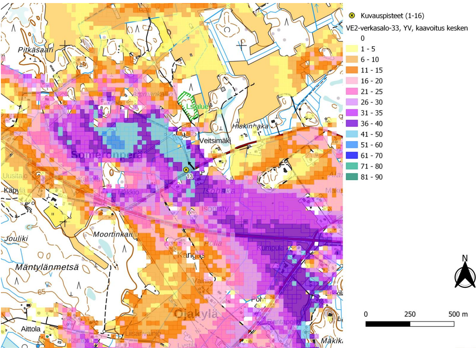
Kuva 105. Kuvauspiste 13. Verkasalon voimalat layout VE2 ja lähialueen hankkeet, joissa kaavoitus on kesken. Näkymäalueanalyysin laskentatulokset voimaloiden napakorkeudella mallinnettuna. (Oikea)
