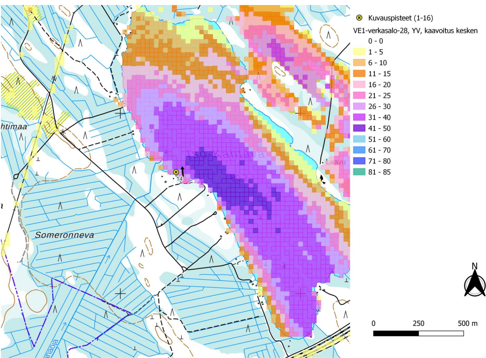
Kuva 109. Kuvauspiste 14. Verkasalon voimalat layout VE1 ja lähialueen hankkeet, joissa kaavoitus on kesken. Näkymäalueanalyysin laskentatulokset voimaloiden napakorkeudella mallinnettuna. (Oikea)
