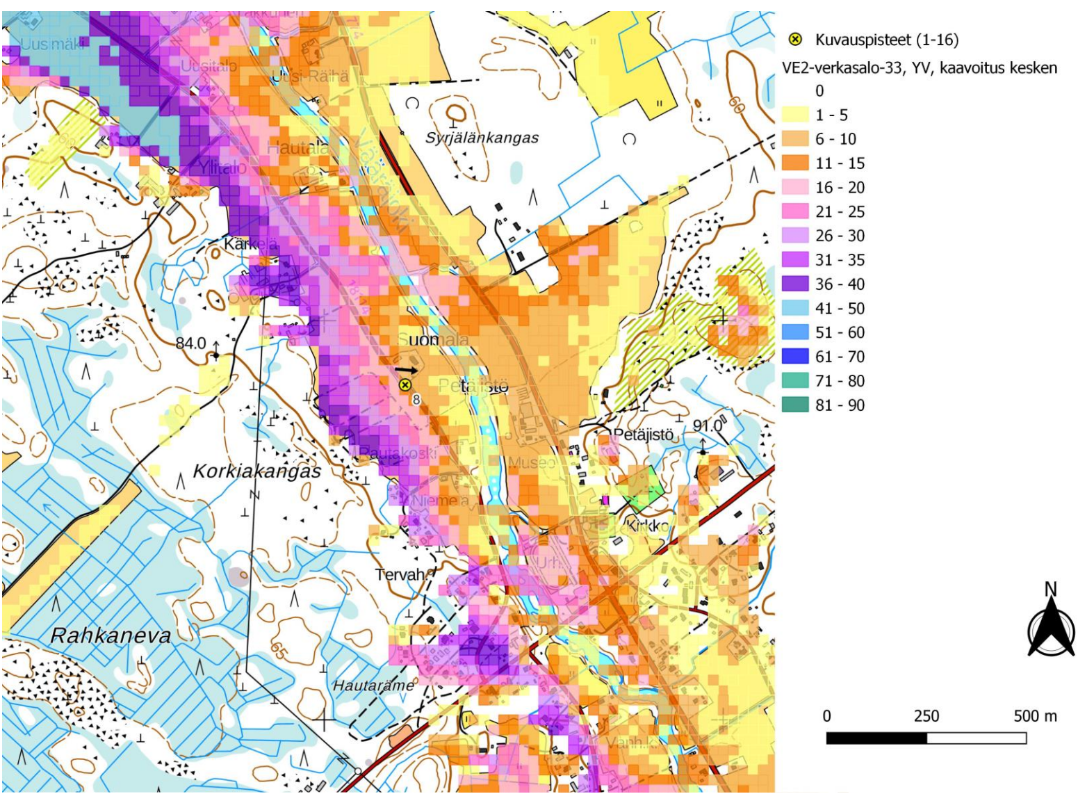
Kuva 66. Kuvauspiste 8. Verkasalon voimalat layout VE2 ja lähialueen hankkeet, joissa kaavoitus on kesken. Näkymäalueanalyysin laskentatulokset voimaloiden napakorkeudella mallinnettuna. (Oikea)
