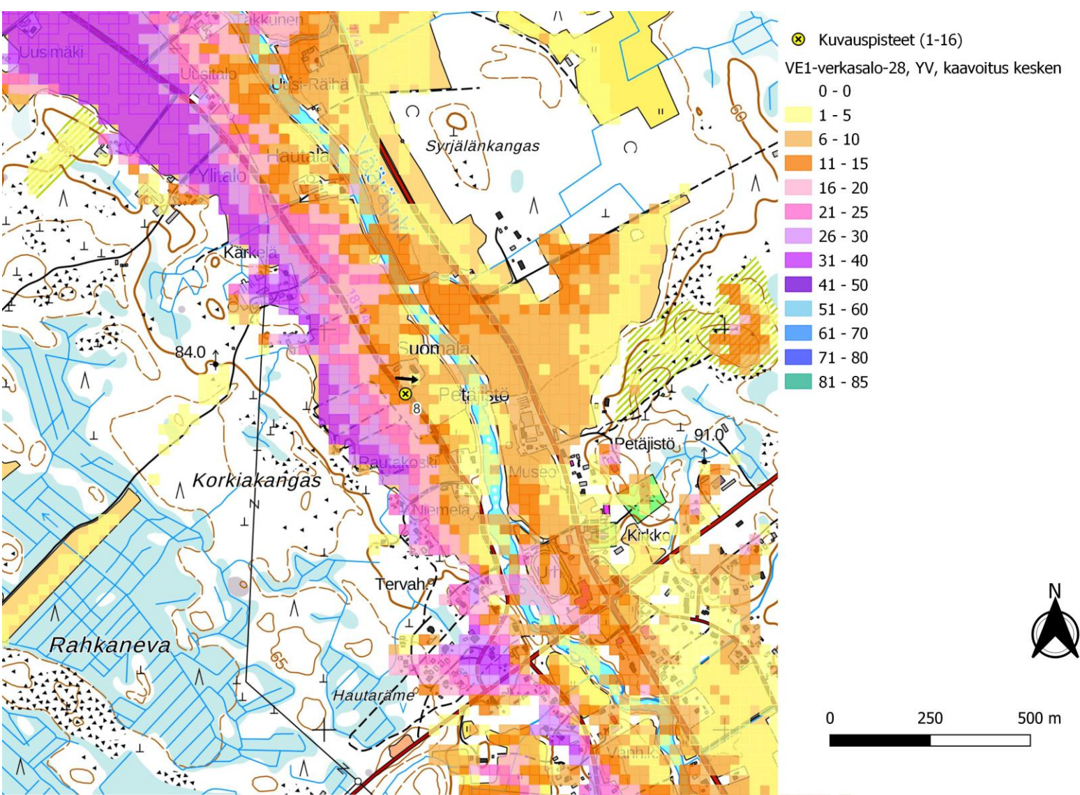
Kuva 62. Kuvauspiste 8. Verkasalon voimalat layout VE1 ja lähialueen hankkeet, joissa kaavoitus on kesken. Näkymäalueanalyysin laskentatulokset voimaloiden napakorkeudella mallinnettuna. (Oikea)
