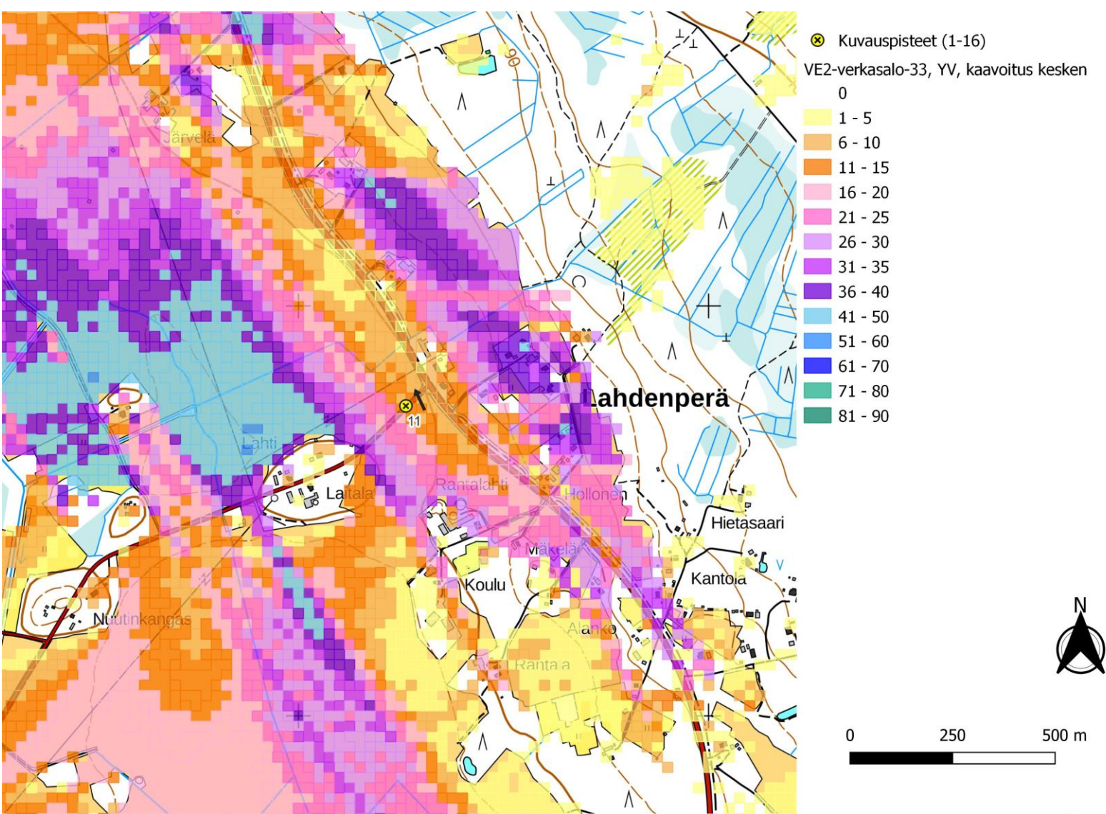
Kuva 89. Kuvauspiste 11. Verkasalon voimalat layout VE2 jaa lähialueen hankkeet, joissa kaavoitus on kesken. Näkymäalueanalyysin laskentatulokset voimaloiden napakorkeudella mallinnettuna. (Oikea)
