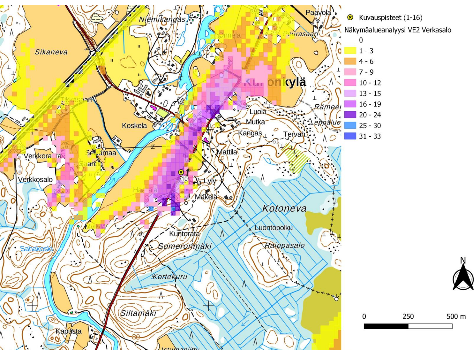
Kuva 81. Kuvauspaiste 10. Verkasalon voimalat layout VE2. Näkymäalueanalyysin laskentatulokset voimaloiden napakorkeudella mallinnettuna. (Vasen)
