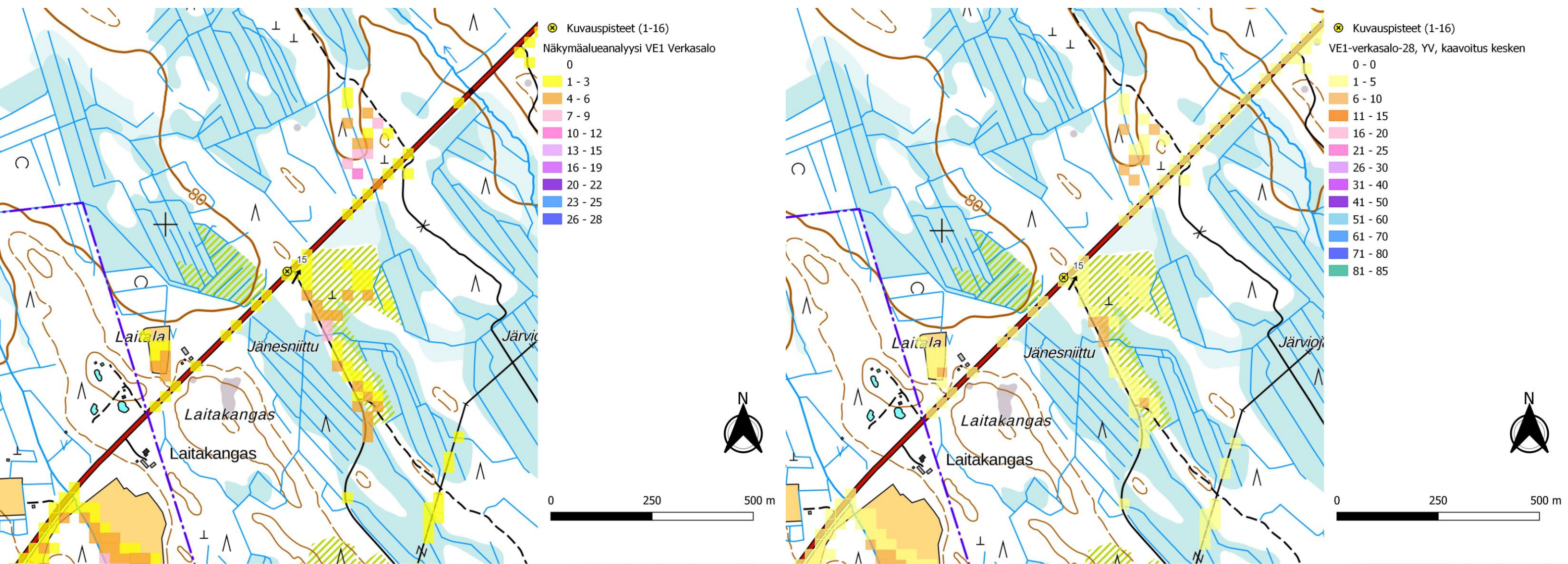
Kuva 116. Kuvauspiste 15. Verkasalon voimalat layout VE1. Näkymäalueanalyysin laskentatulokset voimaloiden napakorkeudella mallinnettuna. (Vasen)
