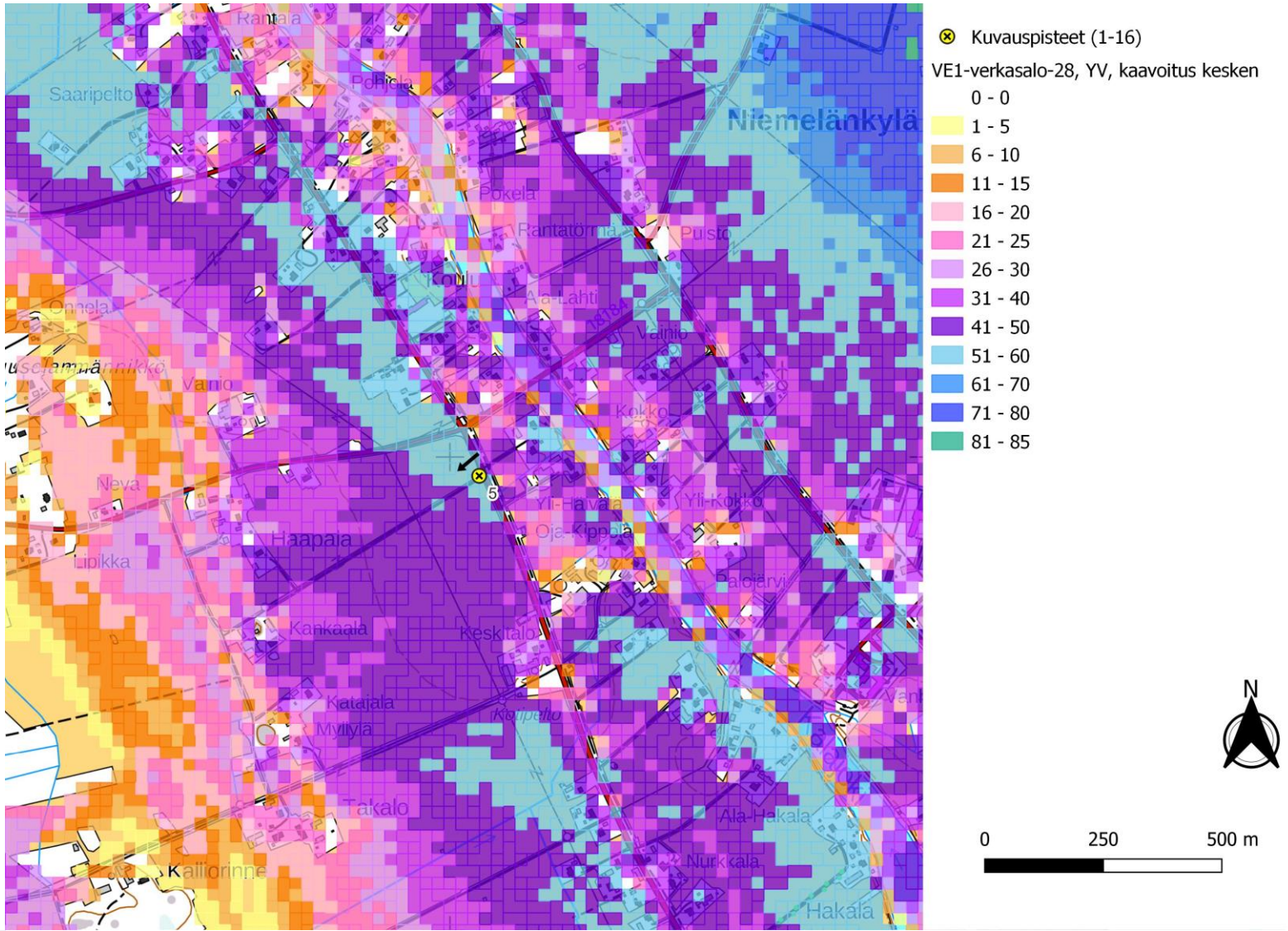
Kuva 38. Kuvauspiste 5. Verkasalon voimalat layout VE1 ja lähialueen hankkeet, joissa kaavoitus on kesken. Näkymäalueanalyysin laskentatulokset voimaloiden napakorkeudella mallinnettuna. (Oikea)
