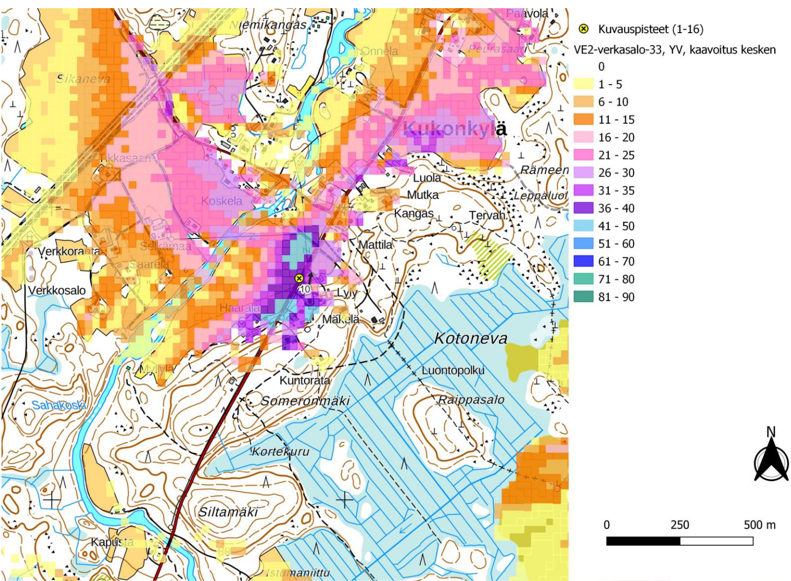
Kuva 82. Kuvauspaiste 10. Verkasalon voimalat layout VE2 ja lähialueen hankkeet, joissa kaavoitus on kesken. Näkymäalueanalyysin laskentatulokset voimaloiden napakorkeudella mallinnettuna. (Oikea)
