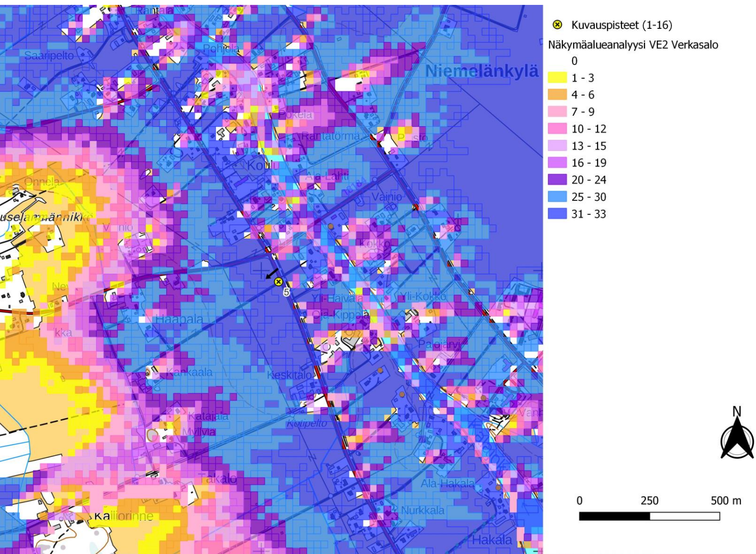
Kuva 41. Kuvauspiste 5. Verkasalon voimalat layout VE2. Näkymäalueanalyysin laskentatulokset voimaloiden napakorkeudella mallinnettuna. (Vasen)
