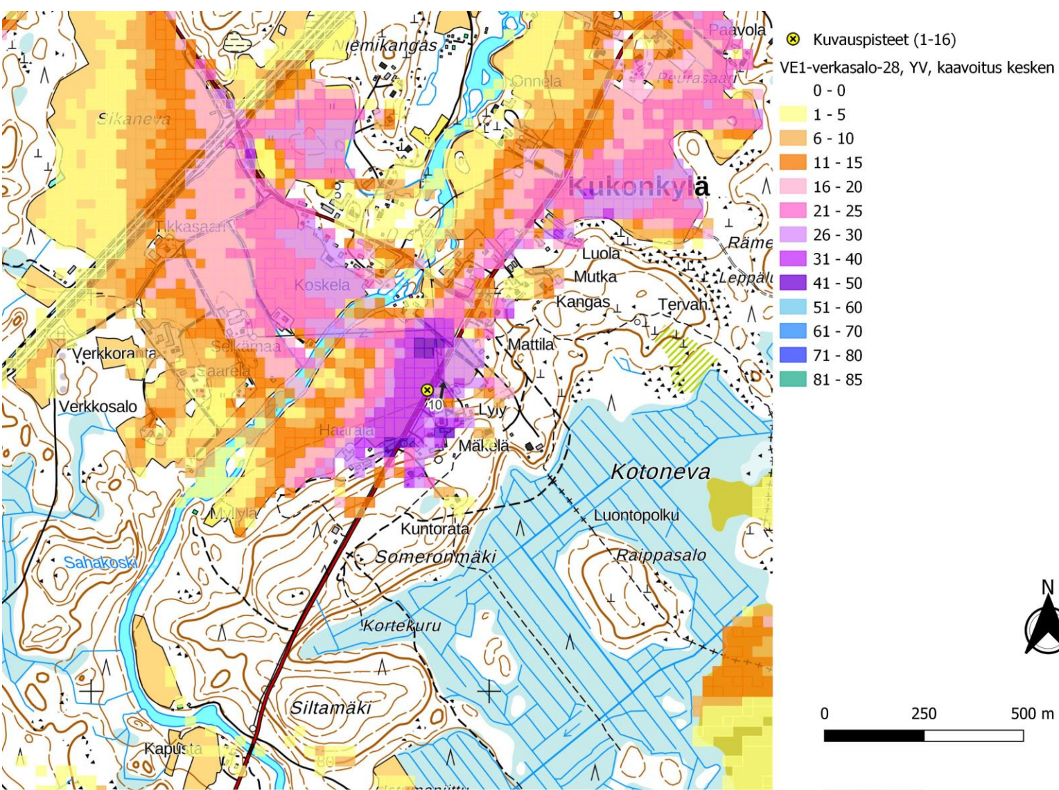
Kuva 78. Kuvauspiste 10. Verkasalon voimalat layout VE1 ja lähialueen hankkeet, joissa kaavoitus on kesken. Näkymäalueanalyysin laskentatulokset voimaloiden napakorkeudella mallinnettuna. (Oikea)
