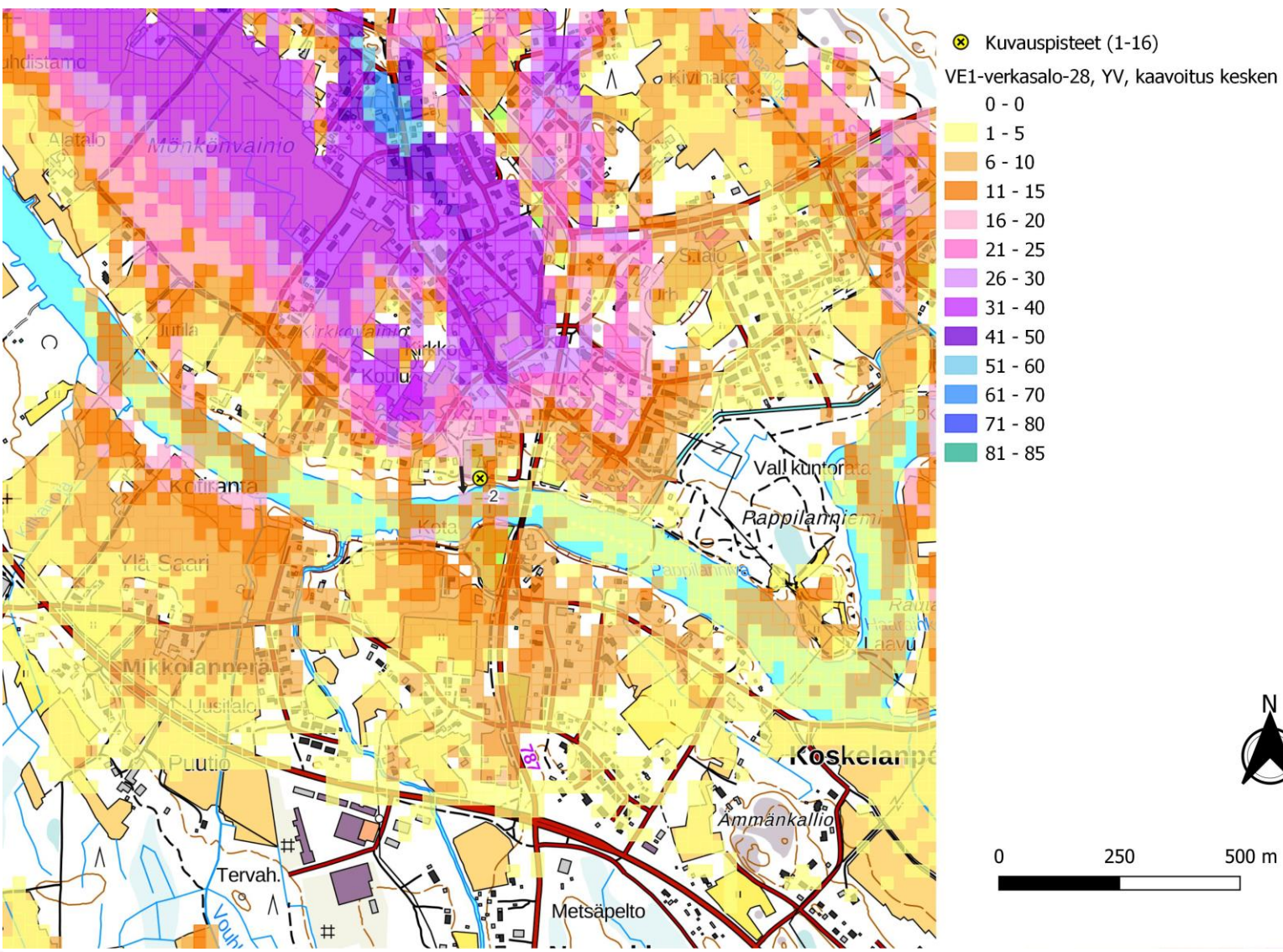
Kuva 14. Kuvauspiste 2. Verkasalon voimalat layout VE1 ja lähialueen hankkeet, joissa kaavoitus on kesken. Näkymäalueanalyysin laskentatulokset voimaloiden napakorkeudella mallinnettuna. (Oikea)
