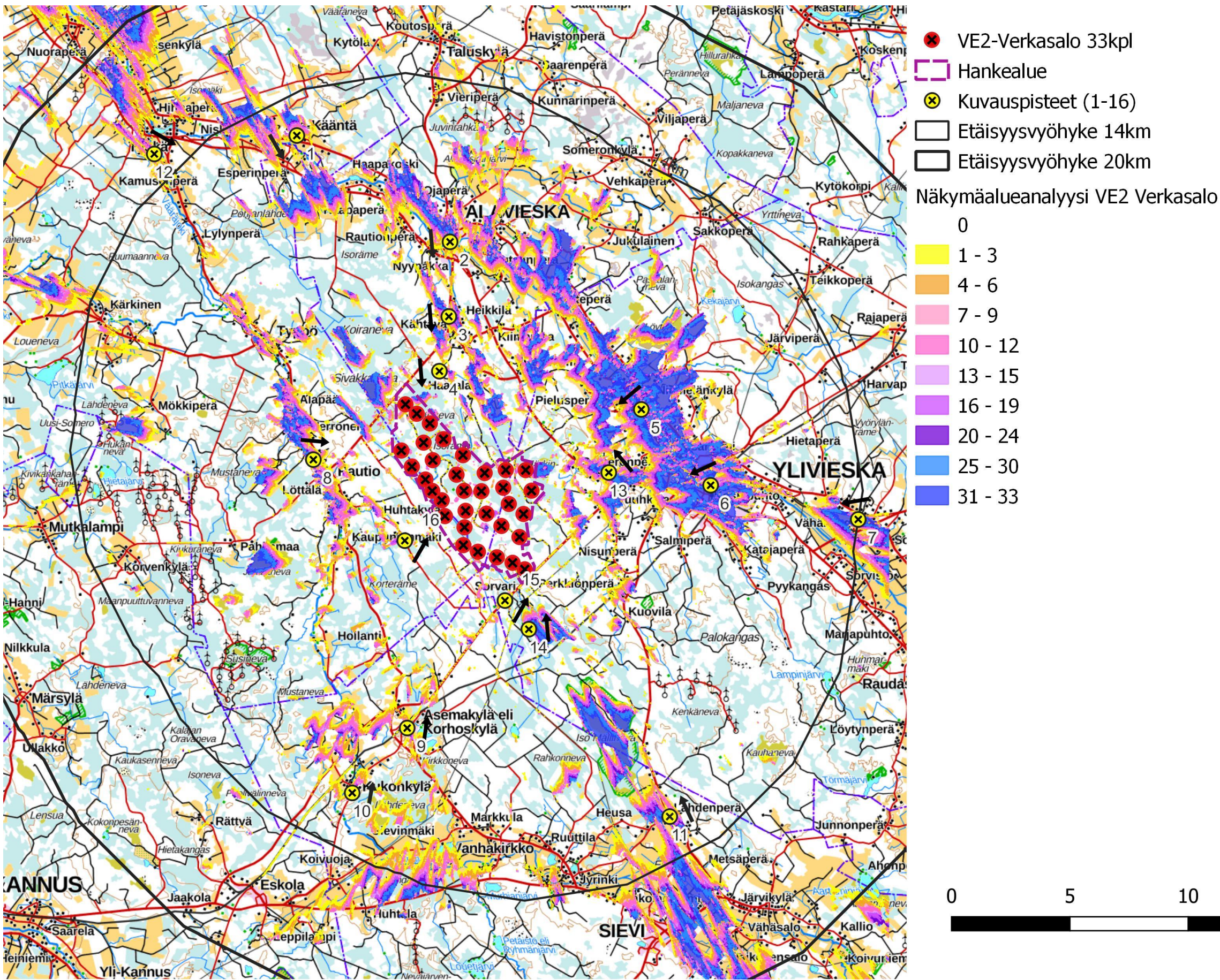
Kuva 3. Verkasalon layout VE2 näkymäalueanalyysin laskentatulokset voimaloiden napakorkeudella (220 metriä) mallinnettuna.
