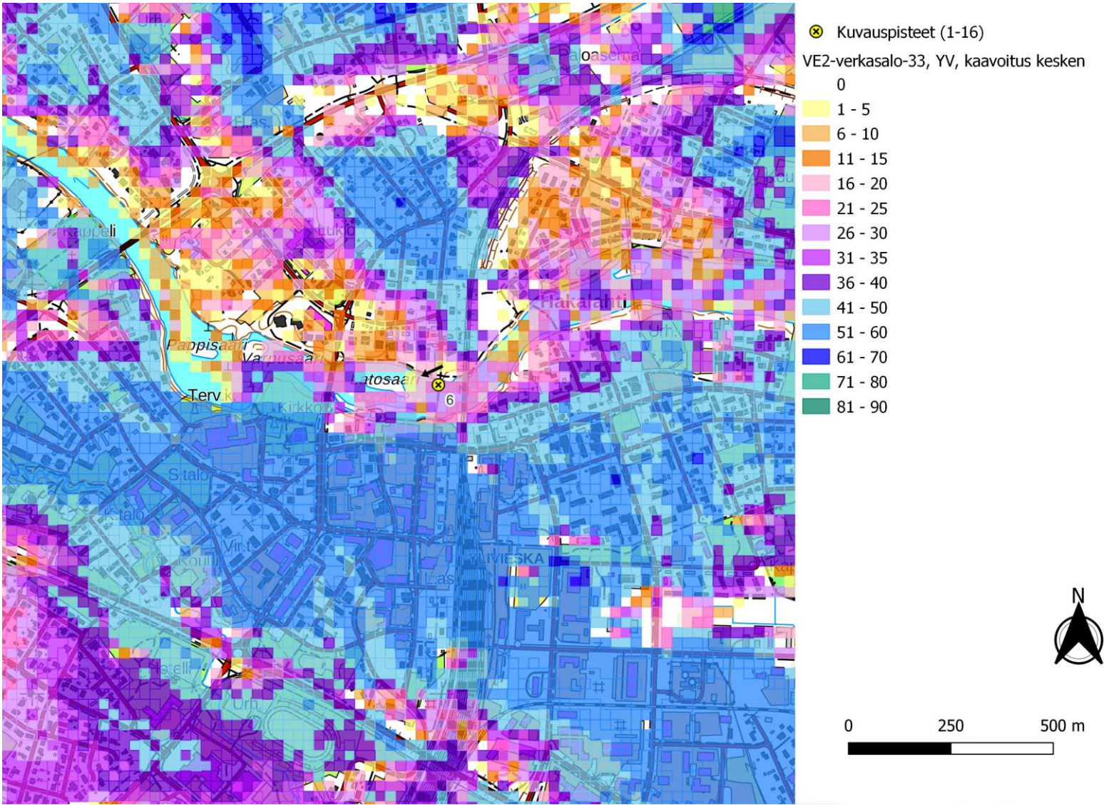
Kuva 50. Kuvauspiste 6. Verkasalon voimalat layout VE2 ja lähialueen hankkeet, joissa kaavoitus on kesken. Näkymäalueanalyysin laskentatulokset voimaloiden napakorkeudella mallinnettuna. (Oikea)
