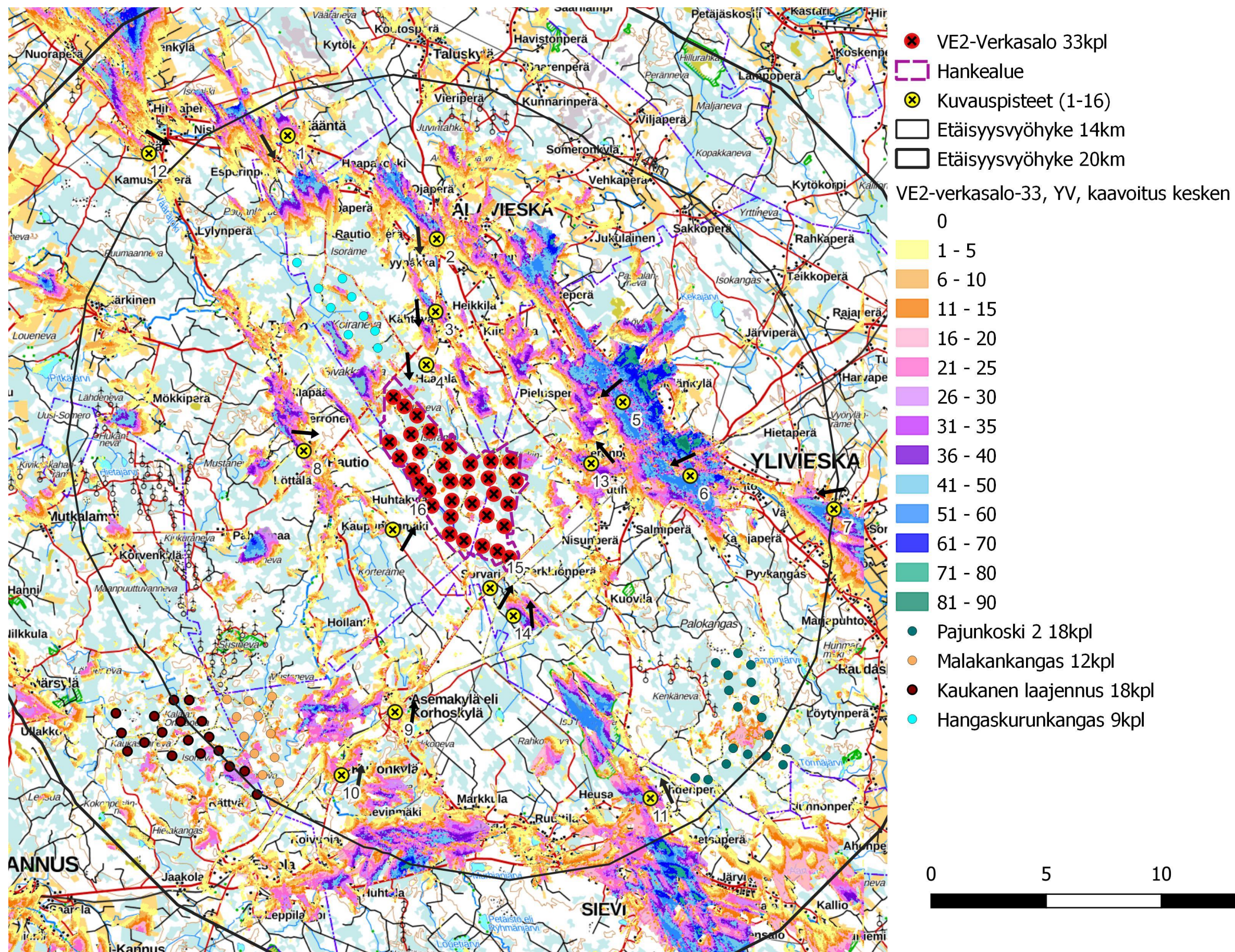
Kuva 4. Verkasalon layout VE2 ja lähialueen hankkeet, joissa kaavoitus on kesken. Näkymäalueanalyysin laskentatulokset voimaloiden napakorkeudella mallinnettuna.
