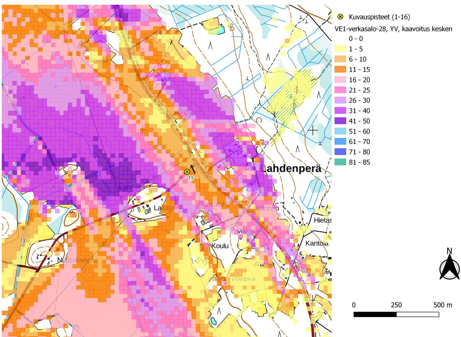
Kuva 86. Kuvauspiste 11. Verkasalon voimalat layout VE1 ja lähialueen hankkeet, joissa kaavoitus on kesken. Näkymäalueanalyysin laskentatulokset voimaloiden napakorkeudella mallinnettuna. (Oikea)
