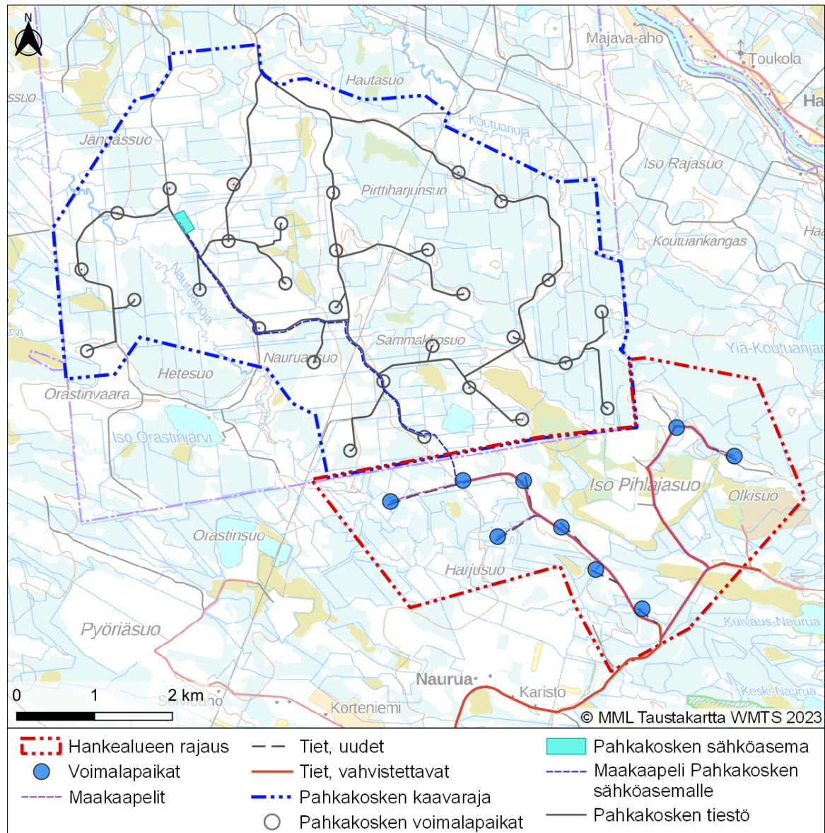
Kuva 2. Iso Pihlajasuon ja Pahkakosken voimalasijoittelu, Pahkakosken sähköasema ja alustava maakaapelireitti.
