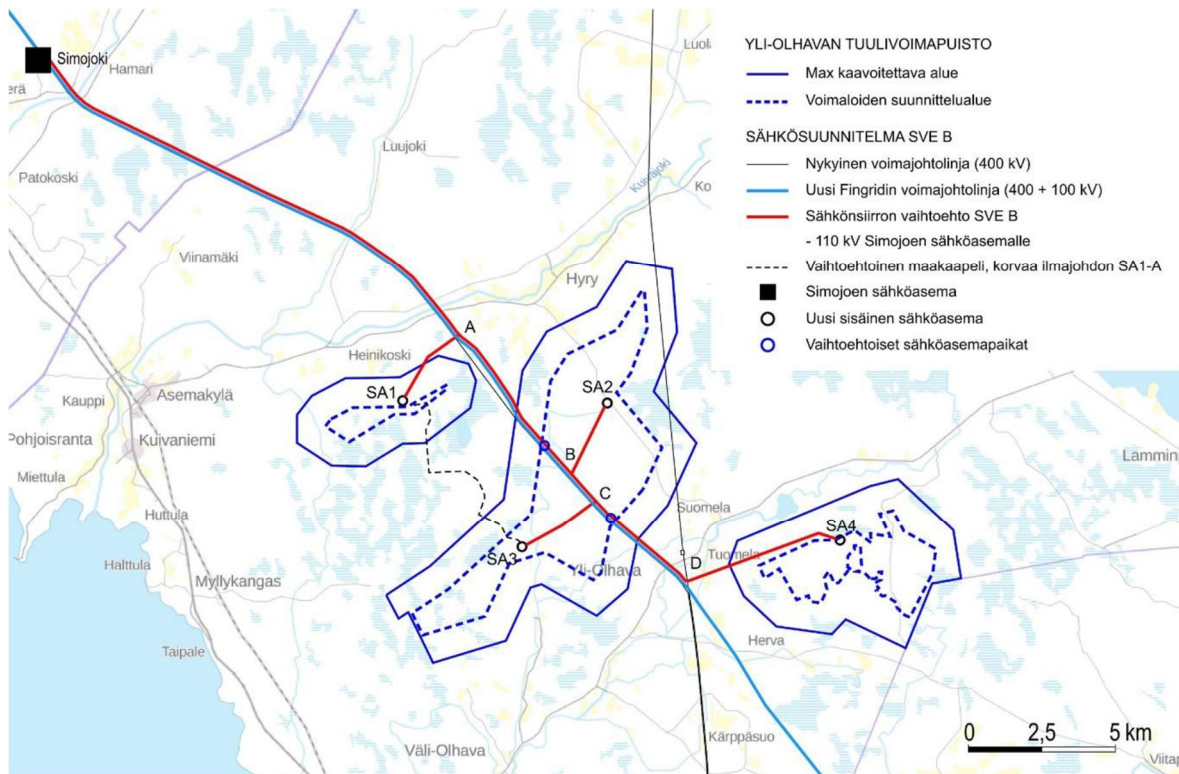
Kuva 25. Sähkönsiirron vaihtoehto (SVE B)
