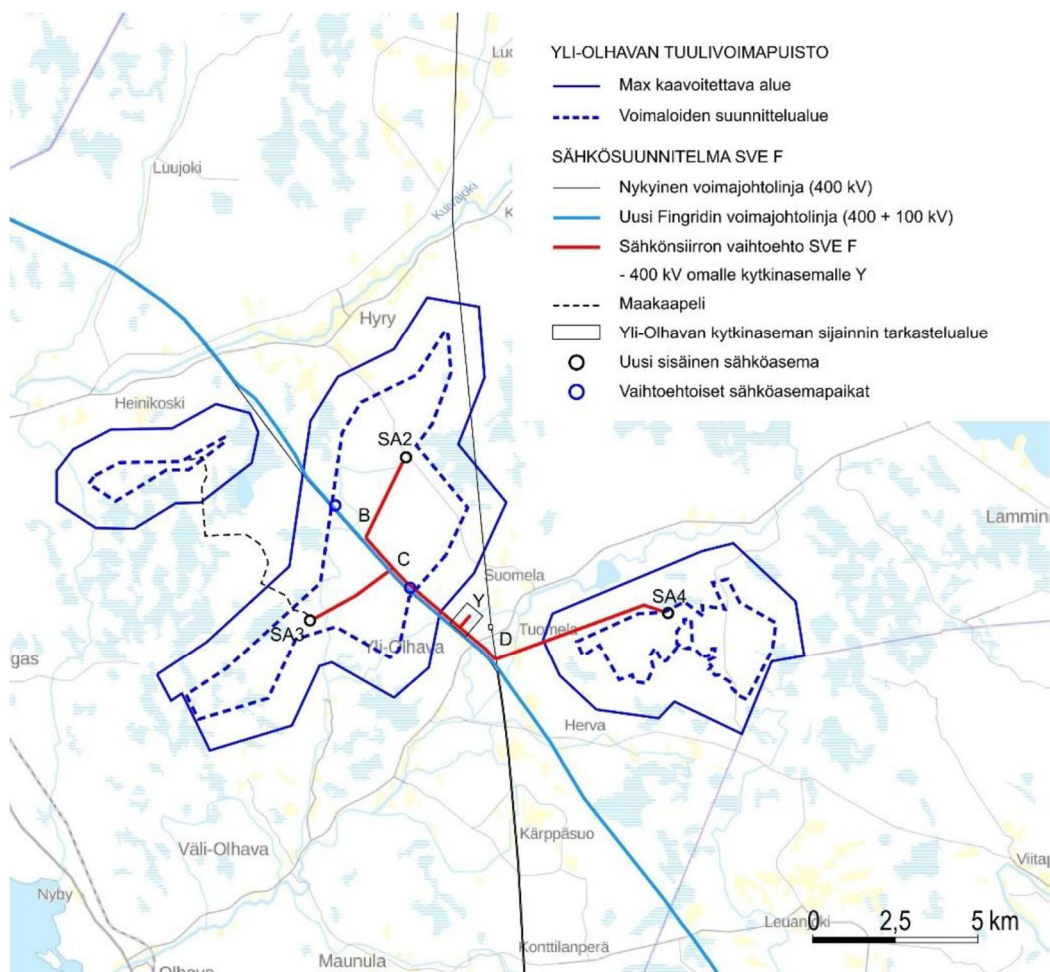
Kuva 27. Sähkönsiirron vaihtoehto (SVE F)
