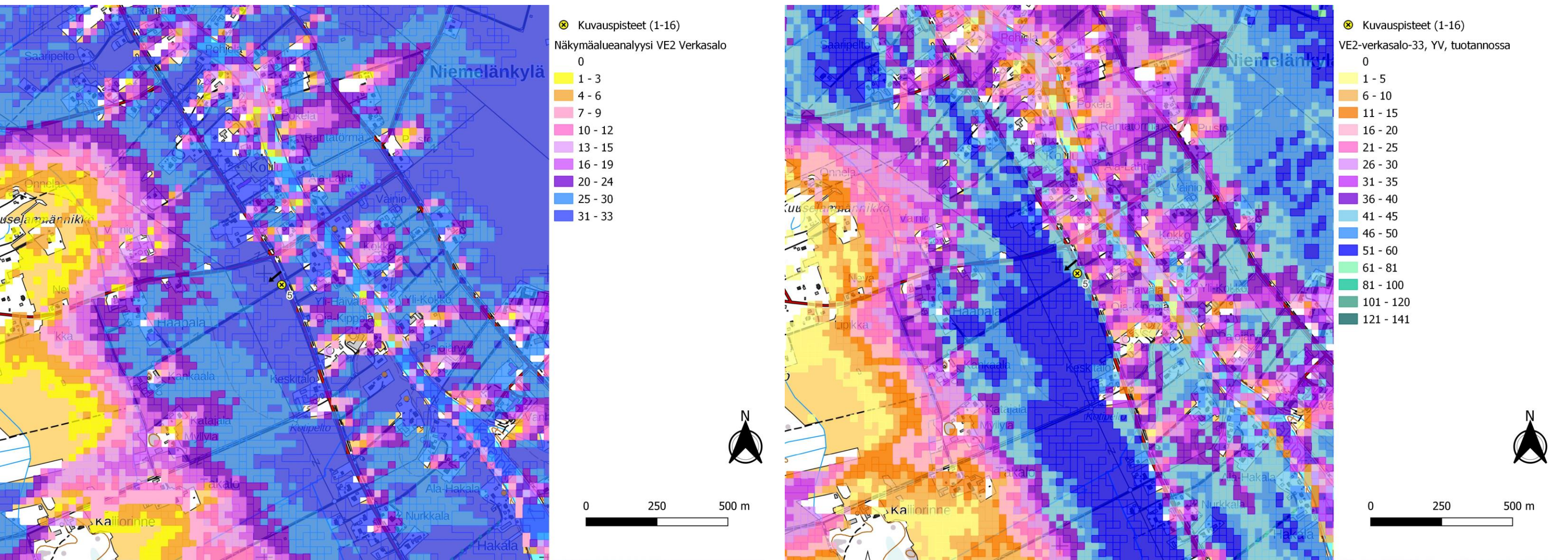
Kuva 41. Kuvauspiste 5. Verkasalon voimalat layout VE2. Näkymäalueanalyysin laskentatulokset voimaloiden napakorkeudella mallinnettuna. (Vasen)
