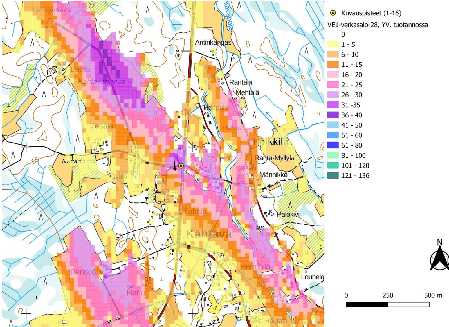
Kuva 22. Kuvaspiste 3. Verkasalon voimalat layout VE1 ja lähialueen toiminnassa olevat voimalat. Näkymäalueanalyysin laskentatulokset voimaloiden napakorkeudella mallinnettuna. (Oikea)
