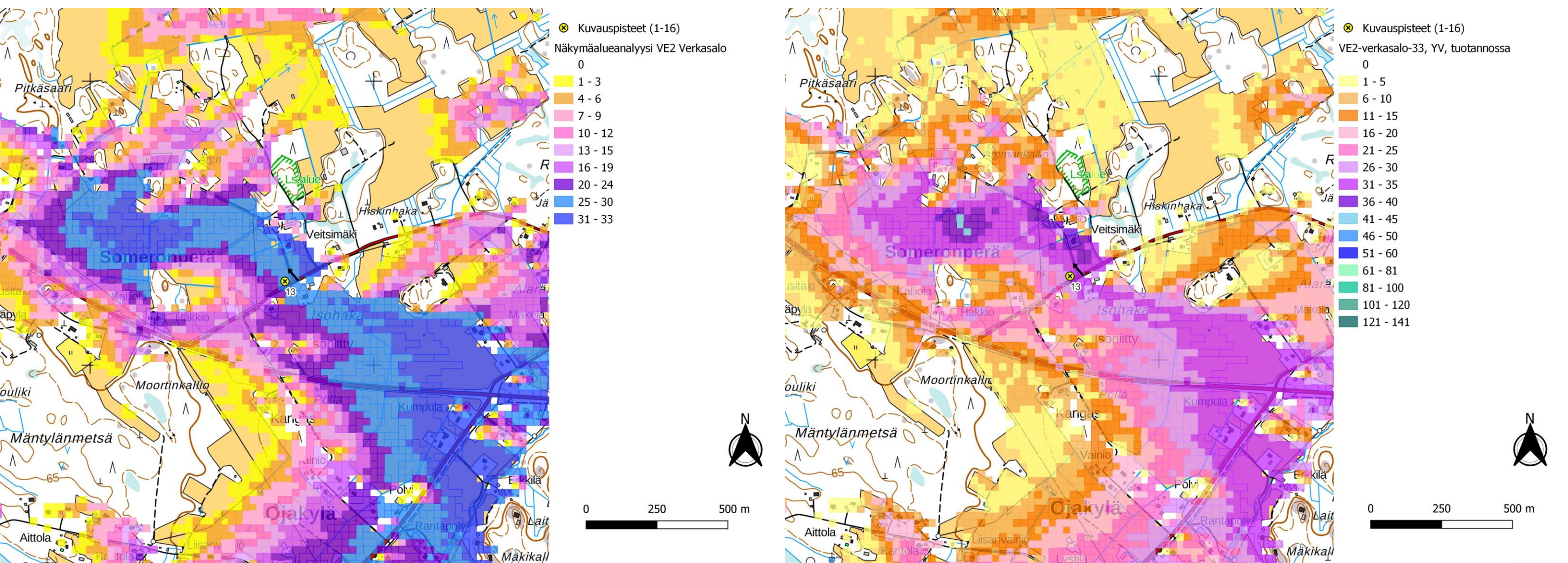
Kuva 104. Kuvauspiste 13. Verkasalon voimalat layout VE2. Näkymäalueanalyysin laskentatulokset voimaloiden napakorkeudella mallinnettuna. (Vasen)
