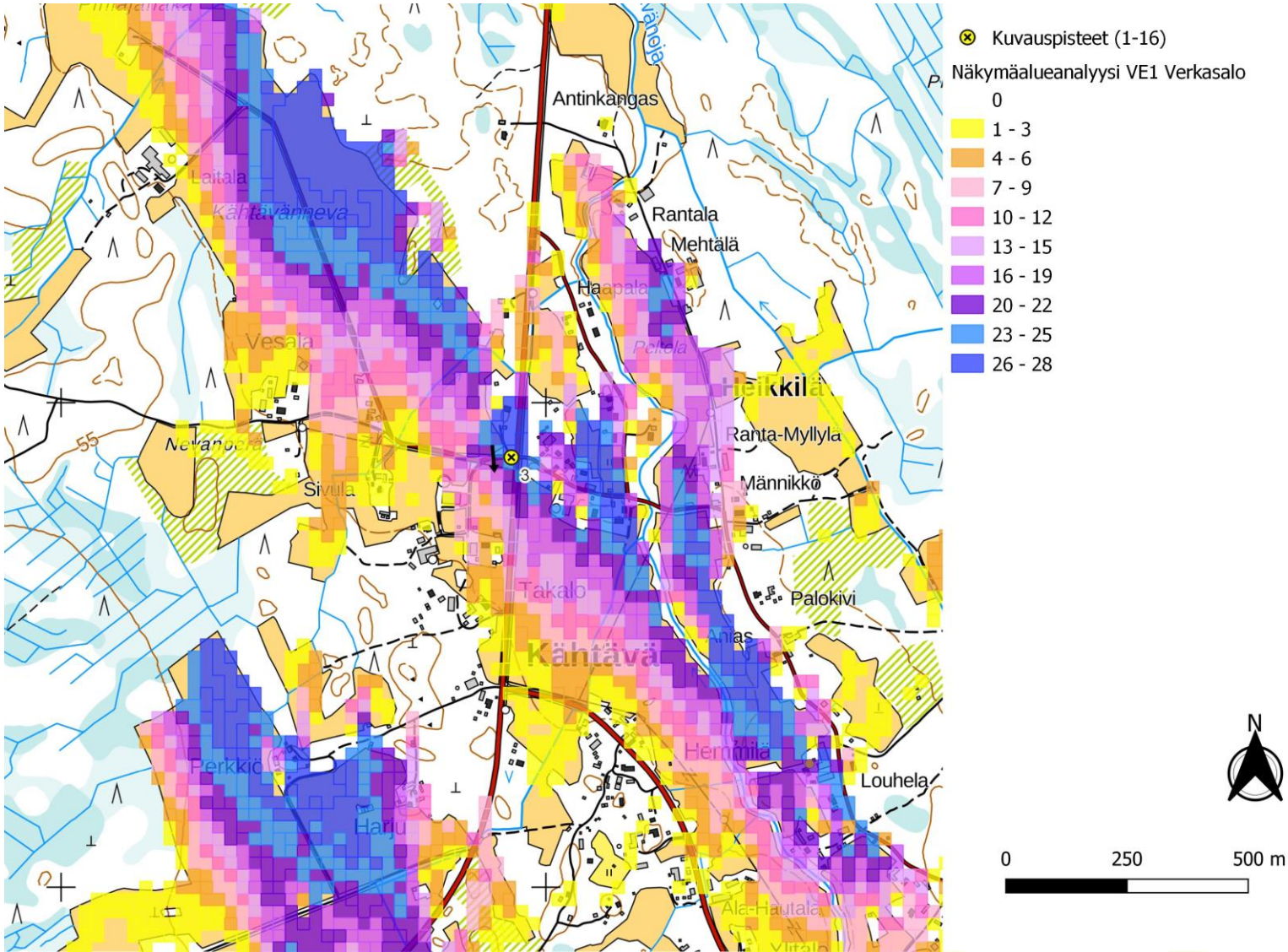
Kuva 21. Kuvaspiste 3. Verkasalon voimalat layout VE1. Näkymäalueanalyysin laskentatulokset voimaloiden napakorkeudella mallinnettuna. (Vasen)
