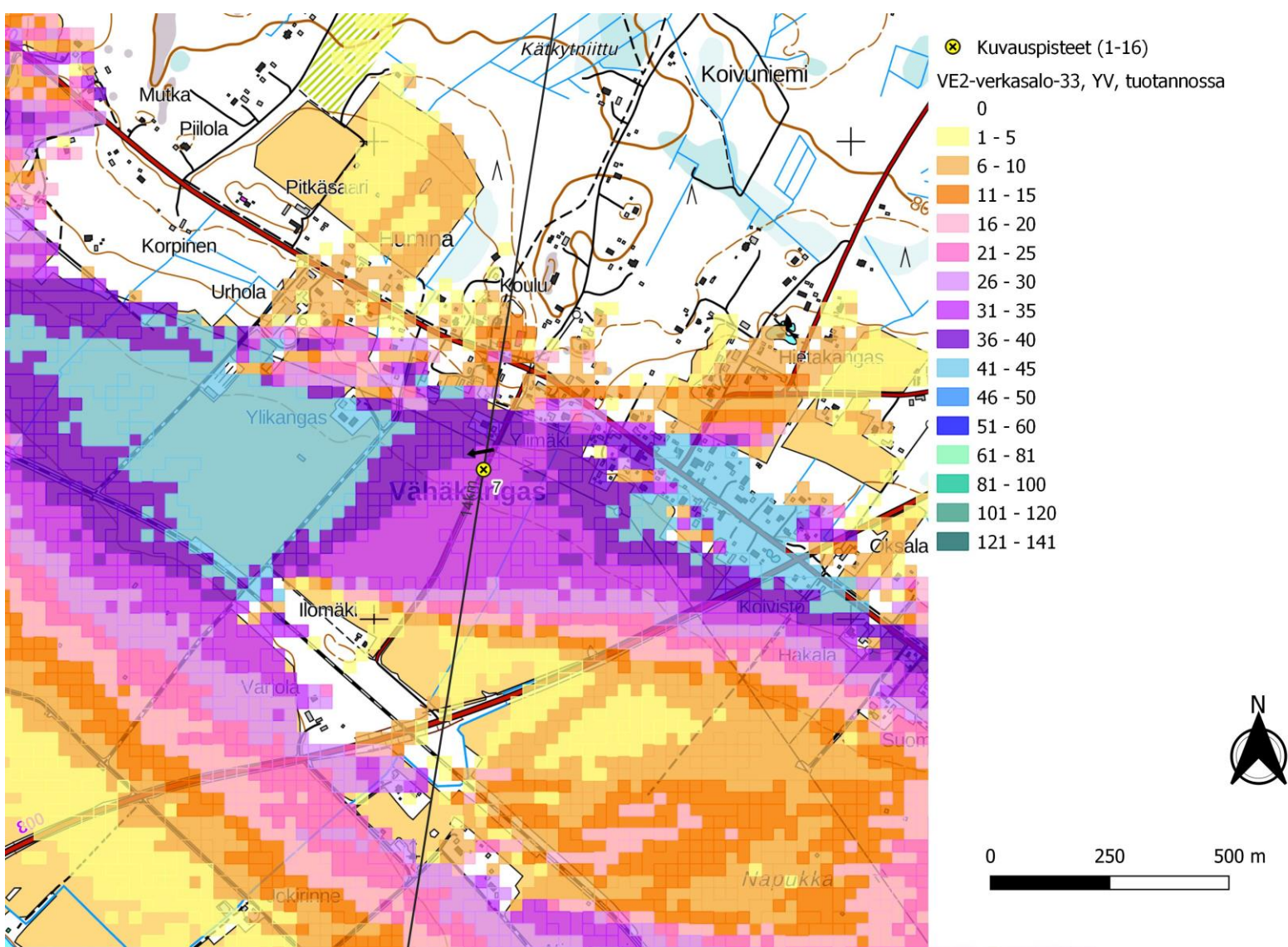
Kuva 58. Kuvauspiste 7. Verkasalon voimalat layout VE2 ja lähialueen toiminnassa olevat voimalat. Näkymäalueanalyysin laskentatulokset voimaloiden napakorkeudella mallinnettuna. (Oikea)
