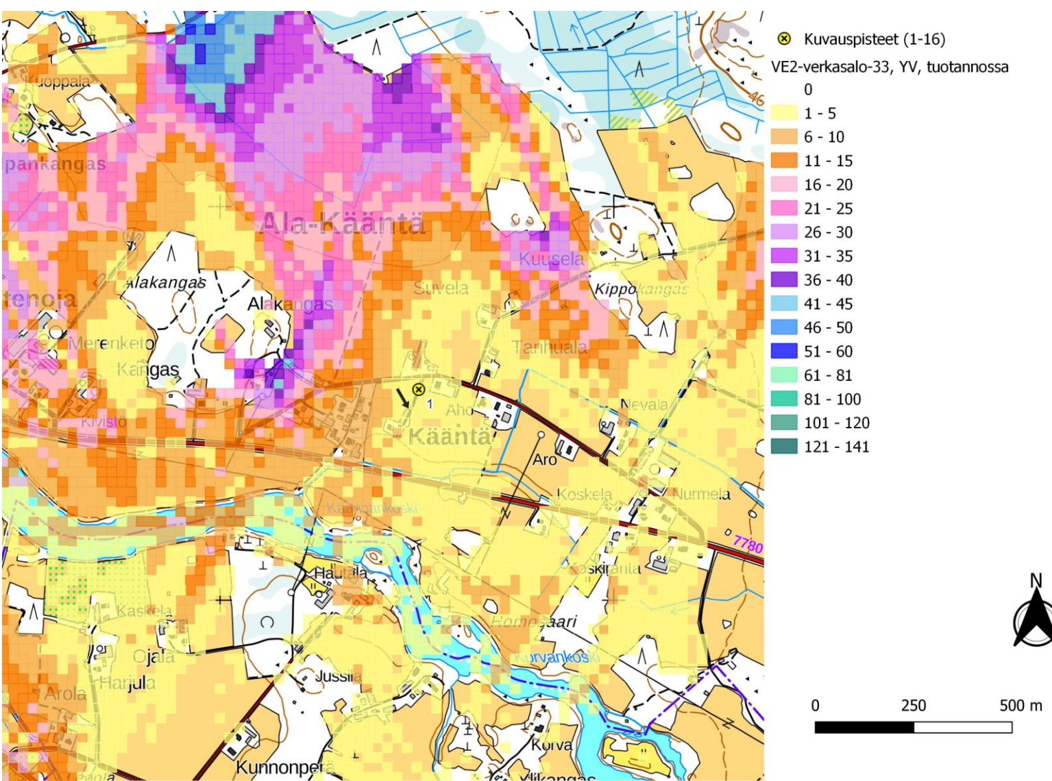
Kuva 10. Kuvauspiste 1. Verkasalon voimalat layout VE2 ja lähialueen toiminnassa olevat voimalat. Näkymäalueanalyysin laskentatulokset voimaloiden napakorkeudella mallinnettuna. (Oikea)
