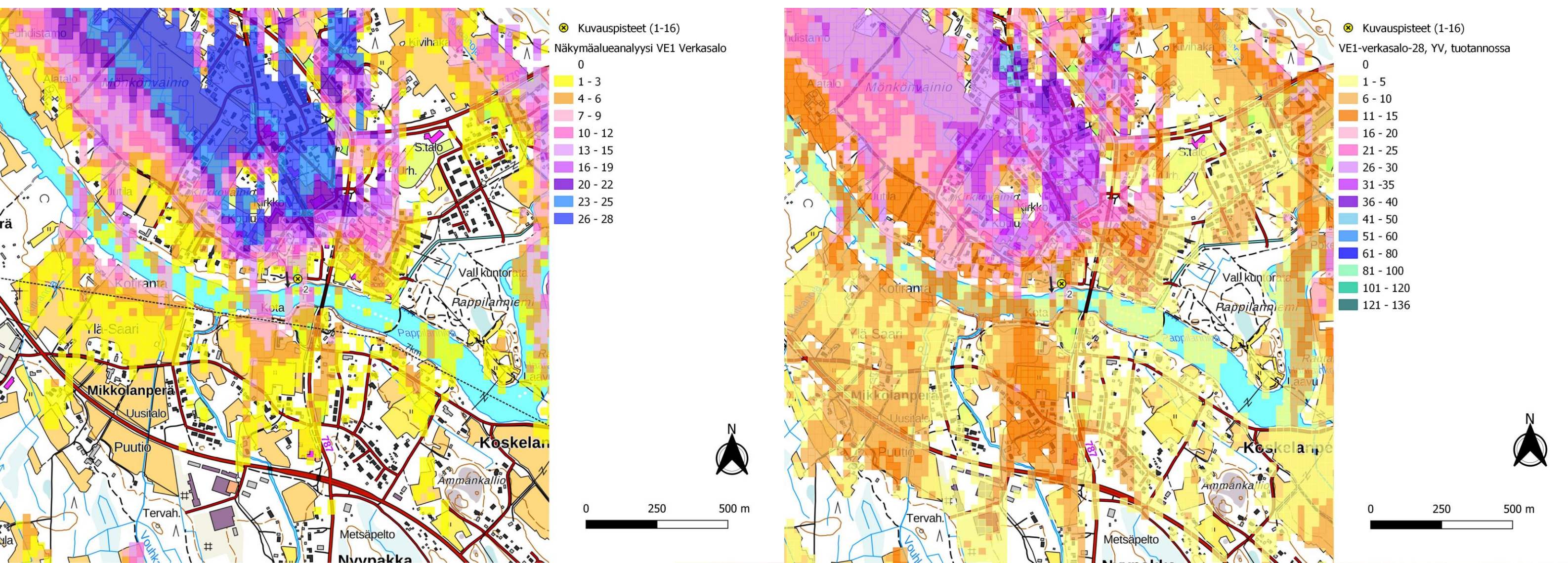
Kuva 13. Kuvauspiste 2. Verkasalon voimalat layout VE1. Näkymäalueanalyysin laskentatulokset voimaloiden napakorkeudella mallinnettuna. (Vasen)
