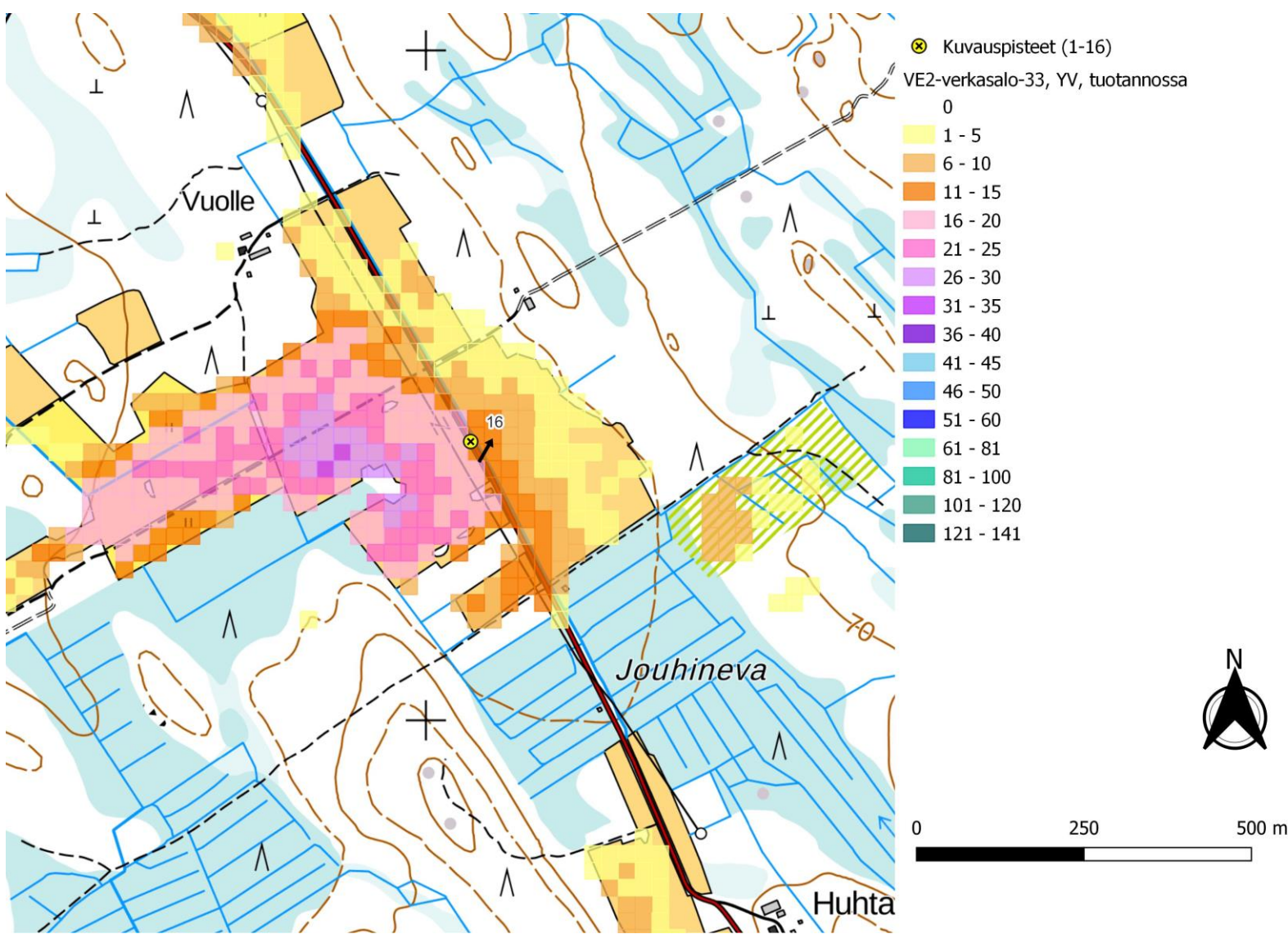
Kuva 129. Kuvauspiste 16. Verkasalon voimalat layout VE2 ja lähialueen toiminnassa olevat voimalat. Näkymäalueanalyysin laskentatulokset voimaloiden napakorkeudella mallinnettuna. (Oikea)
