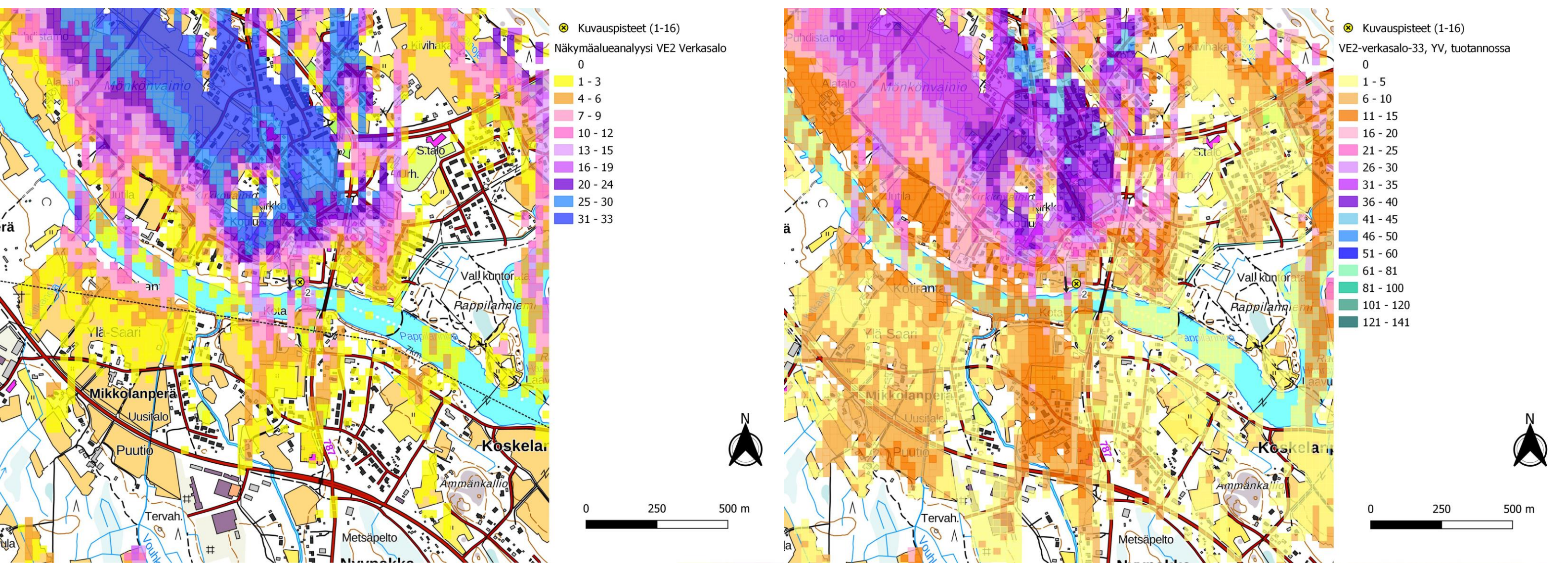
Kuva 17. Kuvauspiste 2. Verkasalon voimalat layout VE2. Näkymäalueanalyysin laskentatulokset voimaloiden napakorkeudella mallinnettuna. (Vasen)
