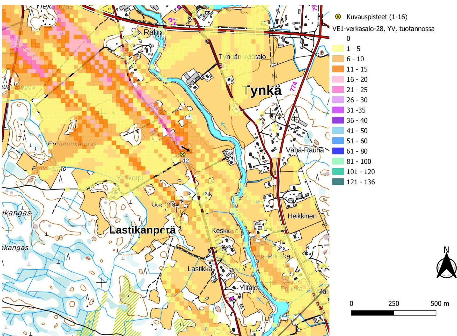
Kuva 93. Kuvauspiste 12. Verkasalon voimalat layout VE1 jaa lähialueen toiminnassa olevat voimalat. Näkymäalueanalyysin laskentatulokset voimaloiden napakorkeudella mallinnettuna. (Oikea)
