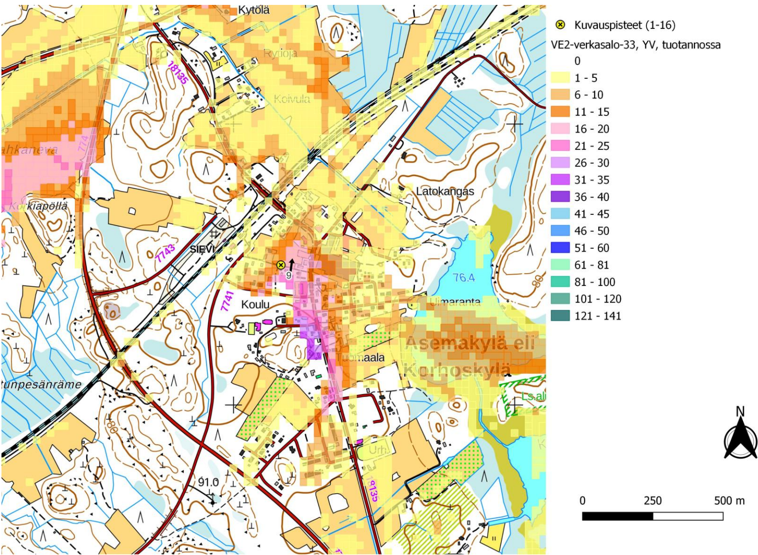
Kuva 74. Kuvauspiste 9. Verkasalon voimalat layout VE2 ja lähialueen toiminnassa olevat voimalat. Näkymäalueanalyysin laskentatulokset voimaloiden napakorkeudella mallinnettuna. (Oikea)
