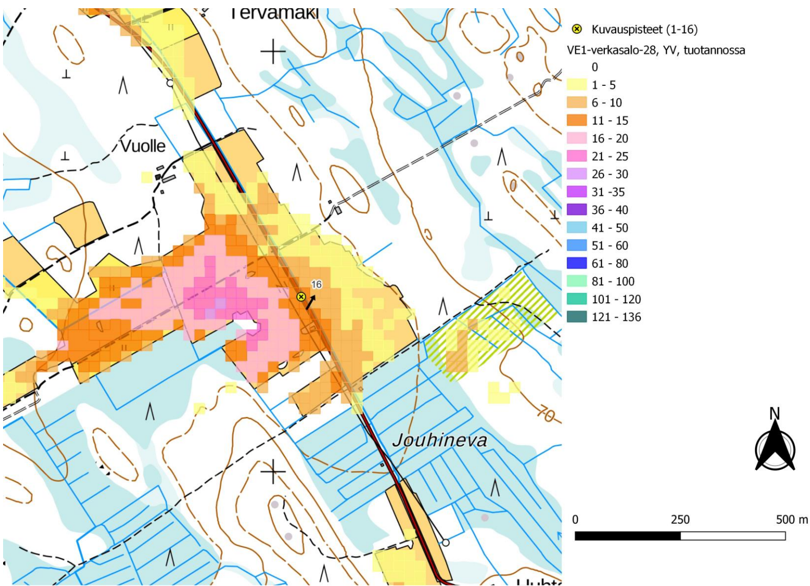
Kuva 125. Kuvauspiste 16. Verkasalon voimalat layout VE1 ja lähialueen toiminnassa olevat voimalat. Näkymäalueanalyysin laskentatulokset voimaloiden napakorkeudella mallinnettuna. (Oikea)
