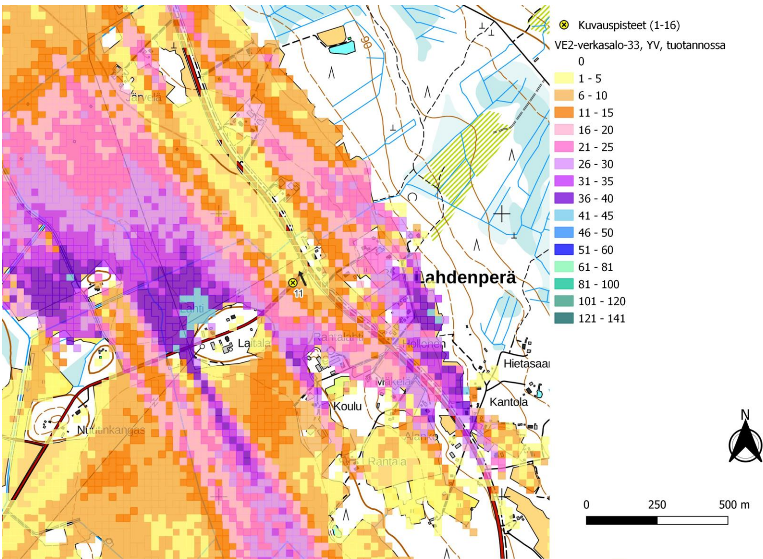
Kuva 89. Kuvauspiste 11. Verkasalon voimalat layout VE2 jaa lähialueen toiminnassa olevat voimalat. Näkymäalueanalyysin laskentatulokset voimaloiden napakorkeudella mallinnettuna. (Oikea)
