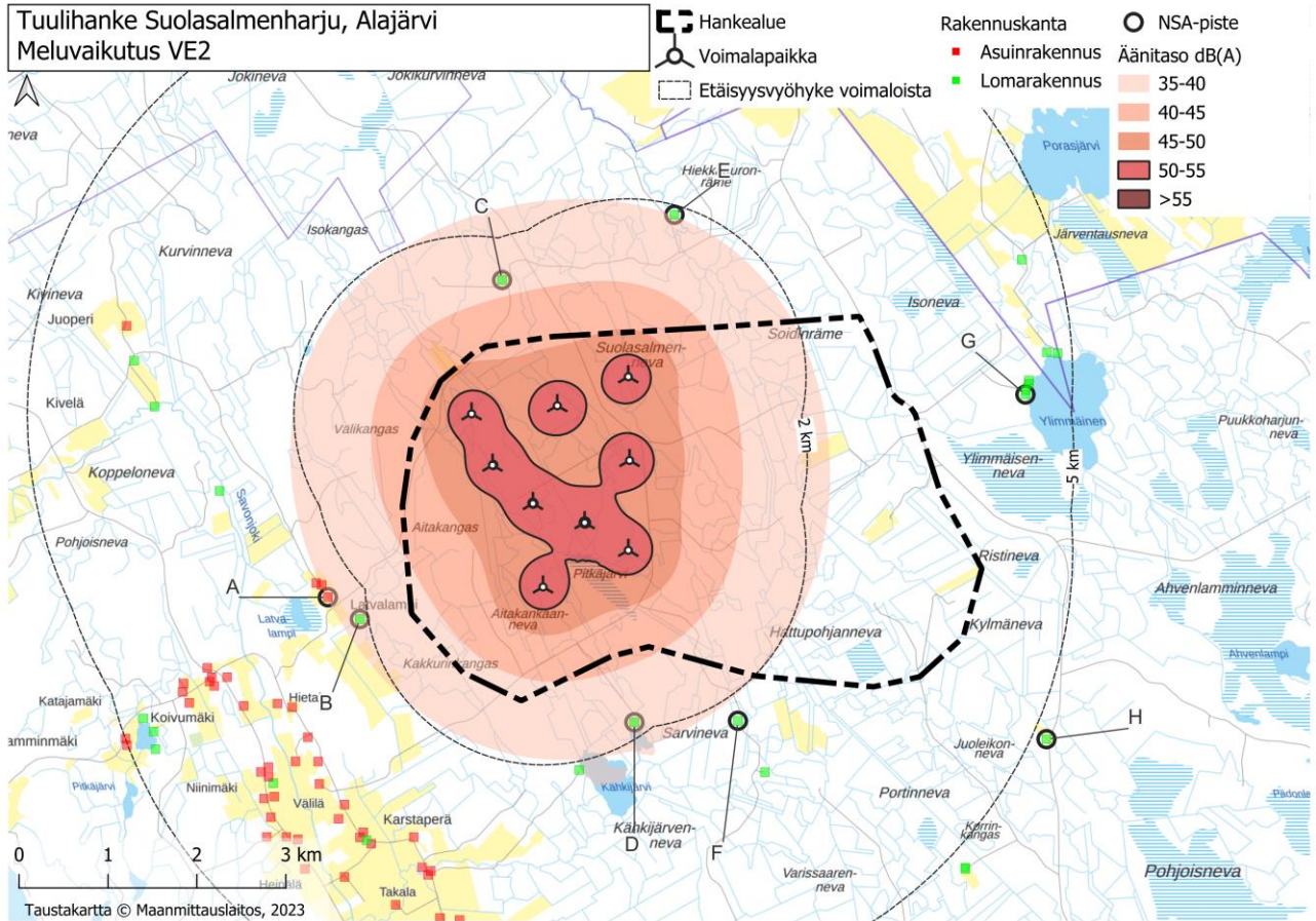
Kuva 5. VE2-layoutin melumallinnuksen mukainen meluvyöhykekartta.
