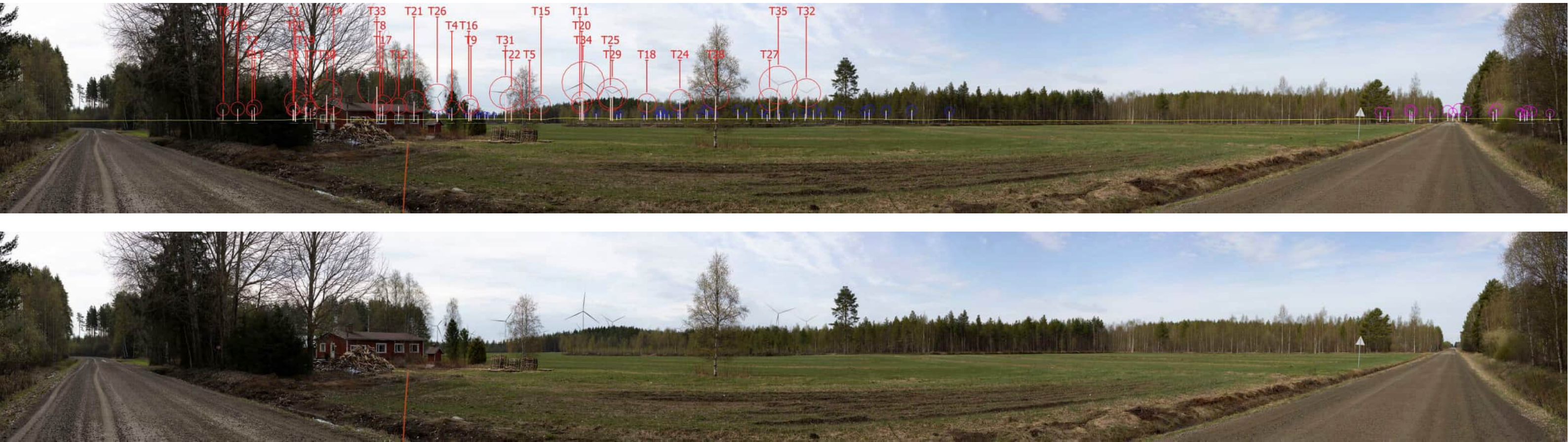
Kuva 231 ja 232. Valokuvasovite kuvauspisteessä 20, layout VE1. Kuva on otettu Kajaanin Kallionperästä Kestiläntieltä, kuvaussuunta luoteeseen. Etäisyys voimaloihin on noin 2,8 kilometriä. Yläkuva draft ja alakuva varsinainen valokuvasovite. Löytösuon voimalat numeroitu ja korostettu punaisella. Toiminnassa olevat hankkeet korostettu Piiparinmäen voimalat sinisellä, Metsäamminkankaan voimalat pinkillä.
