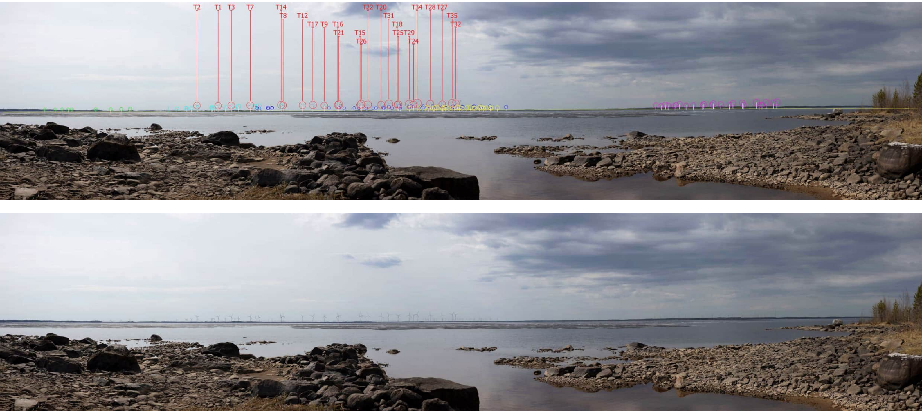
Kuva 261 ja 262. Valokuvasovite kuvauspisteessä 22, layout VE2. Kuva on otettu Vaalan Mustaniemestä, kuvaussuunta luoteeseen. Etäisyys voimaloihin on noin 12,1 kilometriä. Yläkuva draft ja alakuva varsinainen valokuvasovite. Löytösuon voimalat numeroitu ja korostettu punaisella. Toiminnassa olevat hankkeet korostettu Piiparinmäen voimalat sinisellä, Metsälamminkankaan voimalat pinkillä. Yhteisvaikutushankkeet korostettu kuvissa Kokkosuon voimalat turkoosilla, Pyöriännevan voimalat keltaisella, Luolakankaan voimalat vihreällä.
