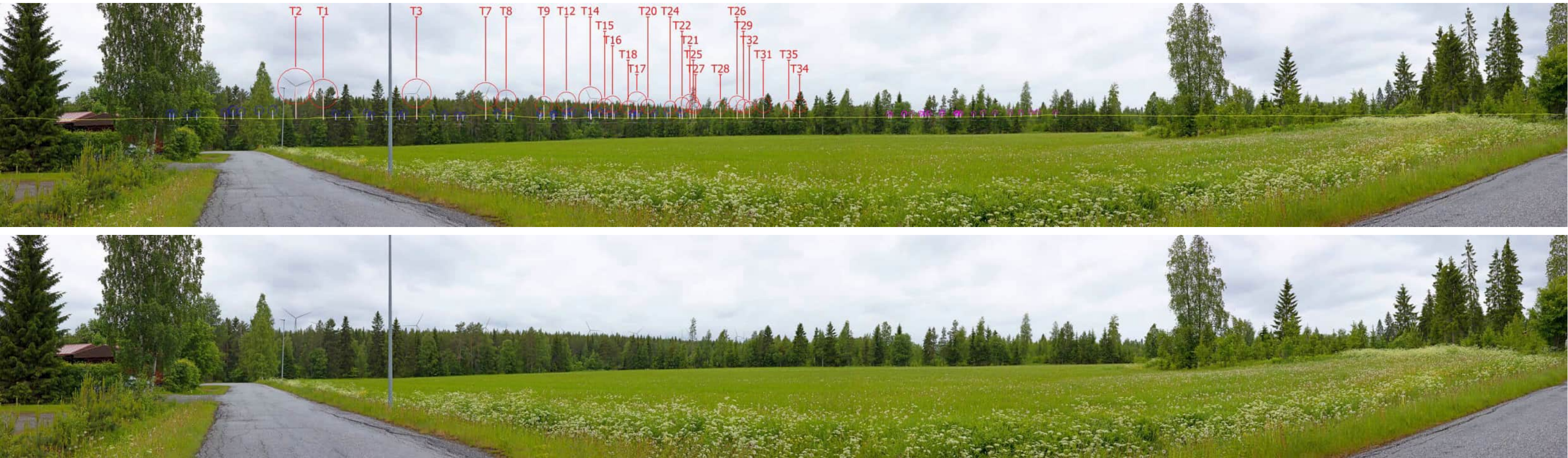
Kuva 127 ja 128. Valokuviasovite kuvauspisteessä 10, layout VE2. Kuva on otettu Kajaanin Vuolijoelta Vuolijoentieltä, kuvaussuunta länsi-luoteeseen. Etäisyys voimaloihin on noin 3,4 kilometriä. Yläkuva draft ja alakuva varsinainen valokuviasovite. Löytösuon voimalat numeroitu ja korostettu punaisella. Toiminnassa olevat hankkeet korostettu Piiparinmäen voimalat sinisellä, Metsälamminkankaan voimalat pinkillä.
