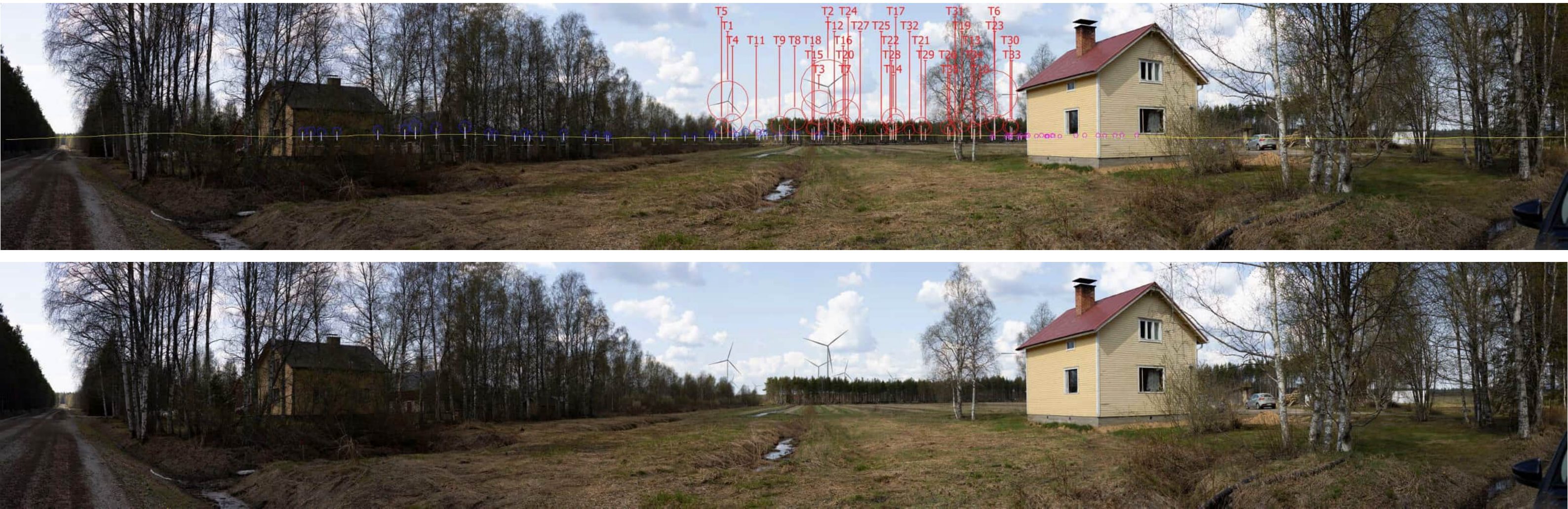
Kuva 183 ja 184. Valokuvasevite kuvauspisteessä 16, layout VE1. Kuva on otettu Kajaanin Vuolijoen Keisarintieltä, kuvaussuunta länsi-luoteeseen. Etäisyys voimaloihin on noin 2,1 kilometriä. Yläkuva draft ja alakuva varsinainen valokuvasevite. Löytösuon voimalat numeroitu ja korostettu punaisella. Toiminnassa olevat hankkeet korostettu Piiparinmäen voimalat sinisellä, Metsäamminkankaan voimalat pinkillä.
