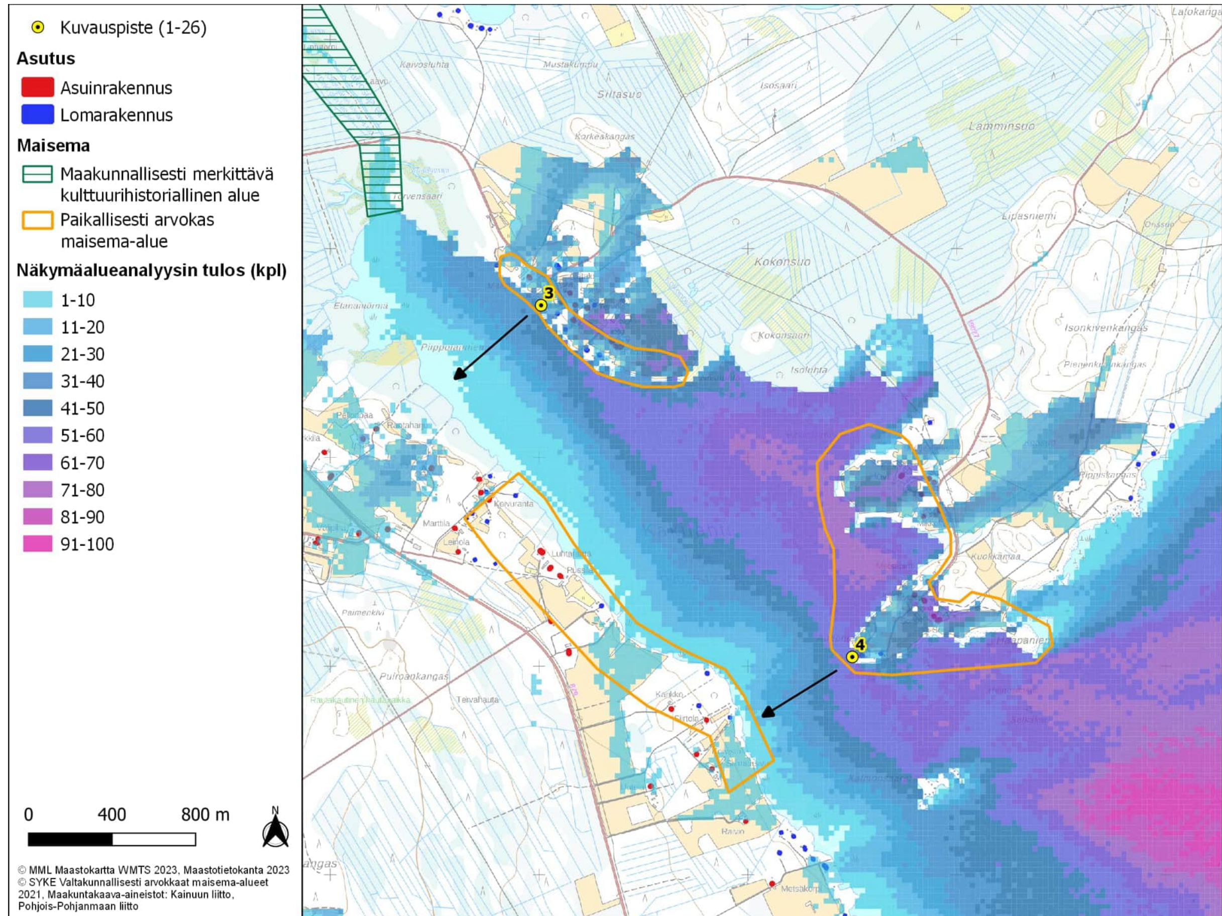
Kuva 46. Kuvauspiste 4, kuva otettu Kajaanin Kärkisaaresta. Löytösuon layout versio 1 (VE1) näkymäalueanalyysin laskentatulokset voimaloiden napakorkeudella mallinnettuna.
