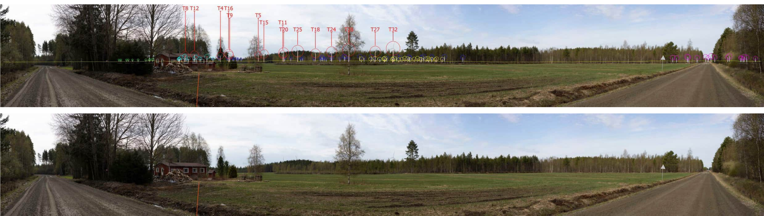
Kuva 241 ja 242. Valokuvasovite kuvauspisteessä 20, layout VE3. Kuva on otettu Kajaanin Kallionperästä Kestiläntieltä, kuvaussuunta luoteeseen. Etäisyys voimaloihin on noin 3,7 kilometriä. Yläkuva draft ja alakuva varsinainen valokuvasovite. Löytösuon voimalat numeroitu ja korostettu punaisella. Toiminnassa olevat hankkeet korostettu Piiparinmäen voimalat sinisellä, Metsälamminkankaan voimalat pinkillä. Yhteisvaikutushankkeet korostettu kuvissa Kokkosuon voimalat turkoosilla, Pyöriännevan voimalat keltaisella, Luolakankaan voimalat vihreällä.
