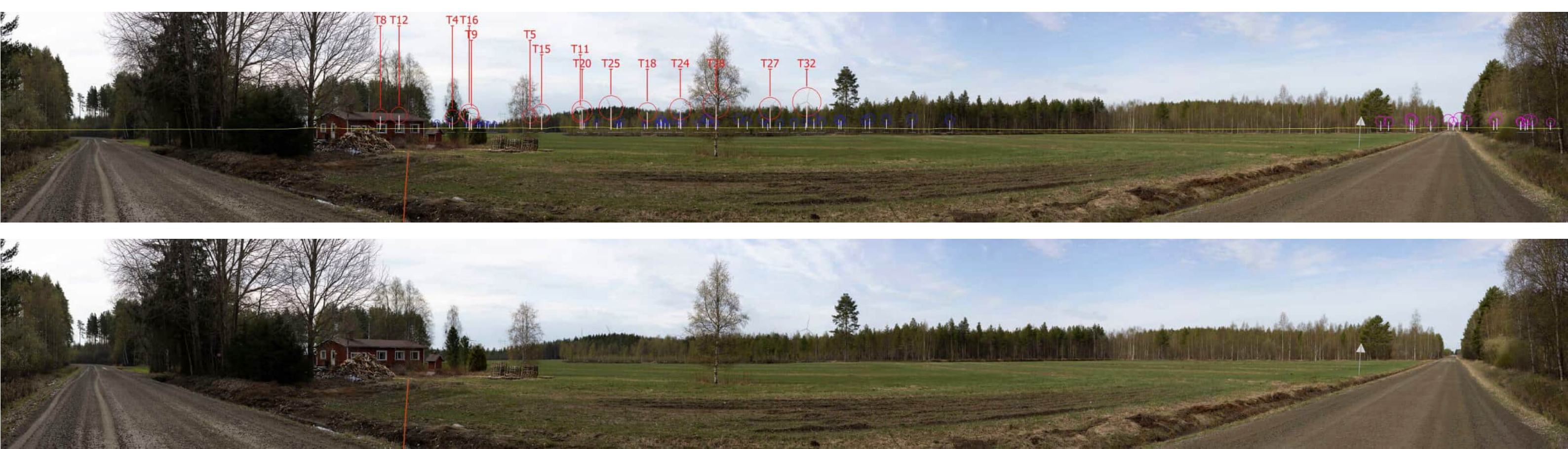
Kuva 239 ja 240. Valokuvasovite kuvauspisteessä 20, layout VE3. Kuva on otettu Kajaanin Kallionperästä Kestiläntieltä, kuvaussuunta luoteeseen. Etäisyys voimaloihin on noin 3,7 kilometriä. Yläkuva draft ja alakuva varsinainen valokuvasovite. Löytösuon voimalat numeroitu ja korostettu punaisella. Toiminnassa olevat hankkeet korostettu Piiparinmäen voimalat sinisellä, Metsälamminkankaan voimalat pinkillä.
