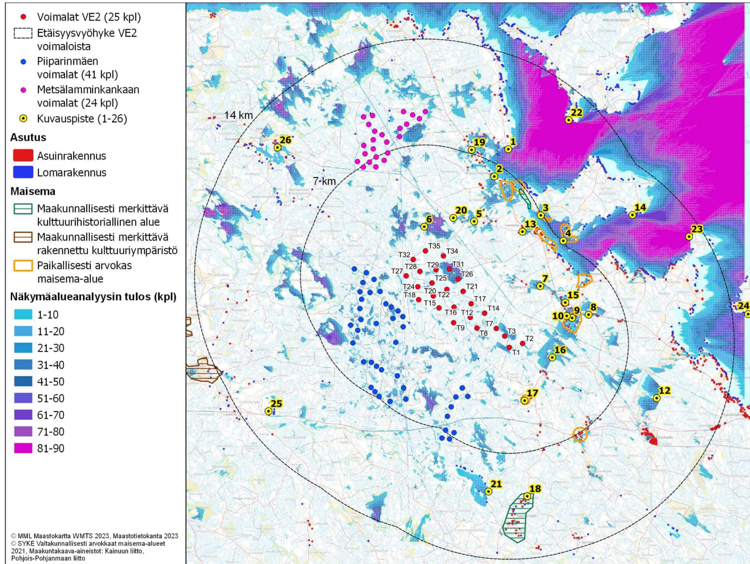
Kuva 3. Lötösuon layout versio 2 (VE2) näkymäalueanalyysin laskentatulokset voimaloiden napakorkeudella mallinnettuna. Lötösuon voimalat numeroitu ja korostettu punaisella. Toiminnassa olevat hankkeet korostettu väreillä, Piiparinmäen voimalat sinisellä, Metsälamminkankaan voimalat pinkillä.
