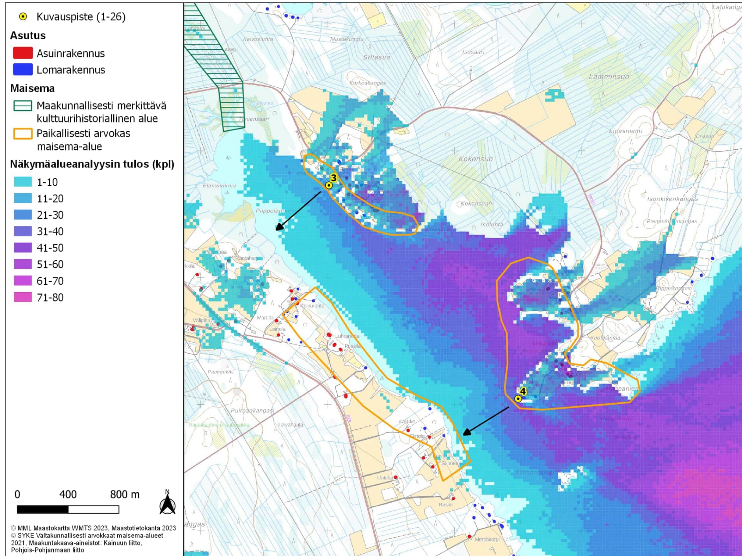
Kuva 56. Kuvauspiste 4, kuva otettu Kajaanin Kärkisaaresta. Löytösuo layout versio 3 (VE3) näkymäalueanalyysin laskentatulokset voimaloiden napakorkeudella mallinnettuna.
