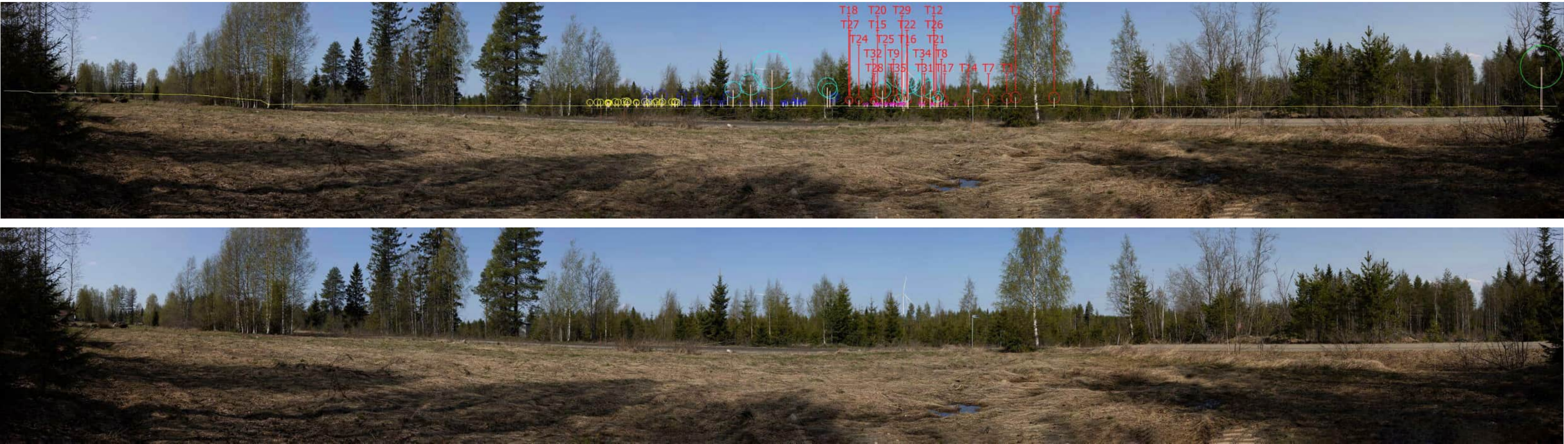
Kuva 213 ja 214. Valokuvasovite kuvauspisteessä 18, layout VE2. Kuva on otettu Kajaanin Saaresmäestä, kuvaussuunta luoteeseen. Etäisyys voimaloihin on noin 9,9 kilometriä. Yläkuva draft ja alakuva varsinainen valokuvasovite. Löytösuon voimalat numeroitu ja korostettu punaisella. Toiminnassa olevat hankkeet korostettu Piiparinmäen voimalat sinisellä, Metsäamminkankaan voimalat pinkillä. Yhteisvaikutushankkeet korostettu kuvissa Kokkosuon voimalat turkoosilla, Pyöriännevan voimalat keltaisella, Luolakankaan voimalat vihreällä.
