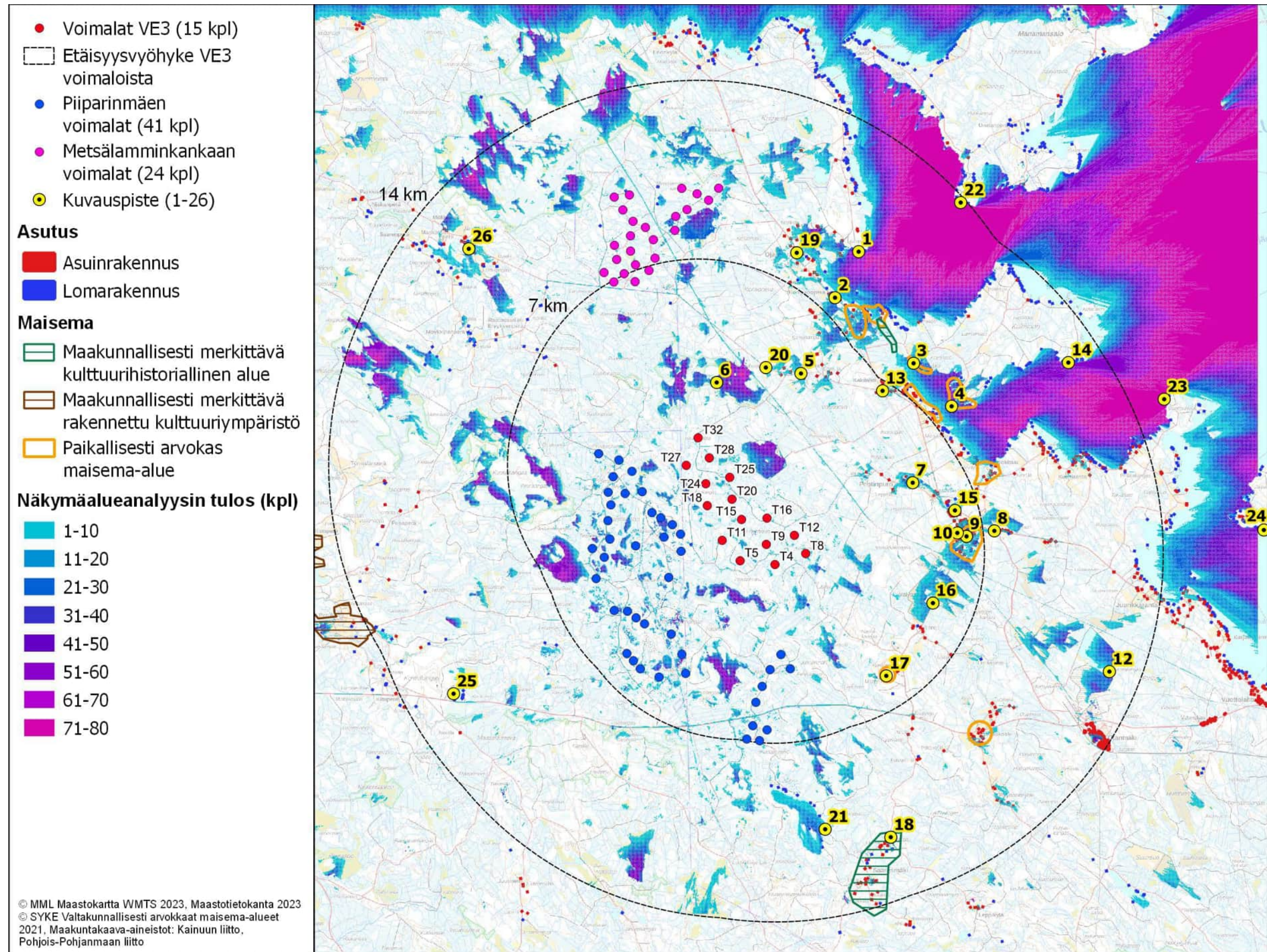
Kuva 5. Löytösuon layout versio 3 (VE3) näkymäalueanalyysin laskentatulokset voimaloiden napakorkeudella mallinnettuna. Löytösuon voimalat numeroitu ja korostettu punaisella. Toiminnassa olevat hankkeet korostettu väreillä, Piiparinmäen voimalat sinisellä, Metsäamminkankaan voimalat pinkillä.
