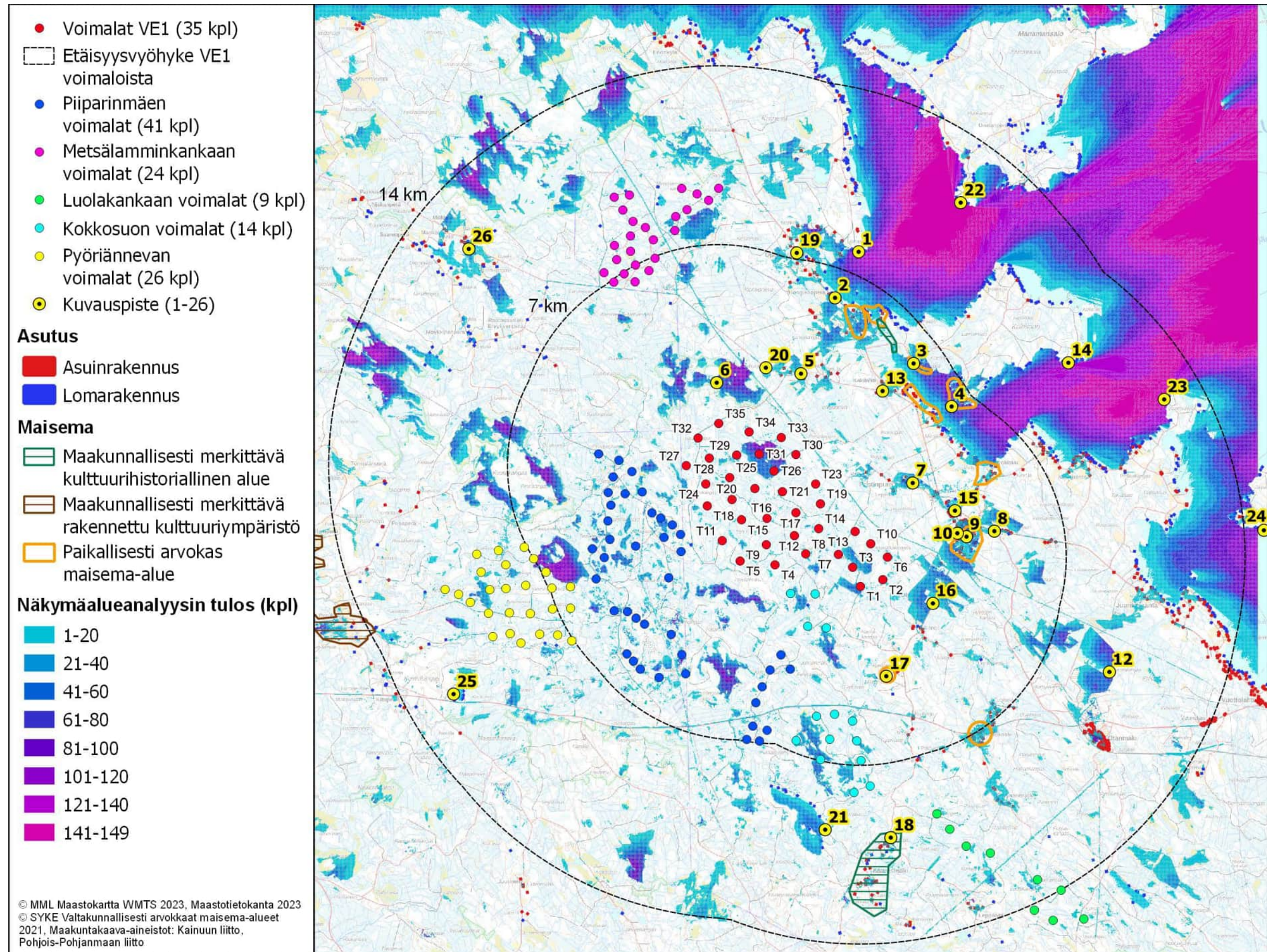
Kuva 2. Löytösuon layout versio 1 (VE1) näkymäalueanalyysin laskentatulokset voimaloiden napakorkeudella mallinnettuna. Löytösuon voimalat numeroitu ja korostettu punaisella. Toiminnassa olevat hankkeet korostettu väreillä, Piiparinmäen voimalat sinisellä, Metsäamminkankaan voimalat pinkillä. Yhteisvaikutushankkeet korostettu kuvissa Kokkosuon voimalat turkoosilla, Pyöriännevan voimalat keltaisella, Luolakankaan voimalat vihreällä.
