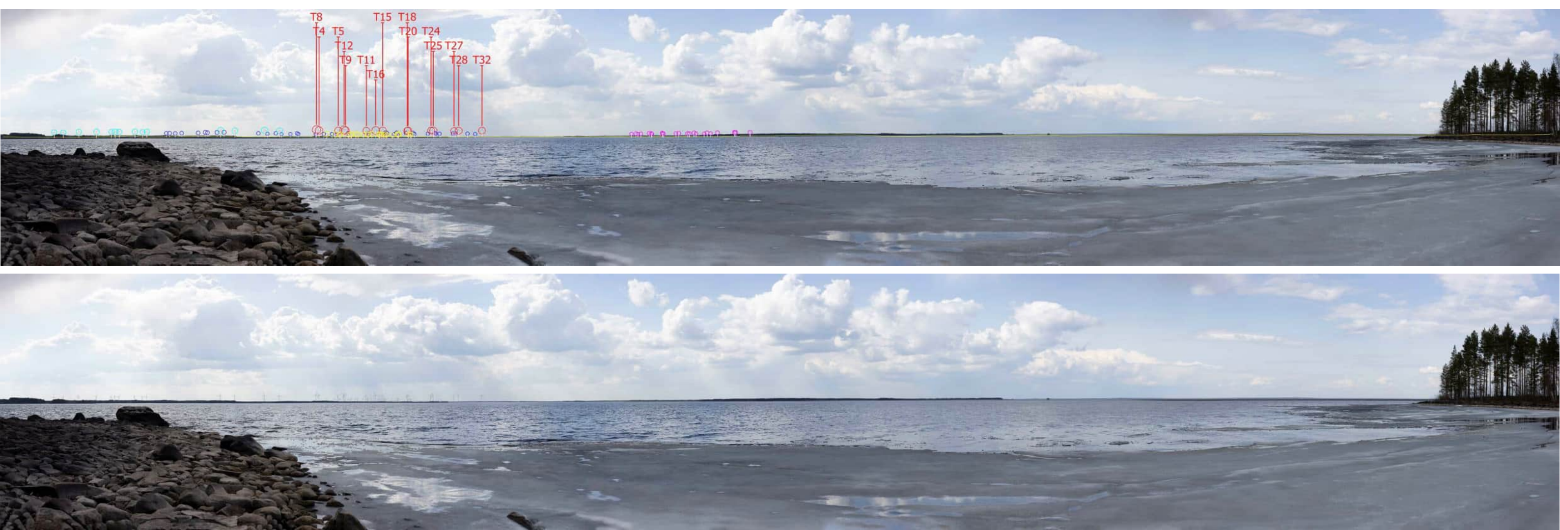
Kuva 277 ja 278. Valokuvasovite kuvauspisteessä 23, layout VE3. Kuva on otettu Kajaanin Vuottoniemestä, kuvaussuunta luoteeseen. Etäisyys voimaloihin on noin 15,1 kilometriä. Yläkuva draft ja alakuva varsinainen valokuvasovite. Löytösuon voimalat numeroitu ja korostettu punaisella. Toiminnassa olevat hankkeet korostettu Piiparinmäen voimalat sinisellä, Metsälamminkankaan voimalat pinkillä. Yhteisvaikutushankkeet korostettu kuvissa Kokkosuon voimalat turkoosilla, Pyöriännevan voimalat keltaisella, Luolakankaan voimalat vihreällä.
