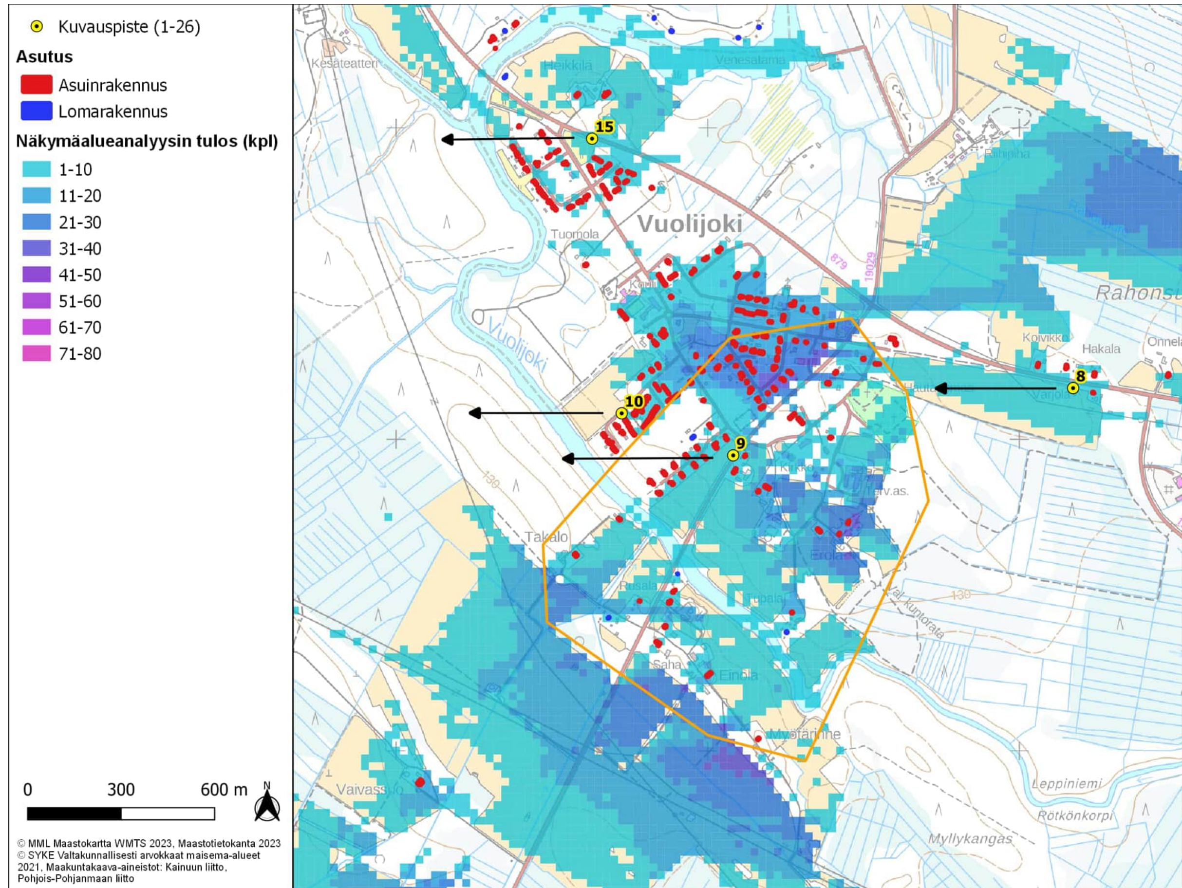
Kuva 118. Kuvauspiste 9. Löytösuon layout versio 3 (VE3) näkymäalueanalyysin laskentatulokset voimaloiden napakorkeudella mallinnettuna.
