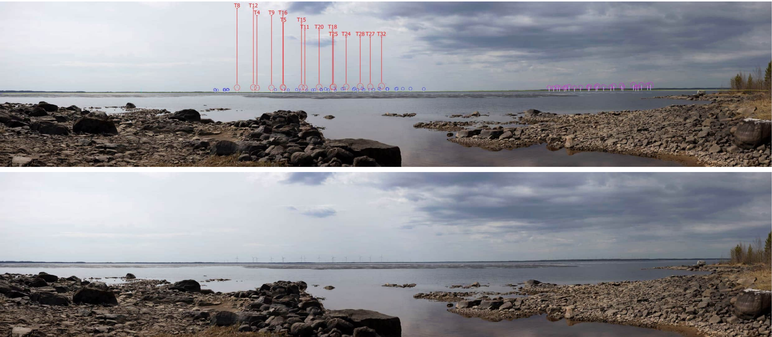
Kuva 263 ja 264. Valokuvassovite kuvauspisteessä 22, layout VE3. Kuva on otettu Vaalan Mustaniemestä, kuvaussuunta luoteeseen. Etäisyys voimaloihin on noin 13,6 kilometriä. Yläkuva draft ja alakuva varsinainen valokuvassovite. Löytösuon voimalat numeroitu ja korostettu punaisella. Toiminnassa olevat hankkeet korostettu Piiparinmäen voimalat sinisellä, Metsälammin kankaan voimalat pinkillä.
