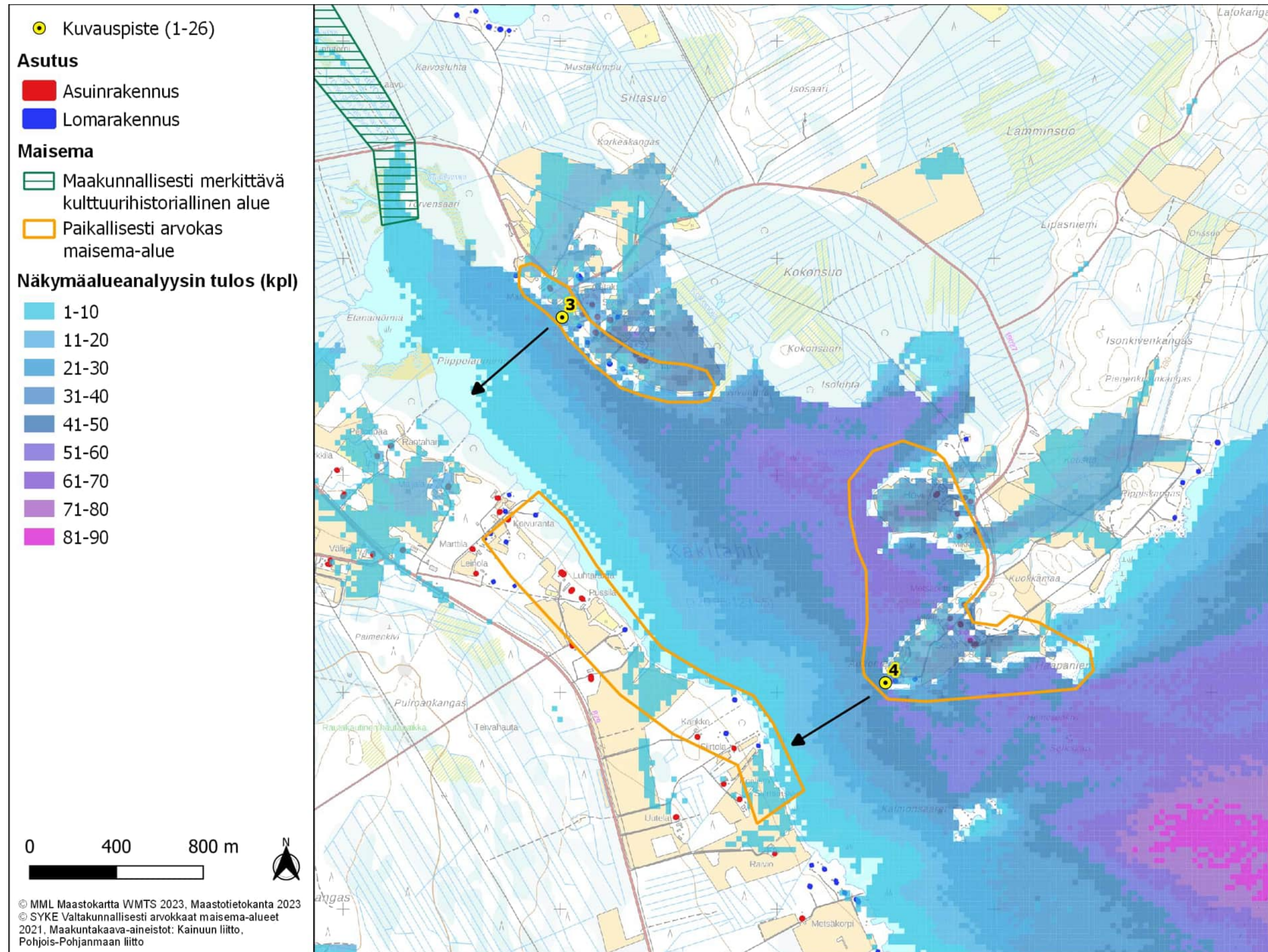
Kuva 36. Kuvauspiste 3, kuva otettu Kajaanin Kärkisaaresta. Löytösuon layout versio 2 (VE2) näkymäalueanalyysin laskentatulokset voimaloiden napakorkeudella mallinnettuna
