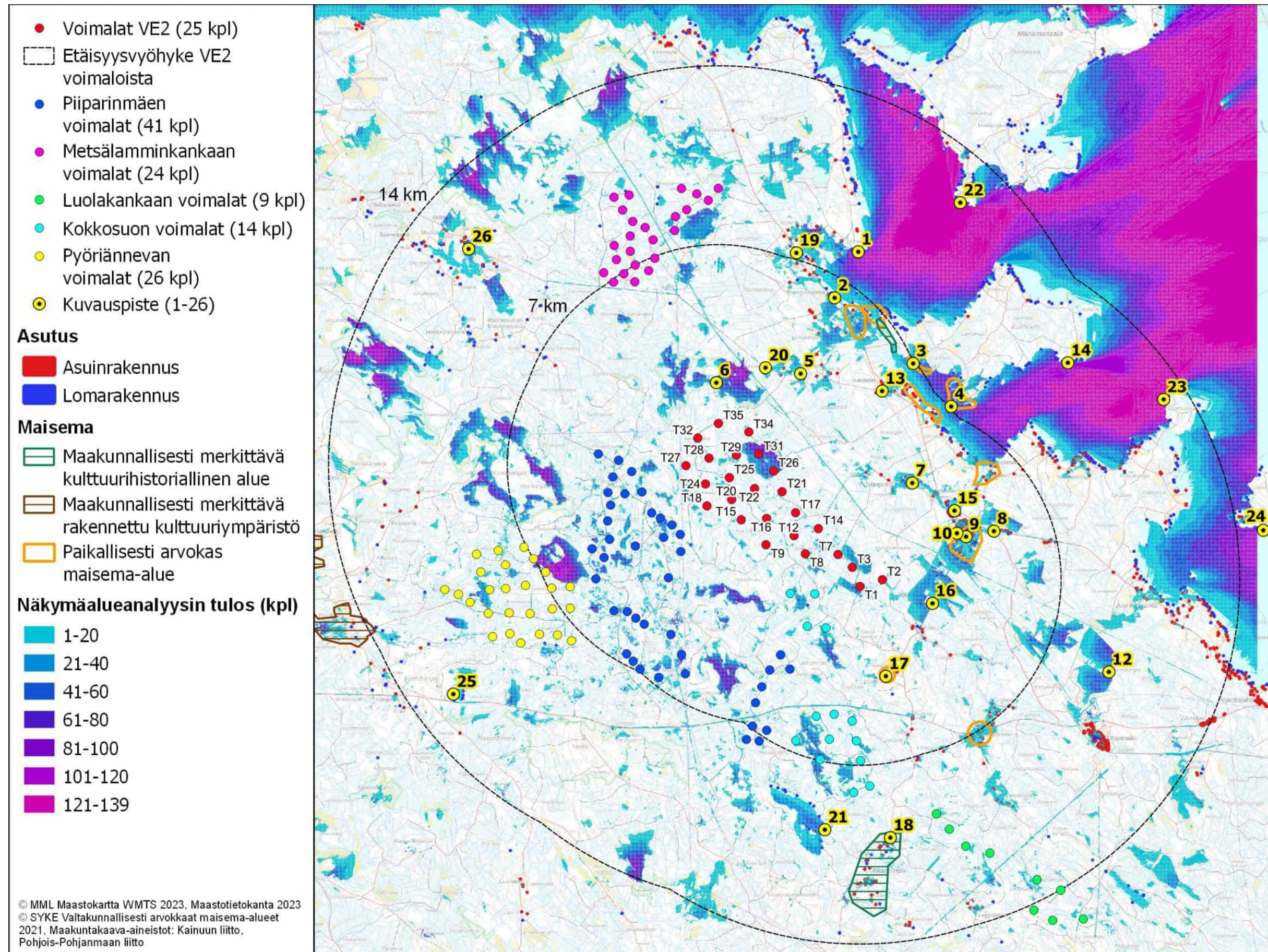
Kuva 4. Lötösuon layout versio 2 (VE2) näkymäalueanalyysin laskentatulokset voimaloiden napakorkeudella mallinnettuna. Lötösuon voimalat numeroitu ja korostettu punaisella. Toiminnassa olevat hankkeet korostettu väreillä, Piiparinmäen voimalat sinisellä, Metsäamminkankaan voimalat pinkillä. Yhteisvaikutushankkeet korostettu kuvissa Kokkosuon voimalat turkoosilla, Pyöriännevan voimalat keltaisella, Luolakankaan voimalat vihreällä.
