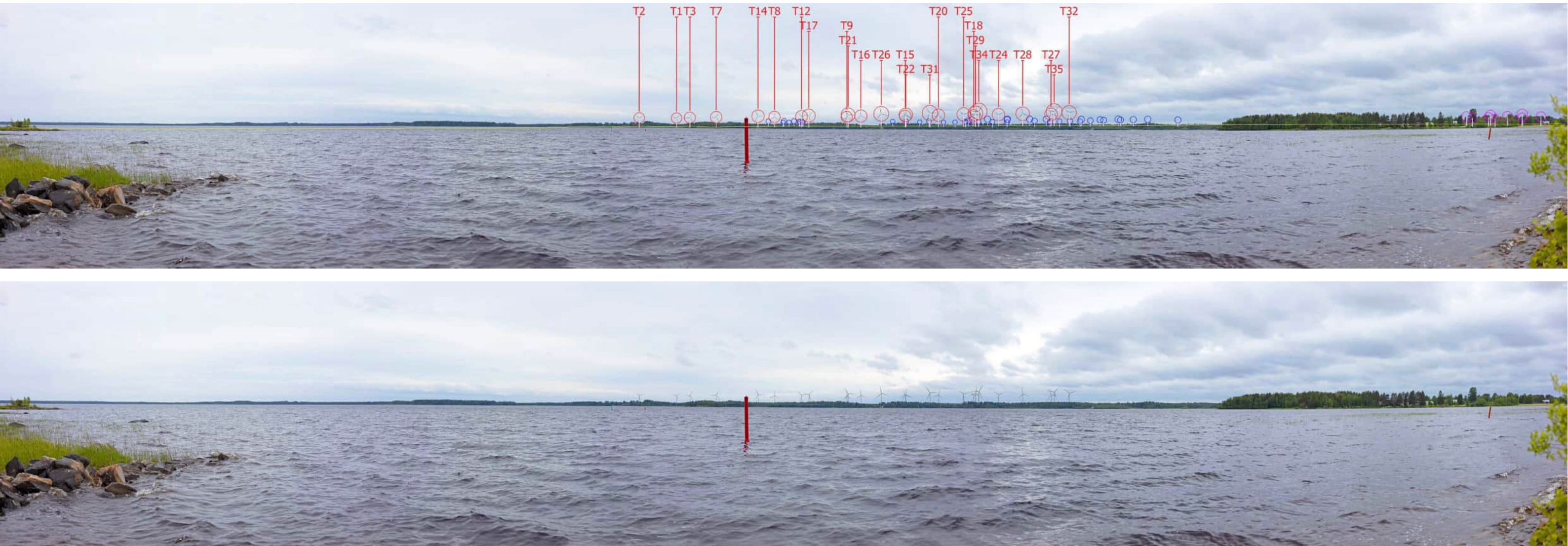
Kuva 11 ja 12. Valokuvasovite kuvauspisteessä 1, layout VE2. Kuva on otettu Kajaanista Kumpuniemestä, Oulunjärven rannalta, kuvaussuunta lounaaseen. Etäisyys voimaloihin on noin 8,5 kilometriä. Yläkuva draft ja alakuva varsinainen valokuvasovite. Löytösuon voimalat numeroitu ja korostettu punaisella. Toiminnassa olevat hankkeet korostettu Piiparinmäen voimalat sinisellä, Metsälamminkankaan voimalat pinkillä.
