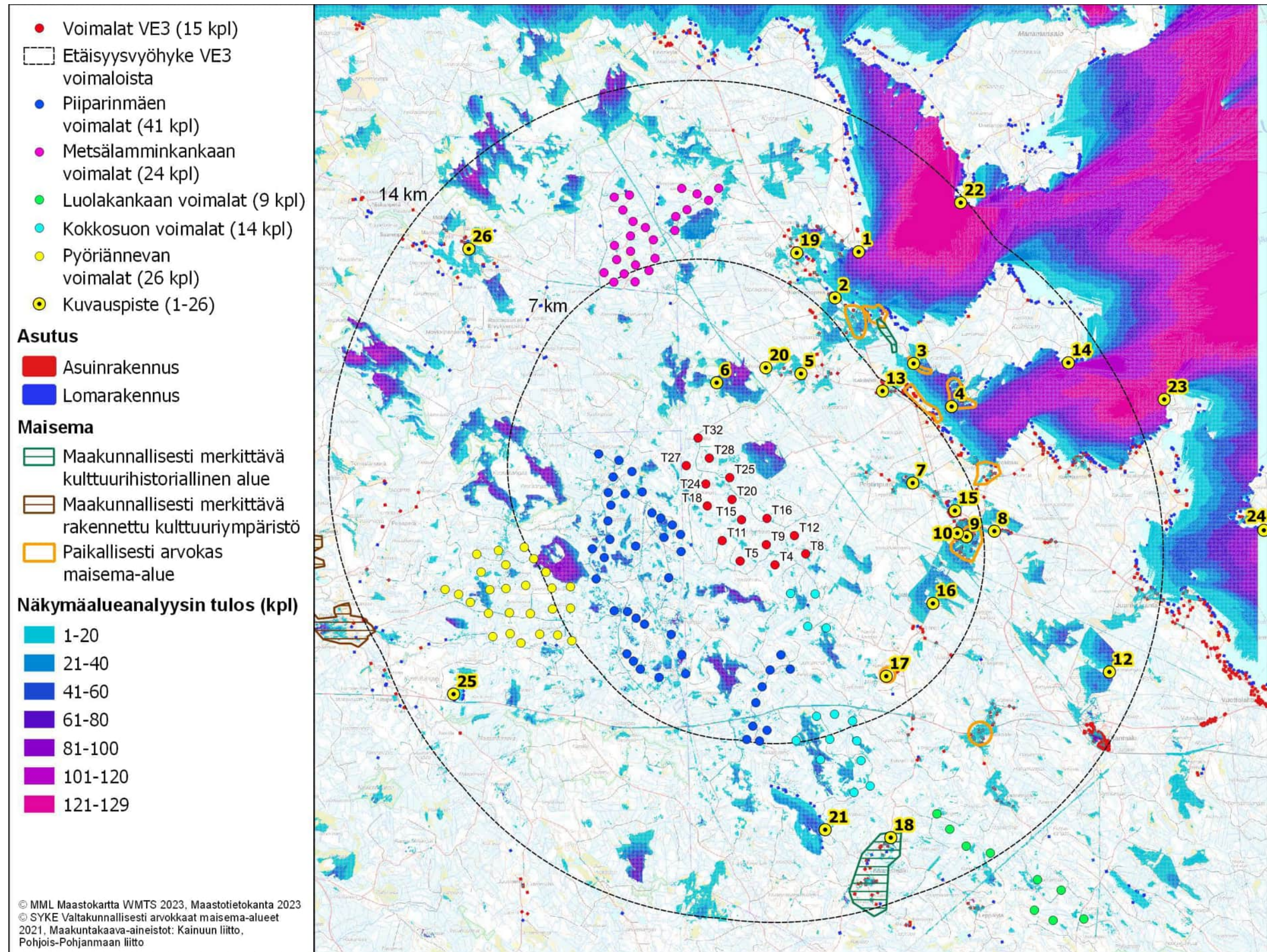
Kuva 6. Löytösuo layout versio 3 (VE3) näkymäalueanalyysin laskentatulokset voimaloiden napakorkeudella mallinnettuna. Löytösuo voimalat numeroitu ja korostettu punaisella. Toiminnassa olevat hankkeet korostettu väreillä, Piiparinmäen voimalat sinisellä, Metsälamminkankaan voimalat pinkillä. Yhteisvaikutushankkeet korostettu kuvissa Kokkosuon voimalat turkoosilla, Pyöriännevan voimalat keltaisella, Luolakankaan voimalat vihreällä
