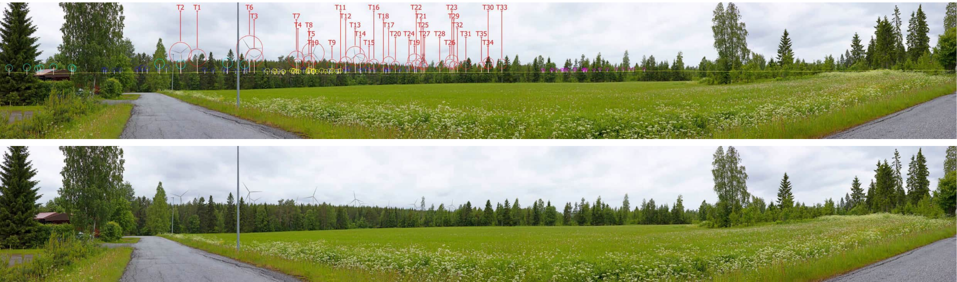
Kuva 125 ja 126. Valokuvasovite kuvauspisteessä 10, layout VE1. Kuva on otettu Kajaanin Vuolijoelta Vuolijoentieltä, kuvaussuunta länsi-luoteeseen. Etäisyys voimaloihin on noin 2,8 kilometriä. Yläkuva draft ja alakuva varsinainen valokuvasovite. Löytösuon voimalat numeroitu ja korostettu punaisella. Toiminnassa olevat hankkeet korostettu Piiparinmäen voimalat sinisellä, Metsälamminkankaan voimalat pinkillä. Yhteisvaikutushankkeet korostettu kuvissa Kokkosuon voimalat turkoosilla, Pyöriännevan voimalat keltaisella, Luolakankaan voimalat vihreällä.
