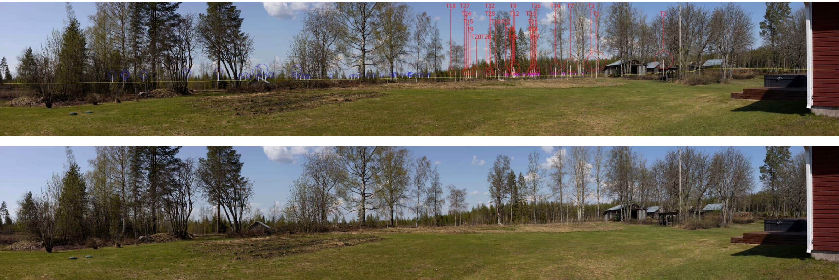
Kuva 199 ja 200. Valokuvasovite kuvauspisteessä 17, layout VE2. Kuva on otettu Kajaanin Ylä-honkamäestä, kuvaussuunta luoteeseen. Etäisyys voimaloihin on noin 3,8 kilometriä. Yläkuva draft ja alakuva varsinainen valokuvasovite. Löytösuon voimalat numeroitu ja korostettu punaisella. Toiminnassa olevat hankkeet korostettu Piiparinmäen voimalat sinisellä, Metsälamminkankaan voimalat pinkillä.
