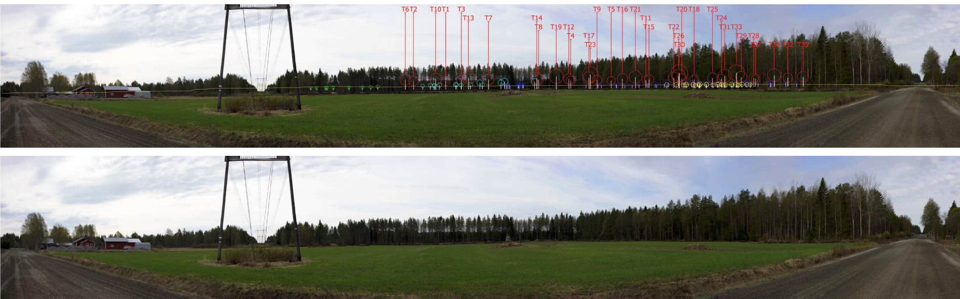
Kuva 149 ja 150. Valokuvasovite kuvauspisteessä 13, layout VE1. Kuva on otettu Kajaanin Käkilahdesta, kuvaussuunta etelä-lounaaseen. Etäisyys voimaloihin on noin 4,4 kilometriä. Yläkuva draft ja alakuva varsinainen valokuvasovite. Löytösuon voimalat numeroitu ja korostettu punaisella. Toiminnassa olevat hankkeet korostettu Piiparinmäen voimalat sinisellä, Metsäamminkankaan voimalat pinkillä. Yhteisvaikutushankkeet korostettu kuvissa Kokkosuon voimalat turkoosilla, Pyöriännevan voimalat keltaisella, Luolakankaan voimalat vihreällä.
