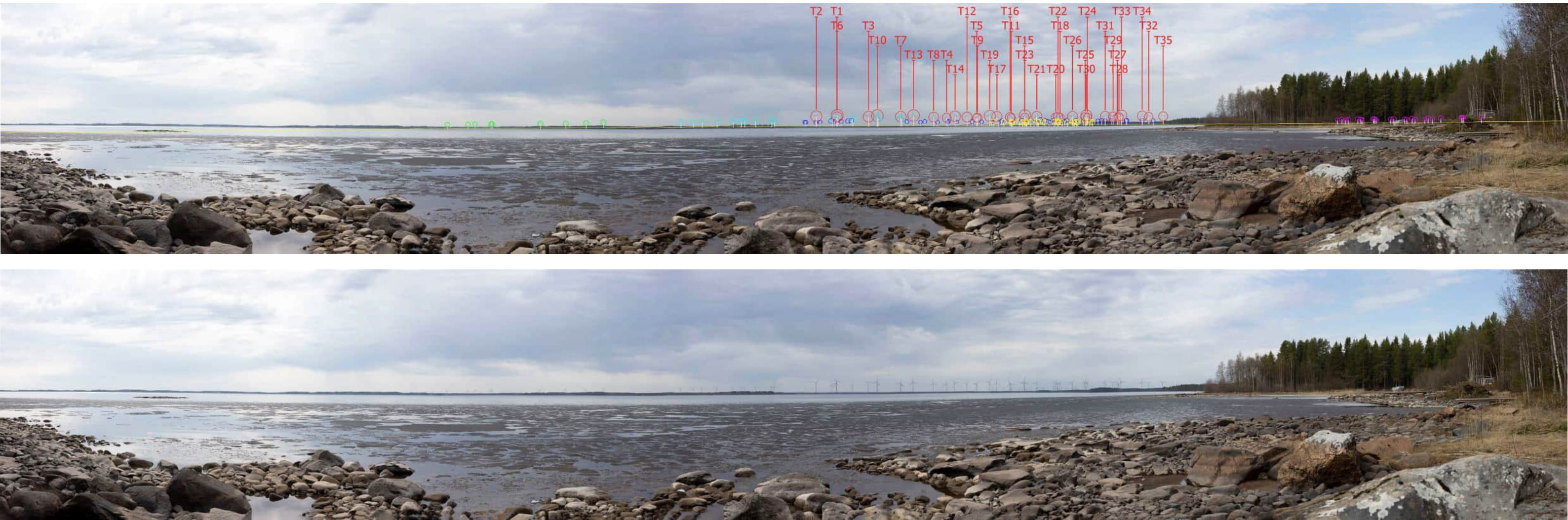
Kuva 161 ja 162. Valokuvaseite kuvapisteessä 14, layout VE1. Kuva on otettu Kajaanin Kärkisaaresta Someronniemen rannalta, kuvaussuunta luoteeseen. Etäisyys voimaloihin on noin 11,2 kilometriä. Yläkuva draft ja alakuva varsinainen valokuvaseite. Löytösuon voimalat numeroitu ja korostettu punaisella. Toiminnassa olevat hankkeet korostettu Piiparinmäen voimalat sinisellä, Metsälamminkaan voimalat pinkillä. Yhteisvaikutushankkeet korostettu kuvissa Kokkosuon voimalat turkoosilla, Pyöriännevan voimalat keltaisella, Luolakankaan voimalat vihreällä.
