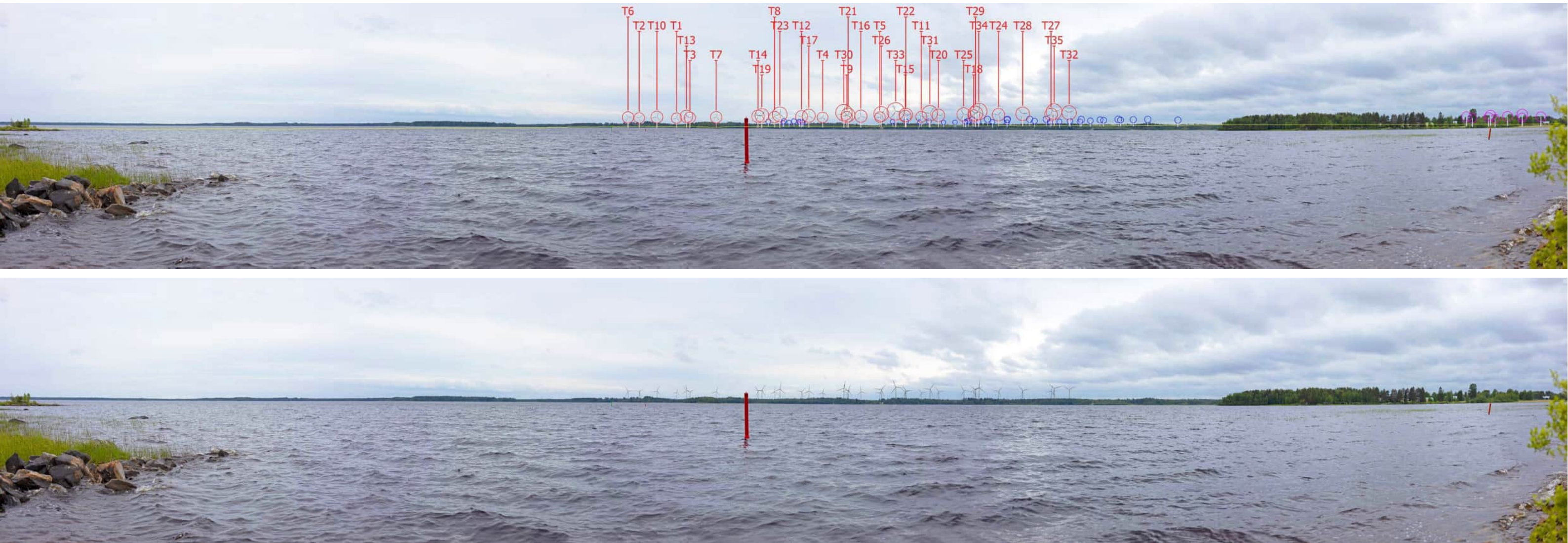
Kuva 7 ja 8. Valokuvasevite kuvauspisteessä 1, layout VE1. Kuva on otettu Kajaanista Kumpuniemestä Oulunjärven rannalta, kuvaussuunta lounaaseen. Etäisyys voimaloihin on noin 8,5 kilometriä. Yläkuva draft ja alakuva varsinainen valokuvasevite. Löytösuon voimalat numeroitu ja korostettu punaisella. Toiminnassa olevat hankkeet korostettu Piiparinmäen voimalat sinisellä, Metsäamminkankaan voimalat pinkillä.
