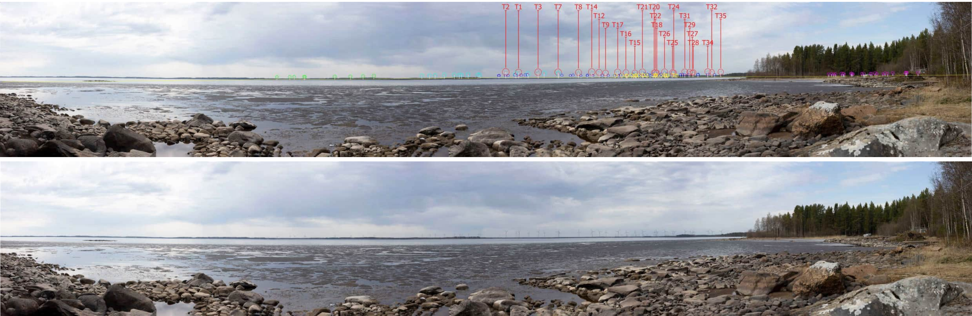
Kuva 165 ja 166. Valokuvasovite kuvauspisteessä 14, layout VE2. Kuva on otettu Kajaanin Kärkisaaresta Someronniemen rannalta, kuvaussuunta luoteeseen. Etäisyys voimaloihin on noin 12,1 kilometriä. Yläkuva draft ja alakuva varsinainen valokuvasovite. Löytösuon voimalat numeroitu ja korostettu punaisella. Toiminnassa olevat hankkeet korostettu Piiparinmäen voimalat sinisellä, Metsälamminkankaan voimalat pinkillä. Yhteisvaikutushankkeet korostettu kuvissa Kokkosuon voimalat turkoosilla, Pyöriännevan voimalat keltaisella, Luolakankaan voimalat vihreällä.
