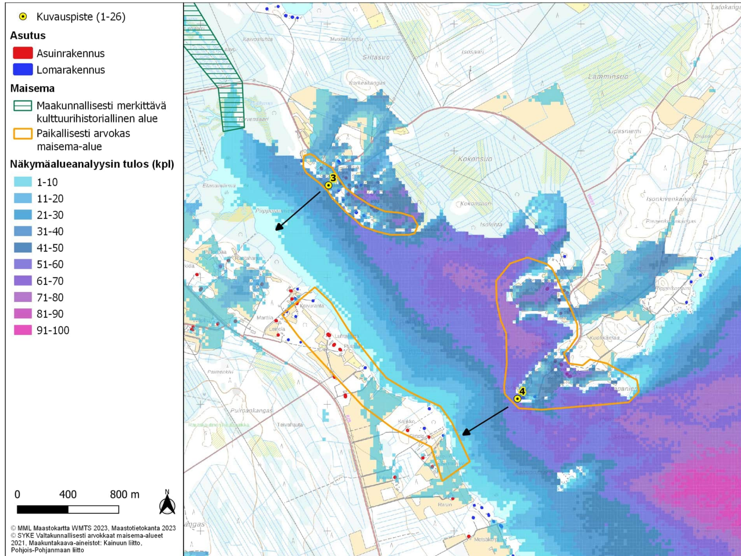
Kuva 31. Kuvauspiste 3, kuva otettu Kajaanin Kärkisaaresta. Löytösuon layout versio 1 (VE1) näkymäalueanalyysin laskentatulokset voimaloiden napakorkeudella mallinnettuna.
