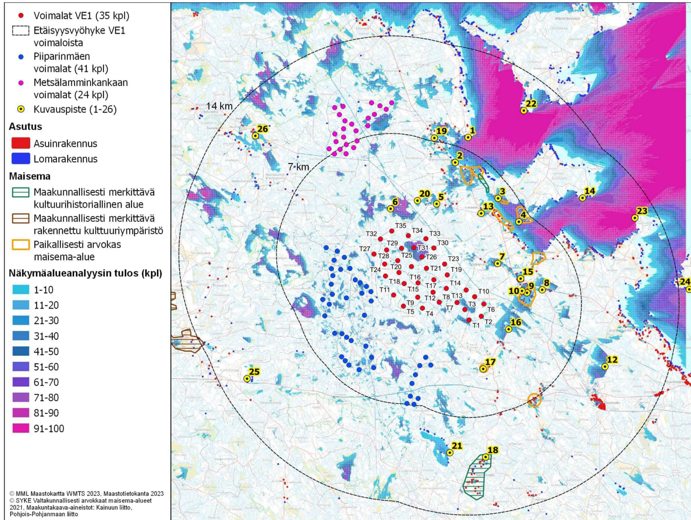
Kuva 1. Löytösuon layout versio 1 (VE1) näkymäalueanalyysin laskentatulokset voimaloiden napakorkeudella mallinnettuna. Löytösuon voimalat numeroitu ja korostettu punaisella. Toiminnassa olevat hankkeet korostettu väreillä, Piiparinmäen voimalat sinisellä, Metsäamminkankaan voimalat pinkillä.
