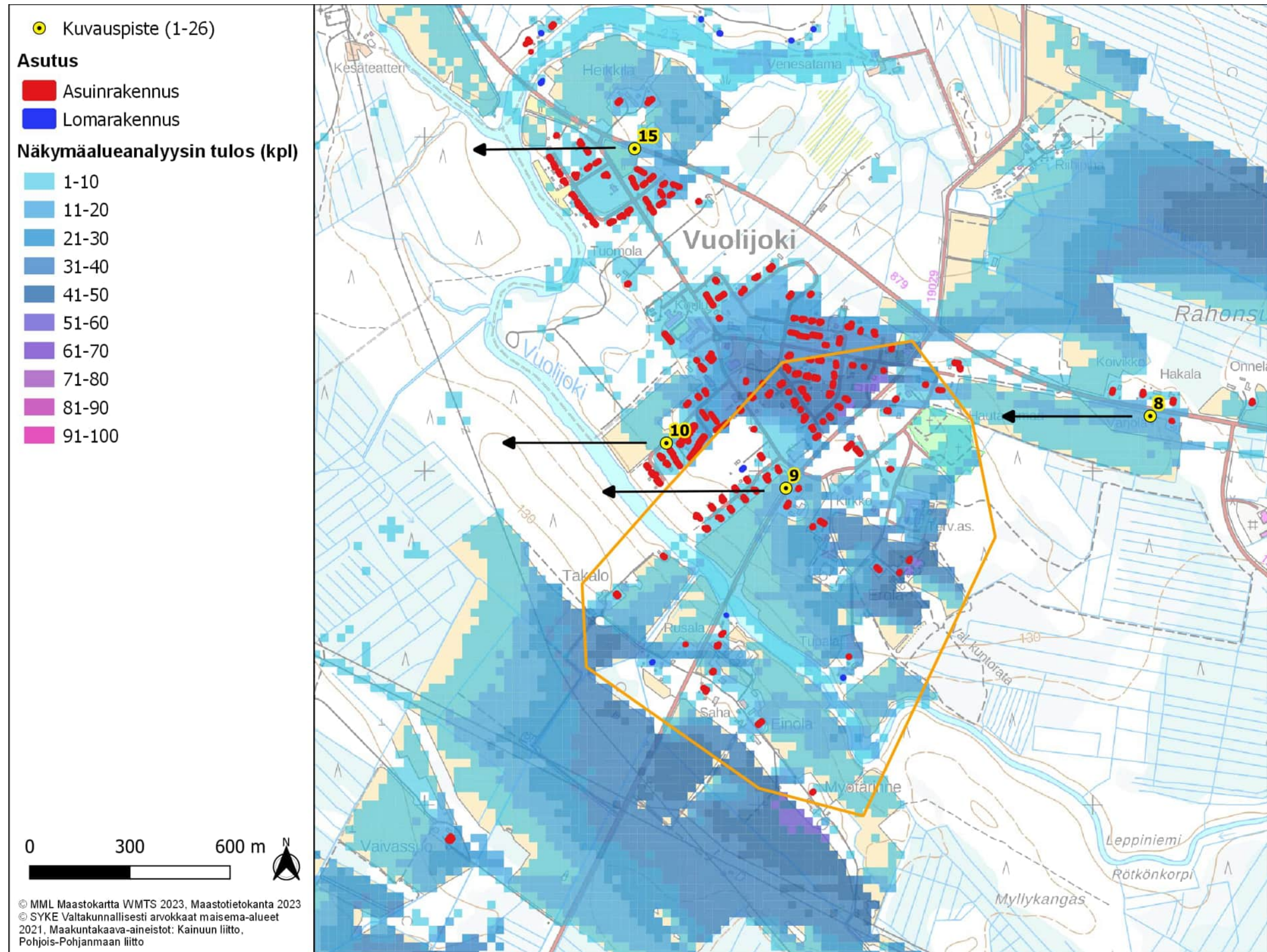
Kuva 108. Kuvauspiste 9. Löytösuon layout versio 1 (VE1) näkymäalueanalyysin laskentatulokset voimaloiden napakorkeudella mallinnettuna.
