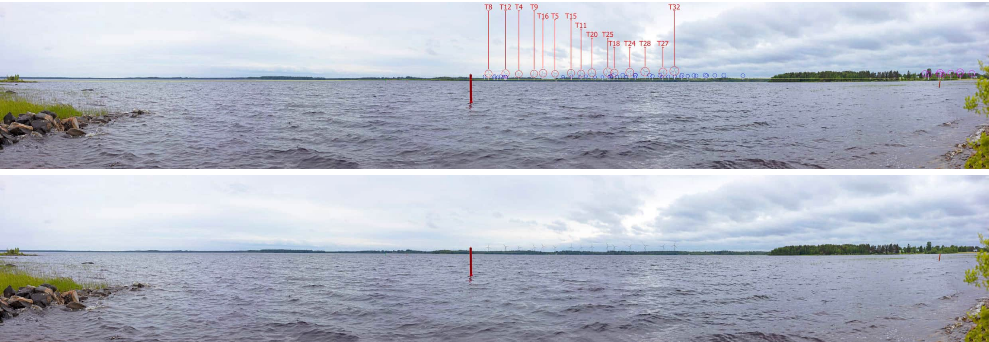
Kuva 15 ja 16. Valokuvasovite kuvauspisteessä 1, layout VE3. Kuva on otettu Kajaanista Kumpuniemestä, Oulunjärven rannalta, kuvaussuunta lounaaseen. Etäisyys voimaloihin on noin 9,5 kilometriä. Yläkuva draft ja alakuva varsinainen valokuvasovite. Löytösuon voimalat numeroitu ja korostettu punaisella. Toiminnassa olevat hankkeet korostettu Piiparinmäen voimalat sinisellä, Metsäamminkankaan voimalat pinkillä.
