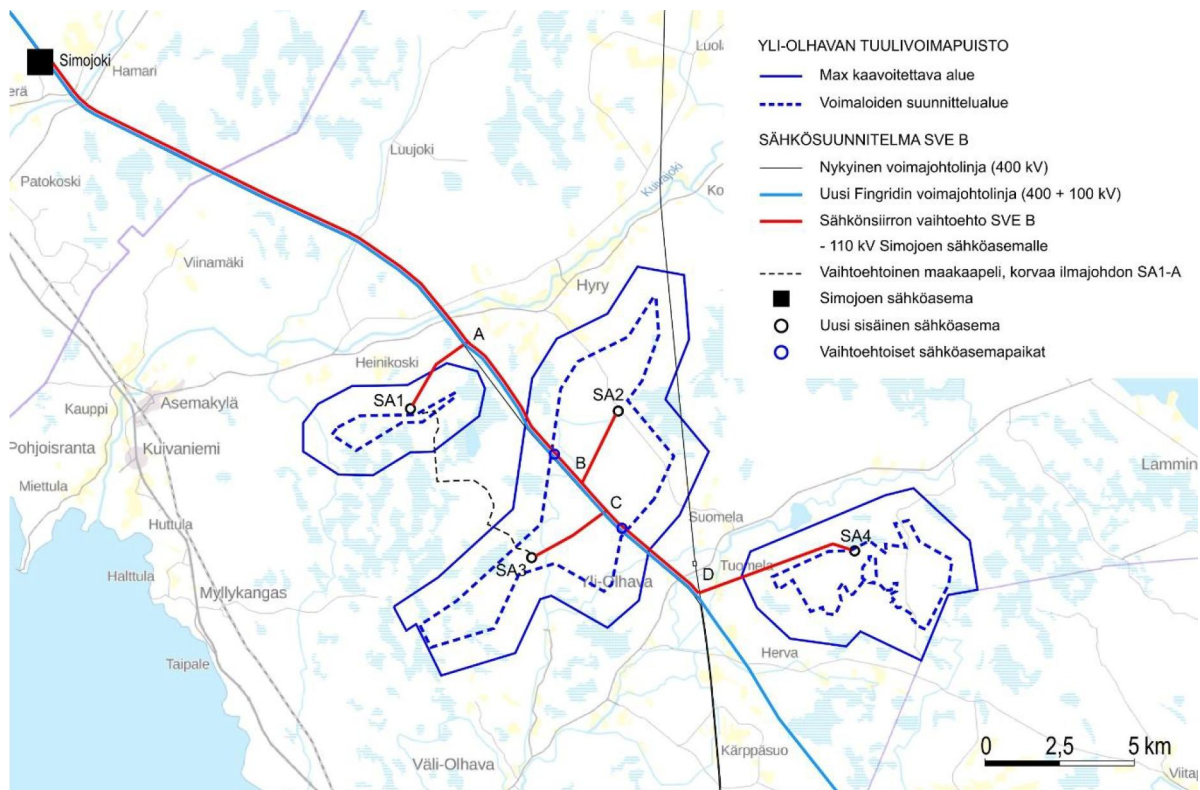
Kuva 6. Yli-Olhavan tuulivoimapuiston sähkönsiirtovaihtoehto SVE B.
