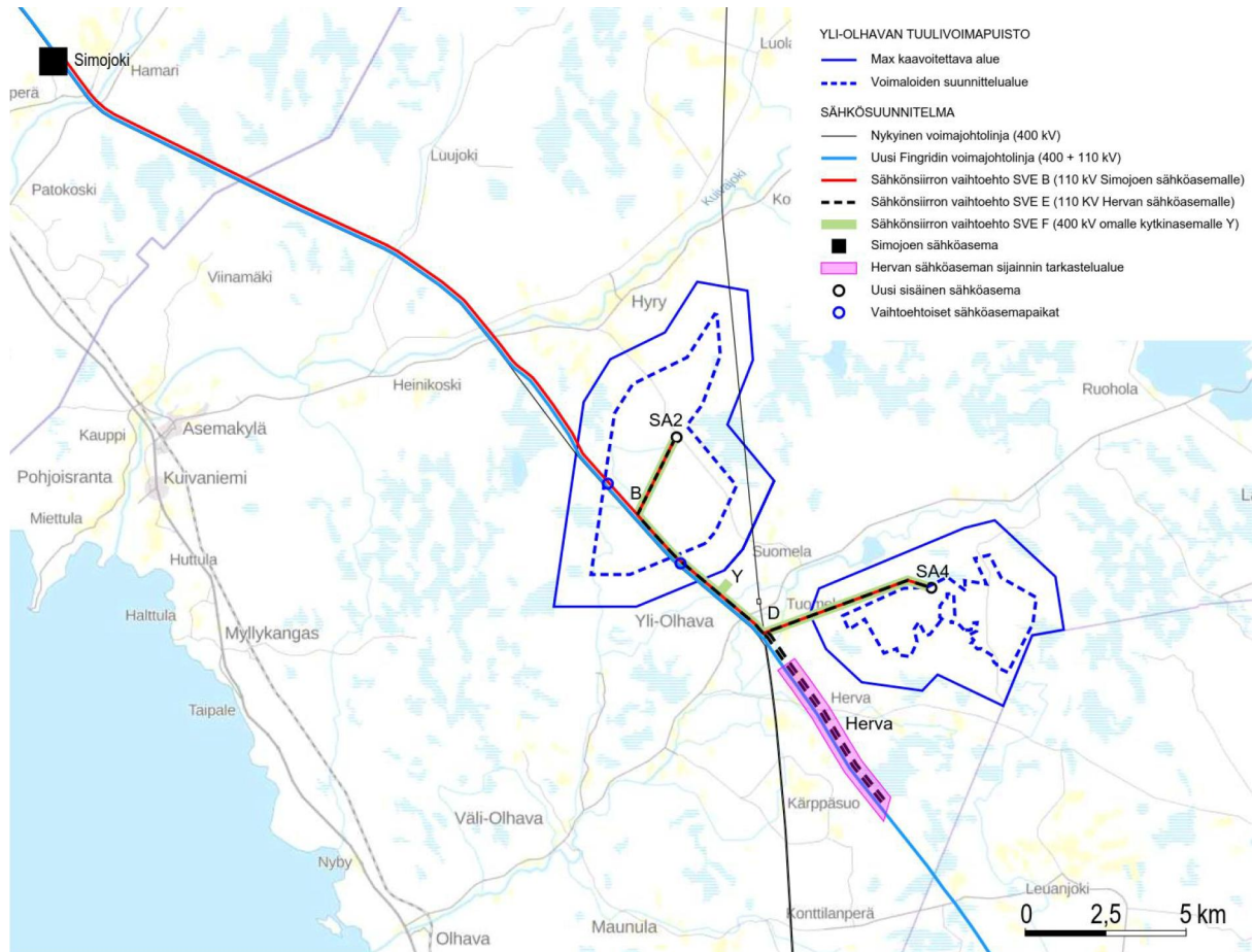
Kuva 9. Sähkönsiirtovaihtoehdot hankevaihtoehdossa VE2.
