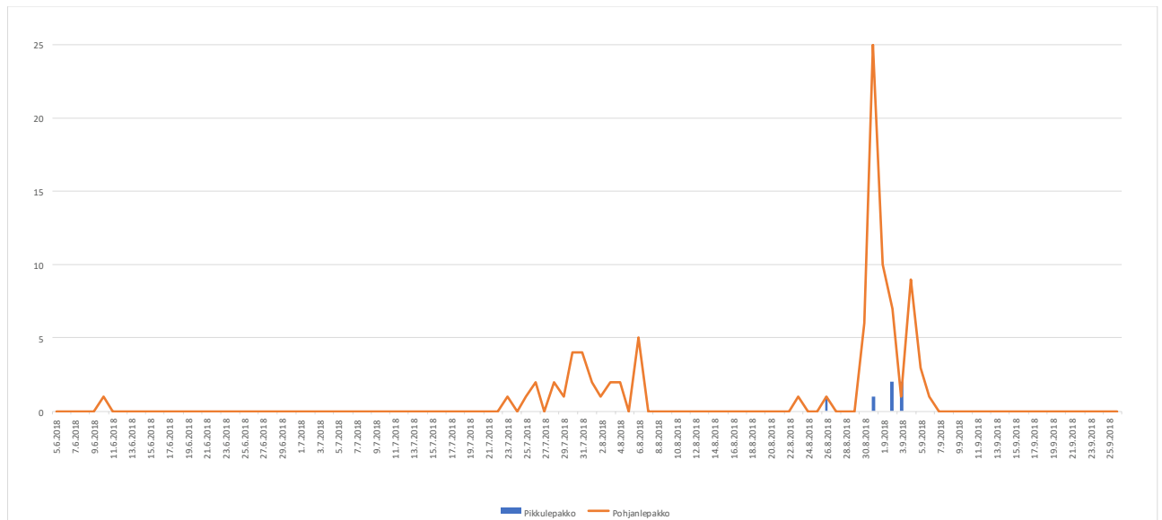
Kuva 35. Passiividetektorien lepakkohavainnot (yhdessä minuutissa aktiivisuusjaksojen lukumäärä) ajalla 5.6. -26.9.2018 Yli-Olhavan selvitysalueella.
