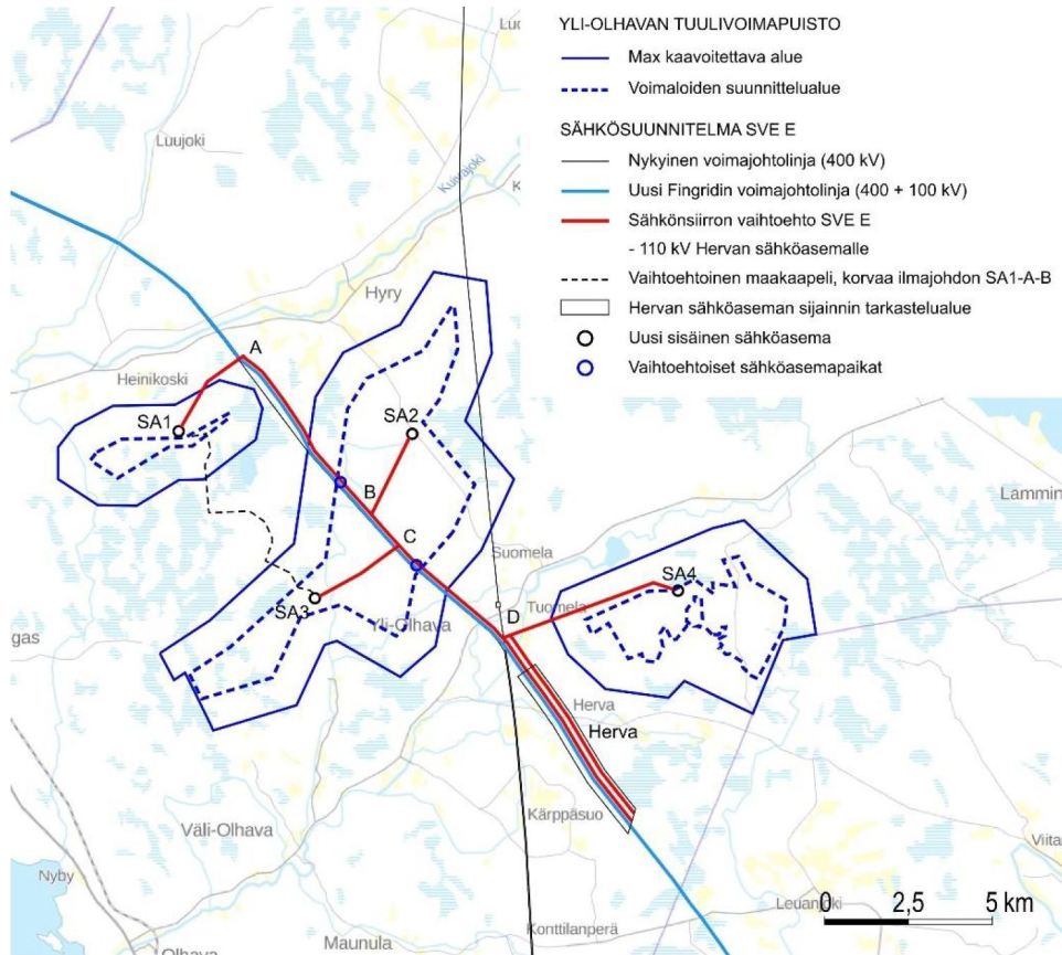
Kuva 7. Yli-Olhavan tuulivoimapuiston sähkönsiirtovaihtoehto SVE E.
