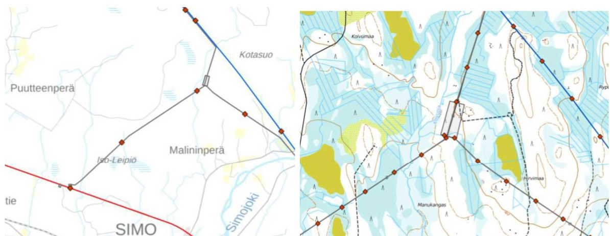
Kuva 10. Suunnitellun Simojoen sähköaseman alustava sijoitusuunnitelma (Fingrid Oyj 06/2019).
