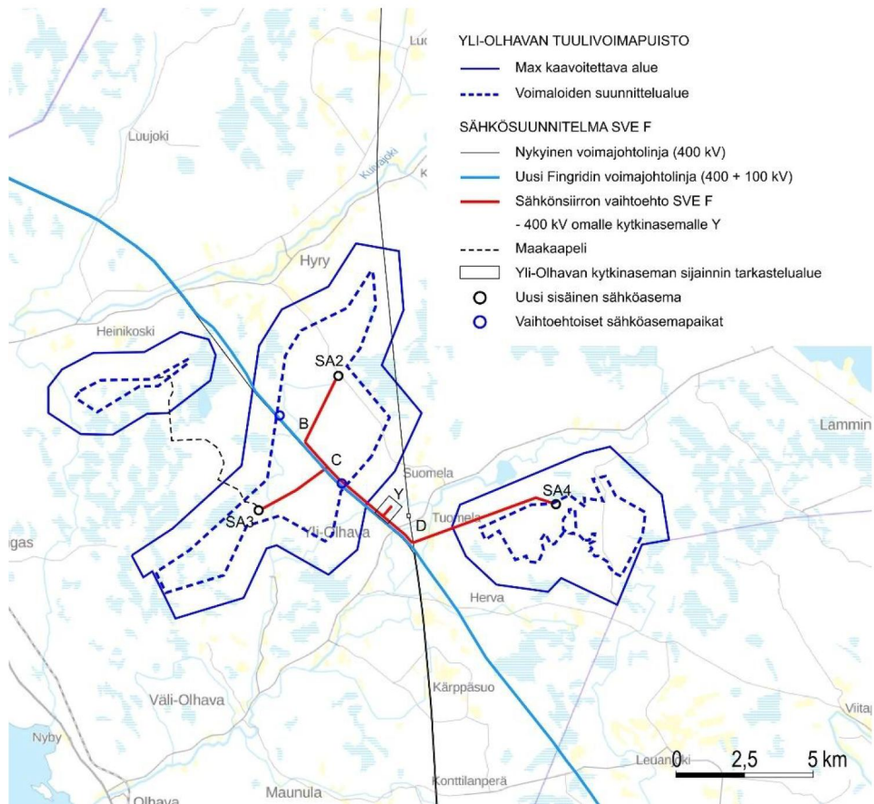
Kuva 8. Yli-Olhavan tuulivoimapuiston sähkönsiirtovaihtoehto SVE F.
