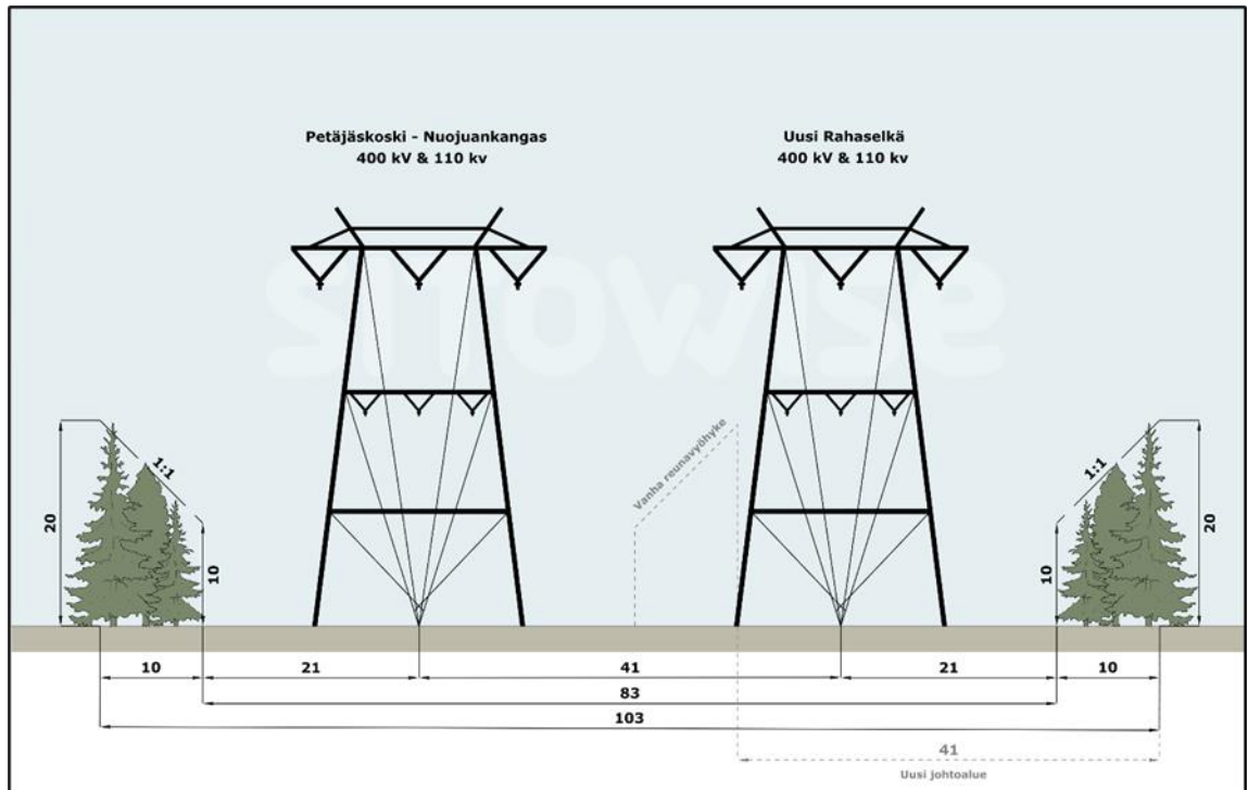
Kuva 3.5 Rahaselkä tuulivoimahankkeen 400 + 110 kV voimajohto rakenteilla olevan Petäjäskoski - Nuovuankangas 400 + 110 kV voimajohdon pohjoispuolella osuudella Tainijoki - Saunakummun sähköasema (jakso d-e).
