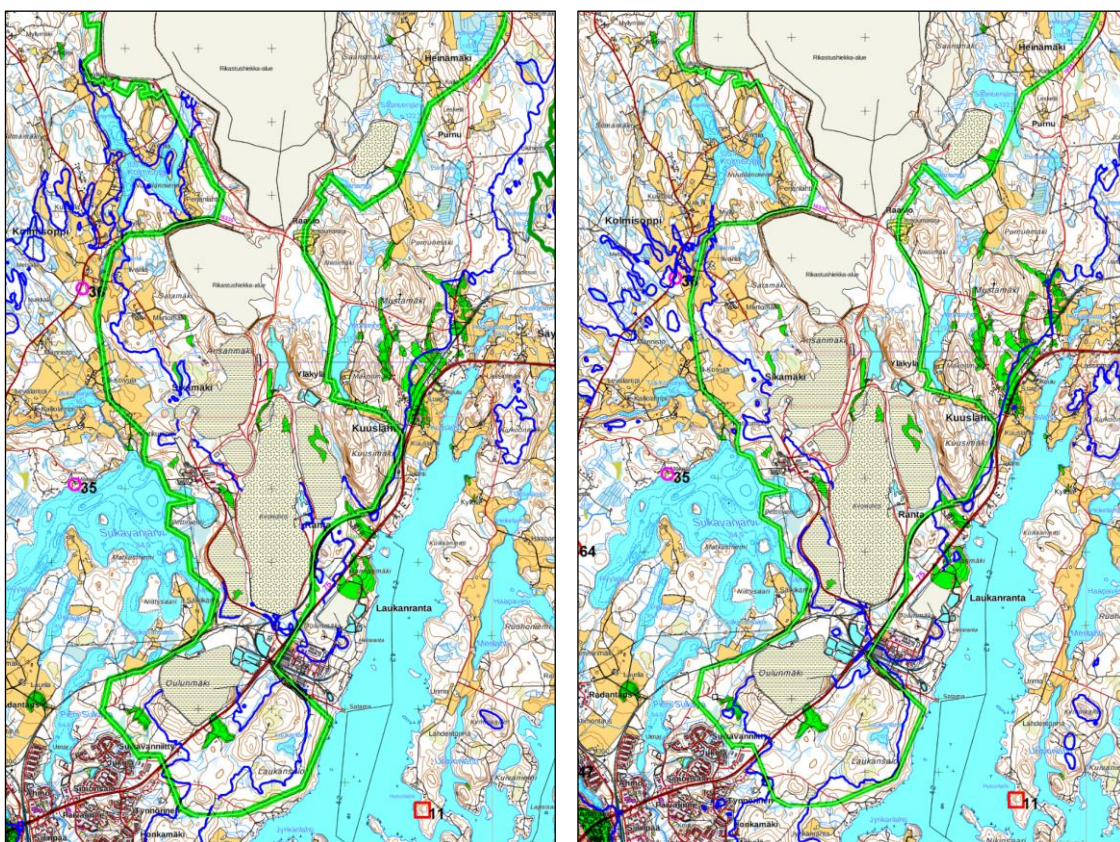
Sinisellä viivalla ranta v. 8000 ja 4700 eKr. Saimaan korkeimman rannan huipun aikana. Hiekkamaaperät (metrin syvyydessä) vihreinä alueina. tutkimusalueen raja-alue vaalean vihreällä viivalla.
