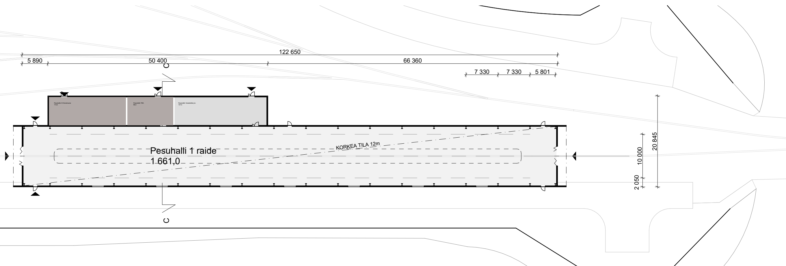
1. kerros pesuhalli 1:500
