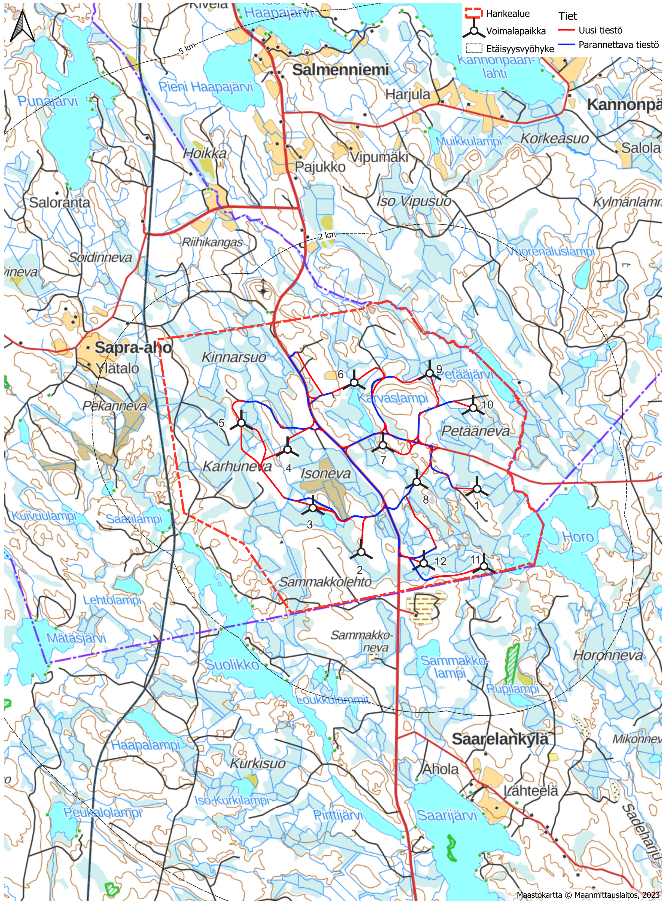
Tuulivoimahanke Tukkimäki, Karstula VE1, 12 voimalaa
