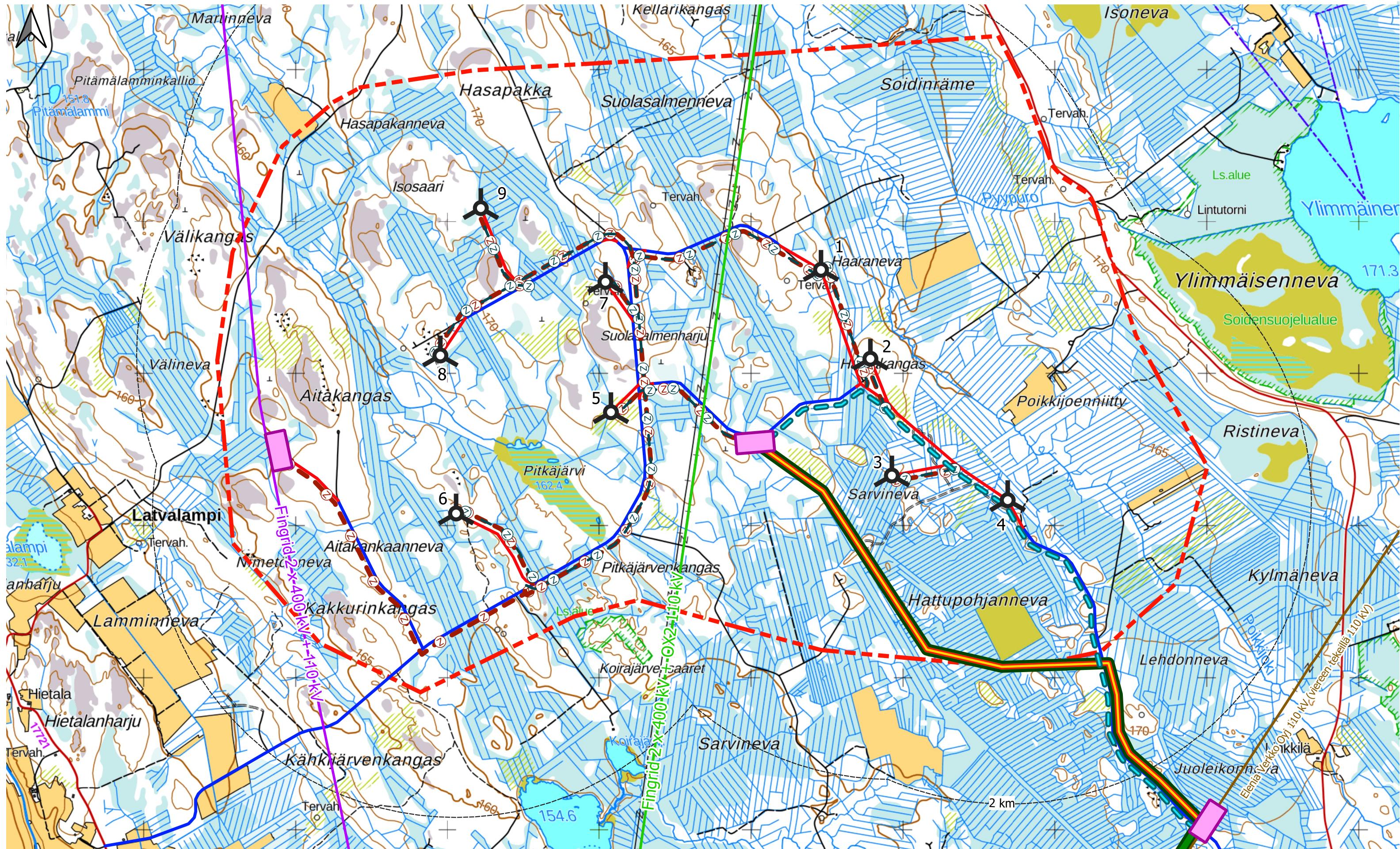
Tuulivoimahanke Suolasalmenharju, Alajärvi VE1, 9 voimalaa
