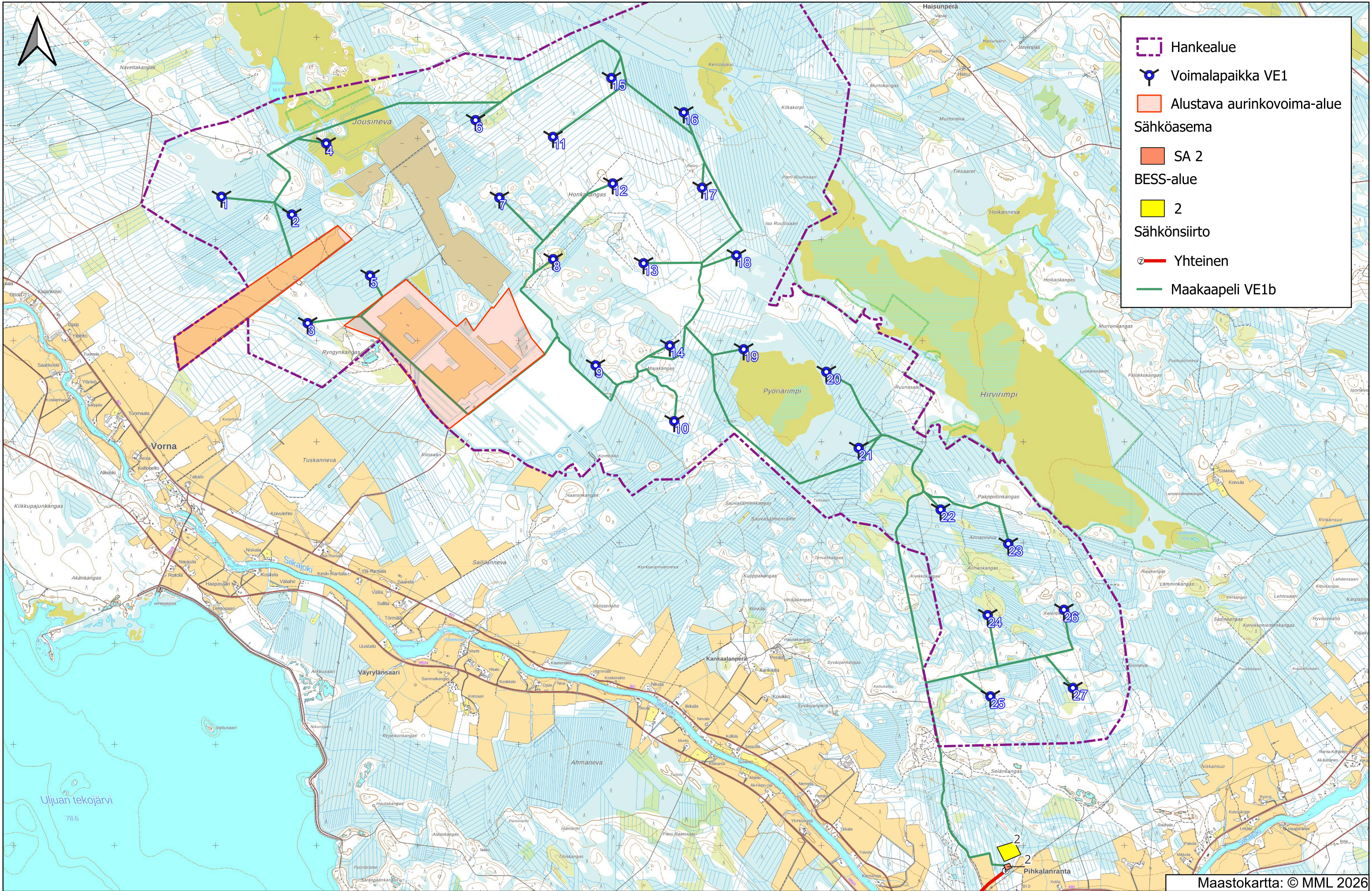
Honkakankaan tuuli- ja aurinkovoimahanke, Siikalatva VE1, Sisäinen sähkönsiirto B
