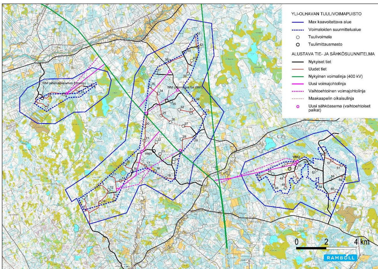
Tuulivoimapuiston suunnitelmakartta.
