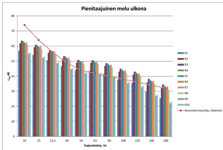
Kuva 5. VE3 pienitaajuisen ulkomelun laskentatulokset reseptoripisteissä
