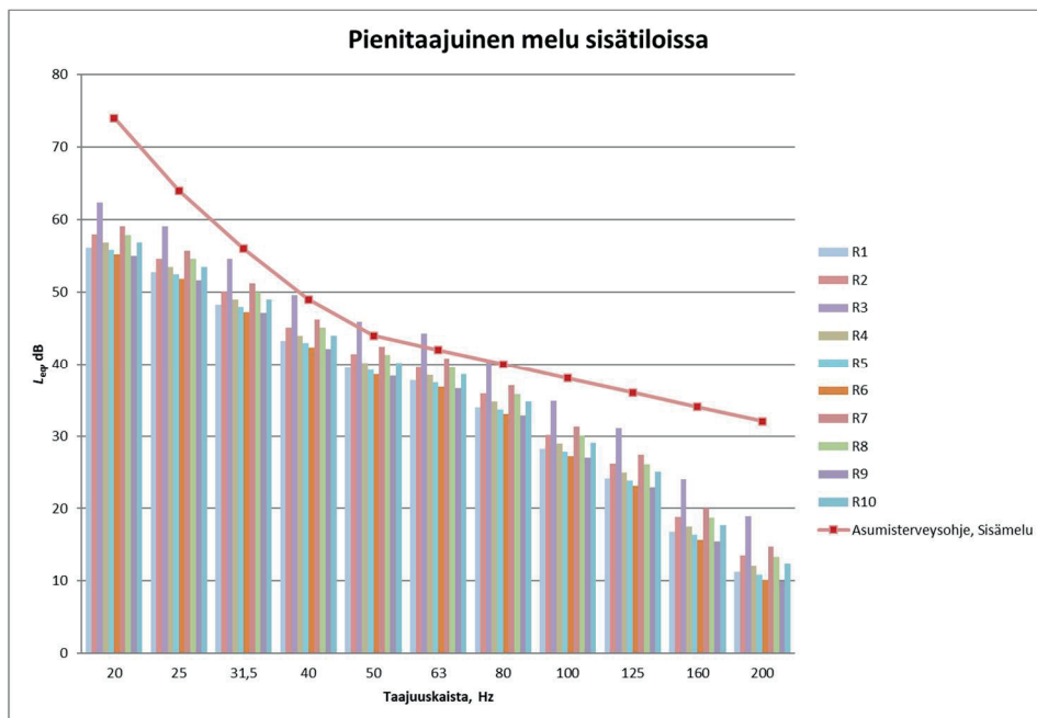
Kuva 2. VE1 pienitaajuisen sisämelun laskentatulokset reseptoripisteissä
