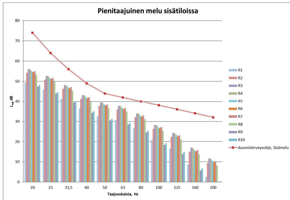
Kuva 4. VE3 pienitaajuisen sisämelun laskentatulokset reseptoripisteissä
