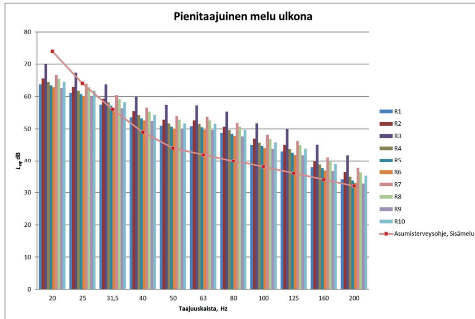
Kuva 3. VE1 pienitaajuisen ulkomelun laskentatulokset reseptoripisteissä
