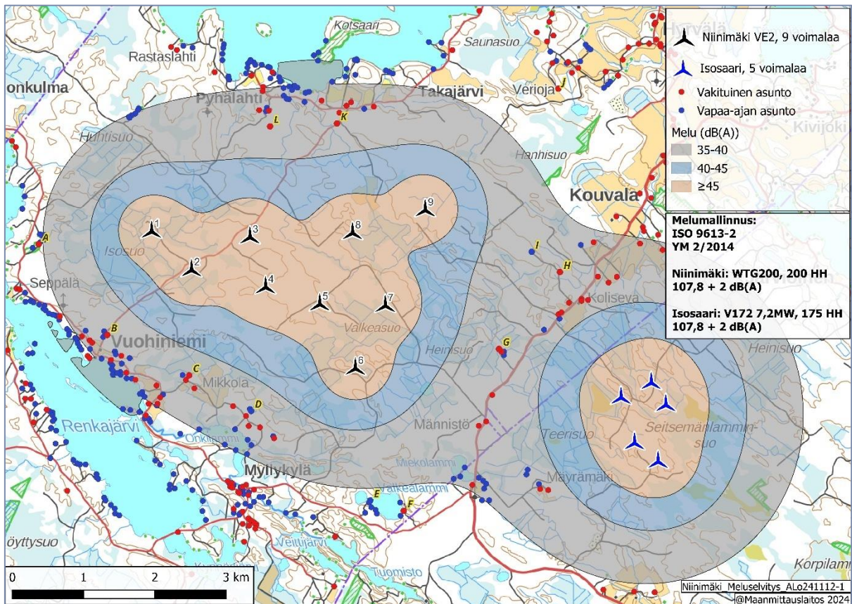
Kuva 4. Niinimäen tuulivoimahankkeen (VE2), WTG200 7,2MW, 200 m HH, 107,8 + 2,0 dB(A), ja läheisen tuulivoimahankkeen, Isosaaren, yhteisvaikutusten melumallinnus. Kaksitoista havainnointipistettä on merkitty kuvaan kirjaimilla (A-L).
