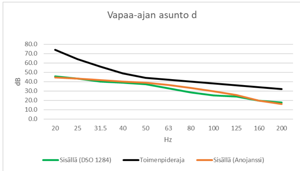
Kuva 12. Ympäristöministeriön ohjeistuksen mukainen pienitaajuuden melun laskenta sekä sosiaali- ja terveysministeriön toimenpiderajat vapaa-ajan asunnossa d.
