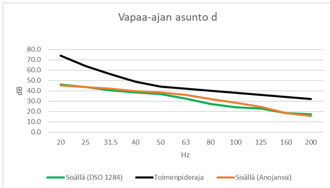
Kuva 10. Ympäristöministeriön ohjeistuksen mukainen pienitaajuisen melun laskenta sekä sosiaali- ja terveysministeriön toimenpiderajat vapaa-ajan asunnossa d.
