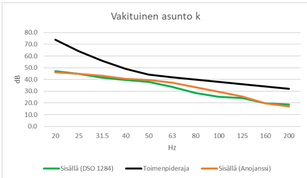
Kuva 5. Ympäristöministeriön ohjeistuksen mukainen pienitaajuisen melun laskenta sekä sosiaali- ja terveysministeriön toimenpiderajat vakituuisessa asunnossa k.
