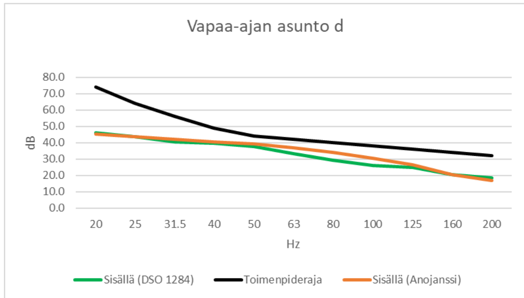
Kuva 6. Ympäristöministeriön ohjeistuksen mukainen pienitaajuisen melun laskenta sekä sosiaali- ja terveysministeriön toimenpiderajat vapaa-ajan asunnossa d.
