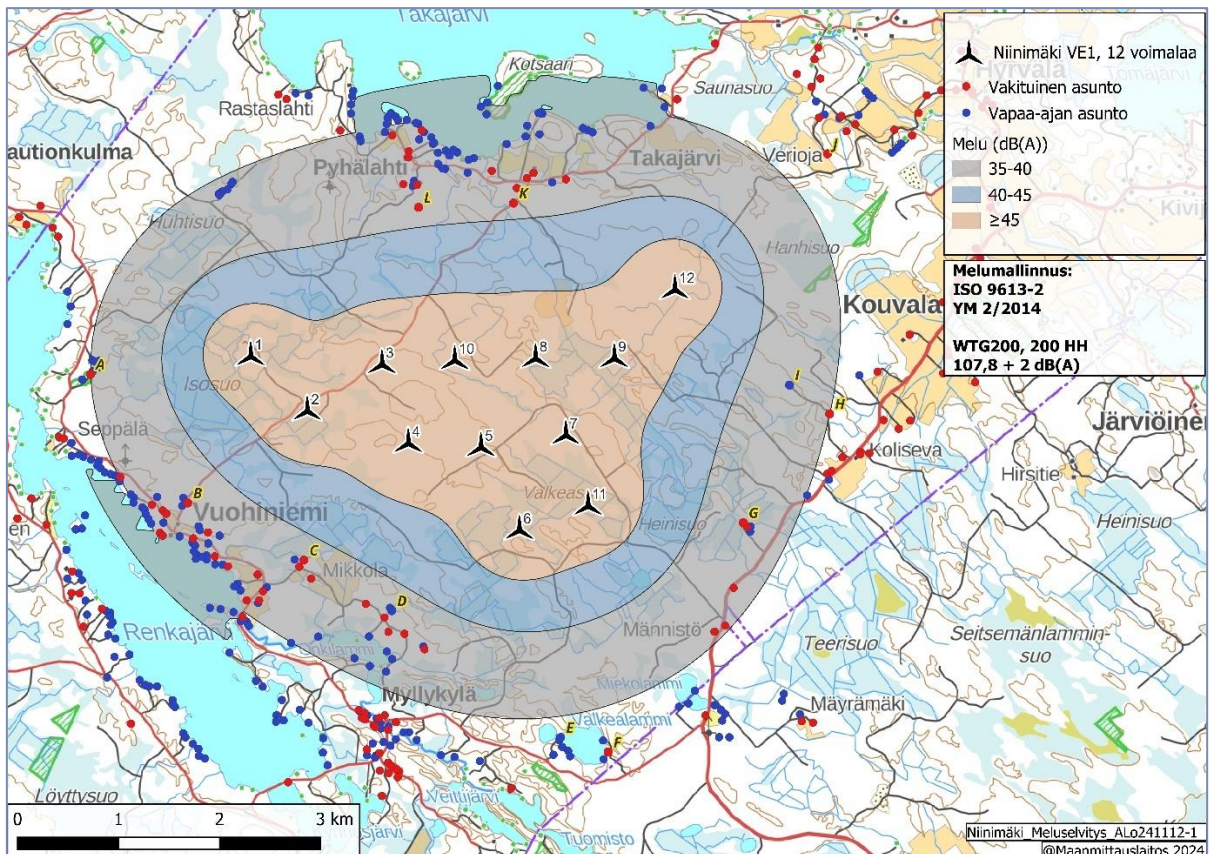
Kuva 1. Niinimäen tuulivoima-alueen melumallinnus (VE1), WTG200 7,2MW, 200 m HH, 107,8 + 2,0 dB(A). Kaksitoista havainnointipistettä on merkitty kuvaan kirjaimilla (A-L).
