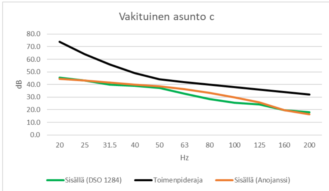
Kuva 11. Ympäristöministeriön ohjeistuksen mukainen pienitaajuisen melun laskenta sekä sosiaali- ja terveysministeriön toimenpiderajat vakituiseissa asunnossa c.
