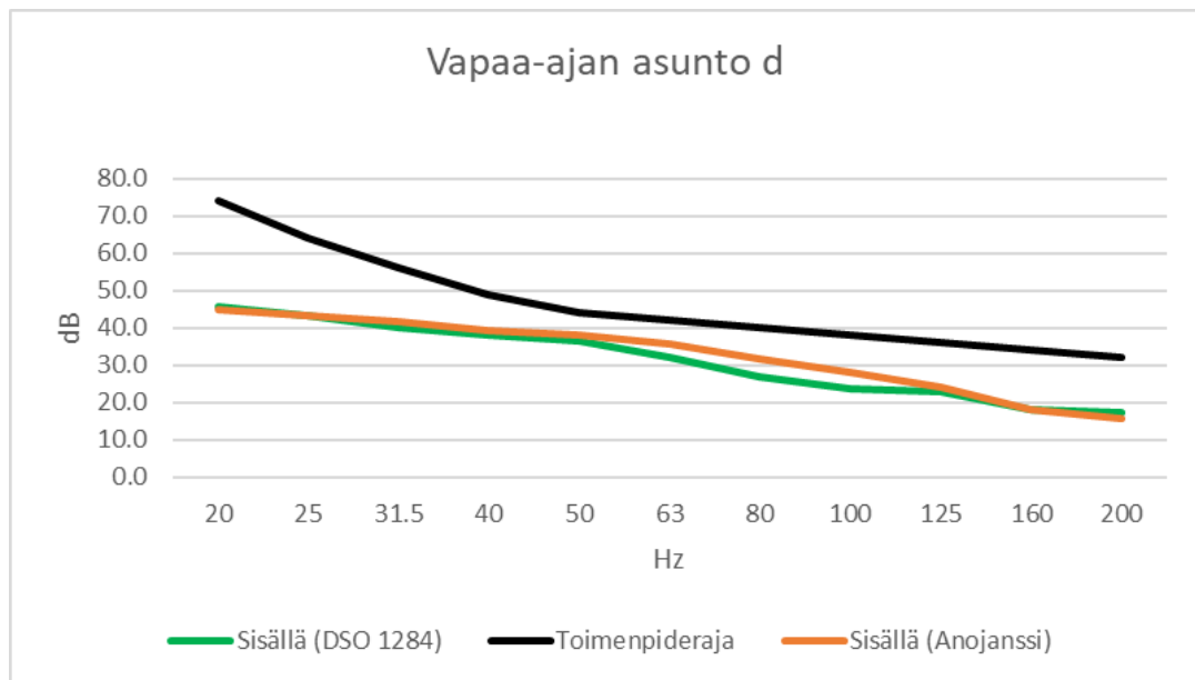
Kuva 8. Ympäristöministeriön ohjeistuksen mukainen pienitaajuisen melun laskenta sekä sosiaali- ja terveysministeriön toimenpiderajat vapaa-ajan asunnossa d.
