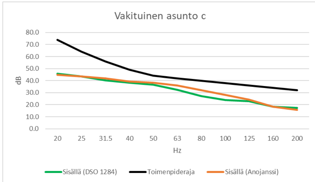
Kuva 7. Ympäristöministeriön ohjeistuksen mukainen pienitaajuisen melun laskenta sekä sosiaali- ja terveysministeriön toimenpiderajat vakituksessa asunnossa c.
