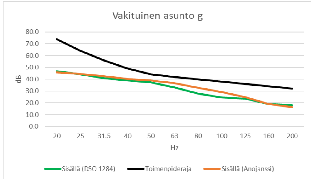
Kuva 9. Ympäristöministeriön ohjeistuksen mukainen pienitaajuisen melun laskenta sekä sosiaali- ja terveysministeriön toimenpiderajat vakituksessa asunnossa g.
