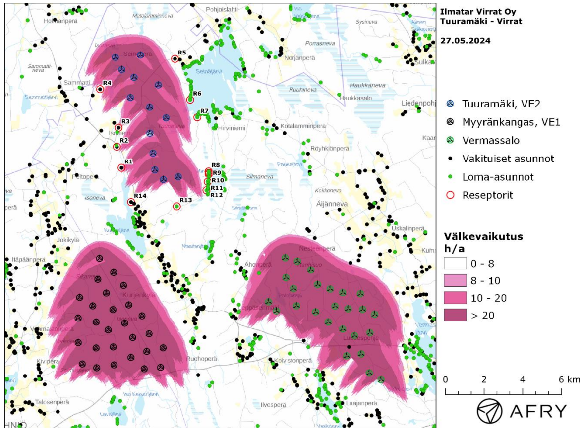
Kuva 6: Todennäköinen vuotuinen välkevaikutus, kun mallinuksissa huomioidaan Tuoramäen, Myyränkankaan VE1 ja Vermassalon tuulivoimapaistot.
