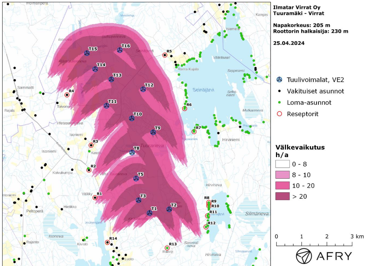
Kuva 4: Tuoramäen tuulivoimaloiden aiheuttama todennäköisen välkkeen määrä ilman puuston vaikutusta.
