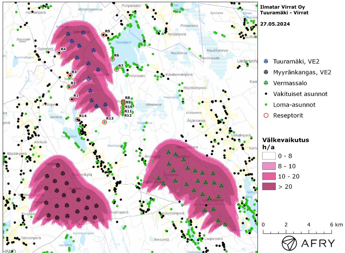
Kuva 7: Todennäköinen vuotuinen välkevaikutus, kun mallinnoissa huomioidaan Tuoramäen, Myyränkankaan VE2 ja Vermassalon tuulivoimapaistot.
