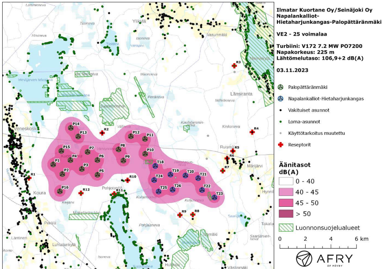
Kuva 6: Keskiäänitasot LAeq tuulivoimapuiston hankealueella toteutusvaihtoehdolla VE2.
