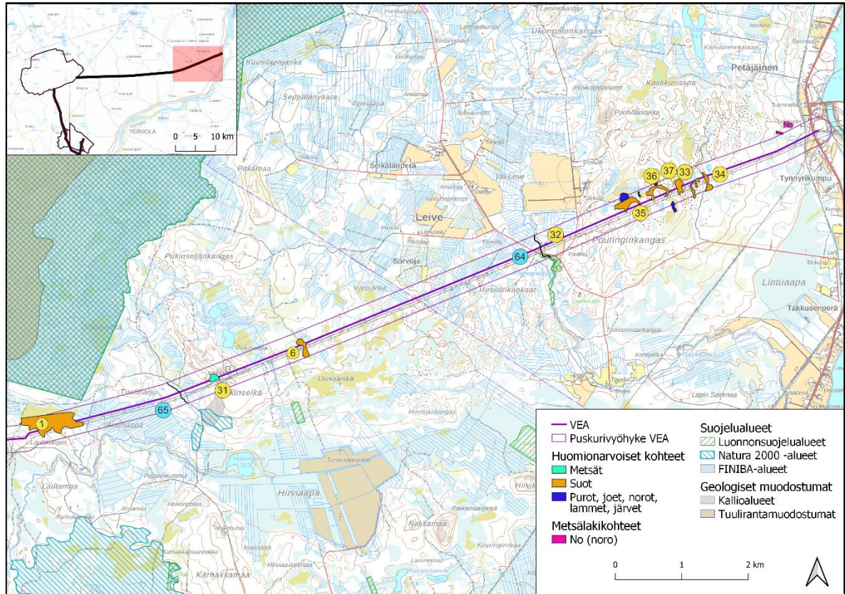
Kuva 13. Sähkönsiirtovaihtoehdon VEA (Martimo-Petäjäskoski) itäosan huomionarvoiset suo- ja metsäkohteet (numero keltaisella pohjalla viittaa alla olevien taulukoiden kohteisiin) sekä vesiläki-kohteet (numero sinisellä pohjalla viittaa taulukon 7 kohteisiin). Lisäksi kartalla näkyvät mahdolliset Metsäkeskuksen rajaamat metsälakikohteet sekä joet, lammet, järvet ja norot. Myös ympäristöhallinnon Oiva-aineistojen geologiset muodostumat ja erilaiset suojelualueet on esitetty kartalla.
