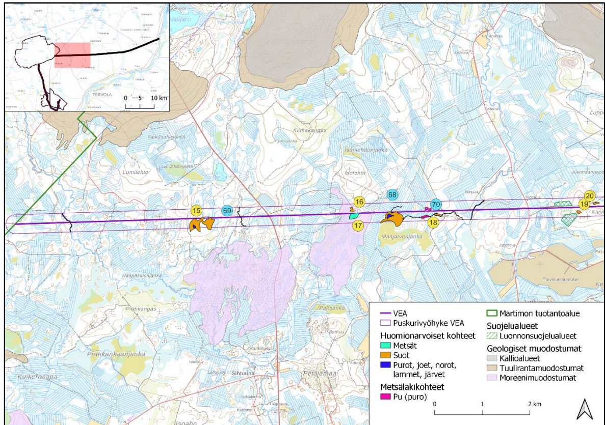
Kuva 5. Sähkösiirtovaihtoehtojen VEA (Martimo-Petäjäskoski) länsiosan huomionarvoiset suo- ja metsäkohteet (numero keltaisella pohjalla viittaa alla olevien taulukoiden kohteisiin) sekä vesiläki-kohteet (numero sinisellä pohjalla viittaa taulukon 7 kohteisiin). Lisäksi kartalla näkyvät mahdolliset Metsäkeskuksen rajaamat metsälakikohteet sekä joet, lammet, järvet ja norot. Myös ympäristöhallinnon Oiva-aineistojen geologiset muodostumat ja erilaiset suojelualueet on esitetty kartalla.
