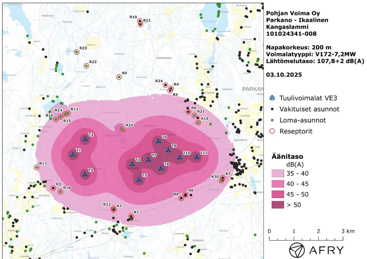
Kuva 3-2: Keskiäänitasot L_{Aeq} Kangaslammin toteutusvaihtoehdolla VE3.
