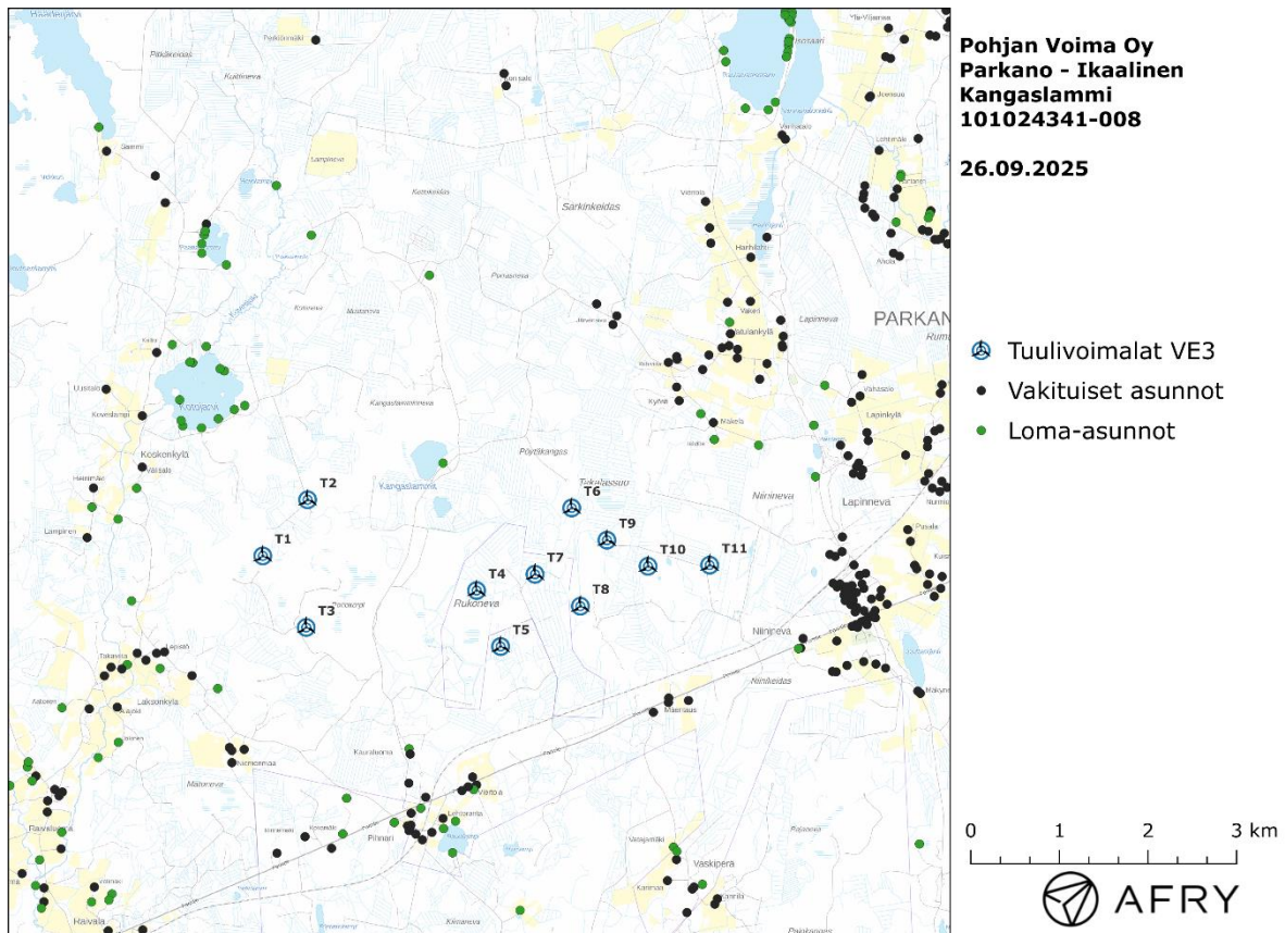
Kuva 1-1: Tuulivoimaloiden sijainnit Kangaslammin toteutusvaihtoehdolla VE3.
