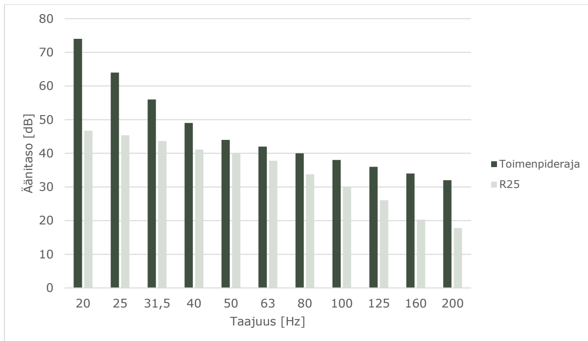
Kuva 3-3: Matalataajuisen sisämelun tasot reseptorin R25 kohdalla.
