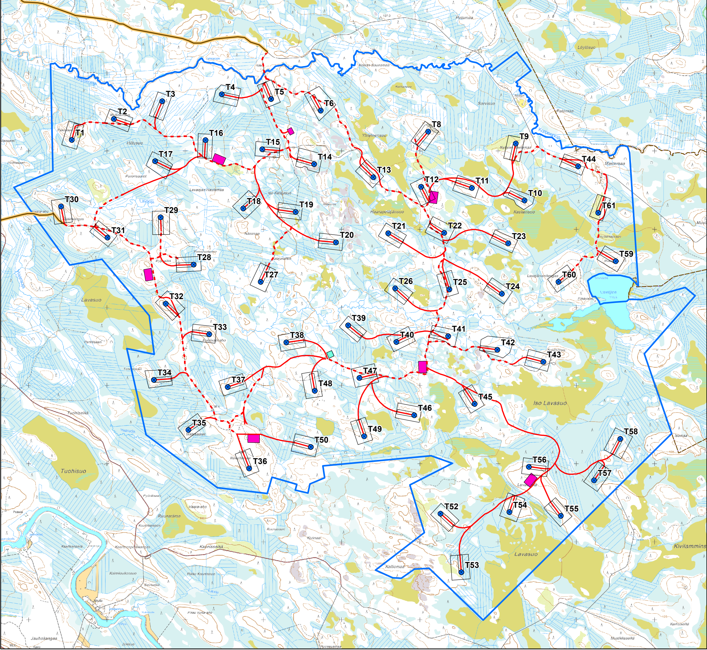
Hankevaihtoehto 1 mukainen tuulivoimaloiden sijoitussuunnitelma
