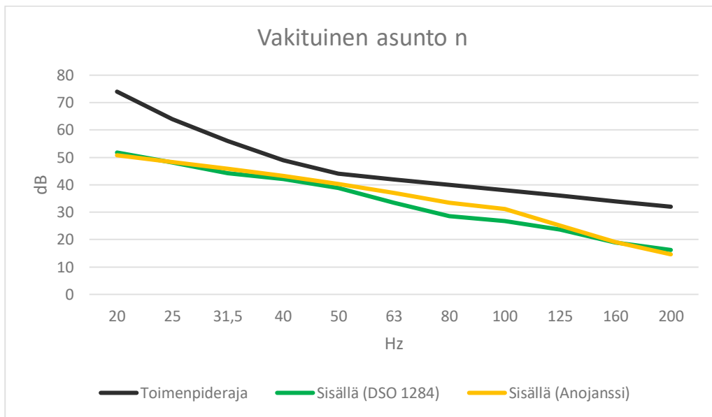
Kuva 7. Ympäristöministeriön ohjeistuksen mukainen pienitaajuisen melun laskenta sekä sosiaali- ja terveysministeriön toimenpiderajat vakituksessa asunnossa n.
