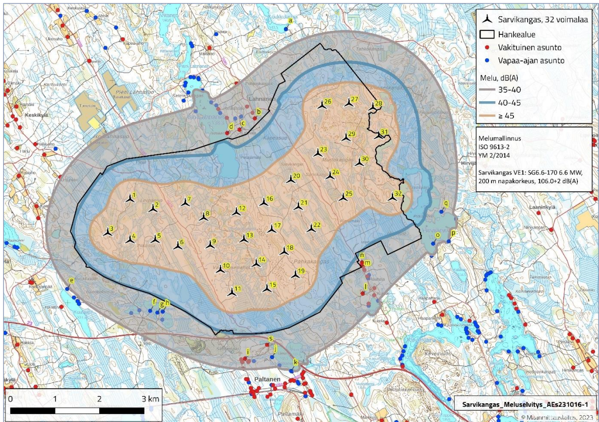
Kuva 1. Sarvikankaan tuulivoimapuiston melumallinnus (VE1). 19 havainnointipistettä on merkitty kuvaan kirjaimilla (a-s).
