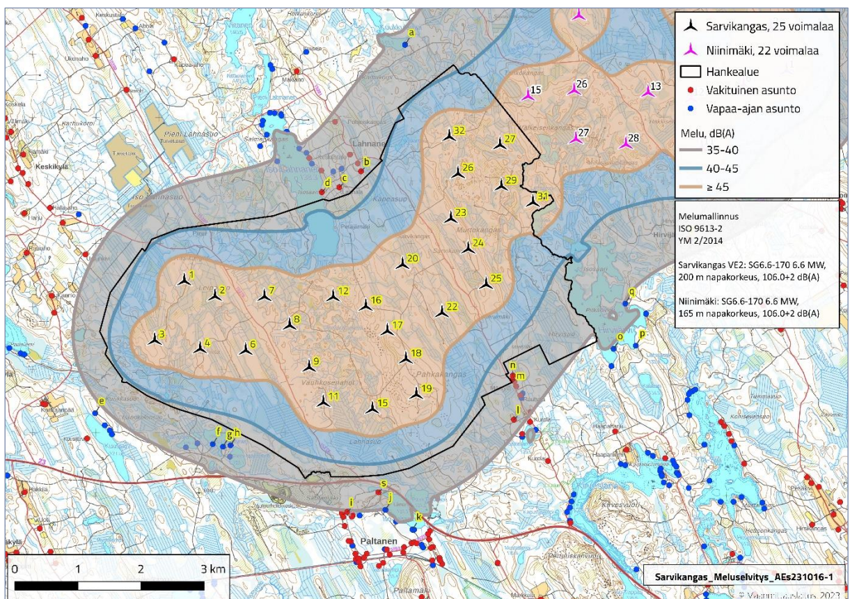
Kuva 4. Sarvikankaan tuulivoimapaiston (VE2) ja naapuripuisto Niinimäen yhteisvaikutusten melumallinnus. 19 havainnointipistettä on merkitty kuvaan kirjaimilla (a-s).
