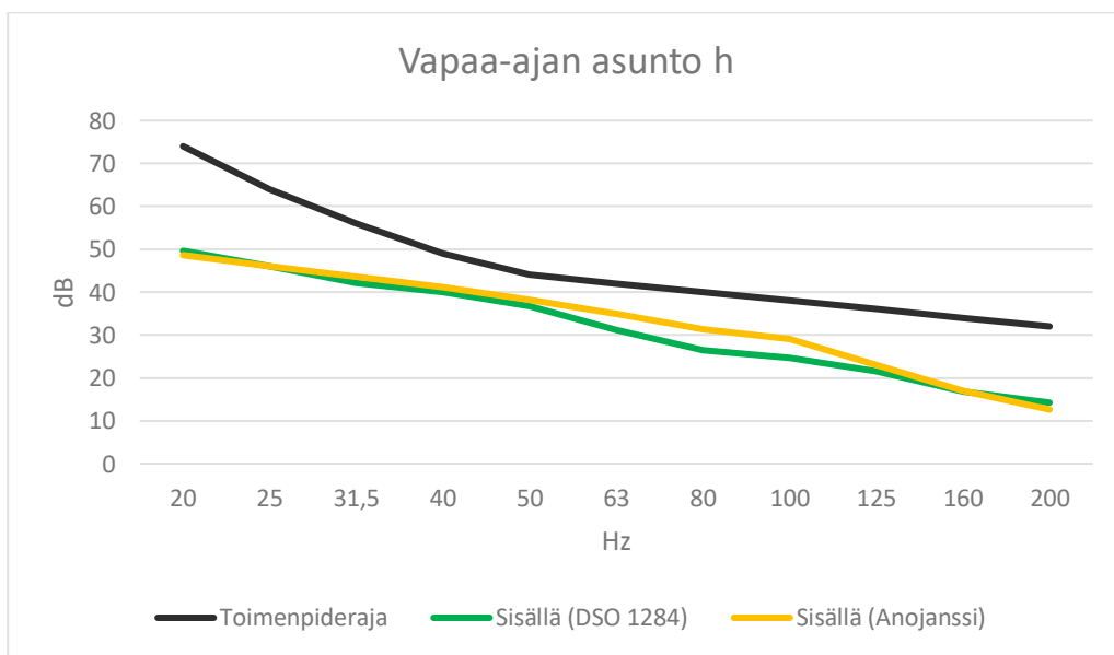
Kuva 10. Ympäristöministeriön ohjeistuksen mukainen pienitaajuisen melun laskenta sekä sosiaali- ja terveysministeriön toimenpiderajat vapaa-ajan asunnossa h.
