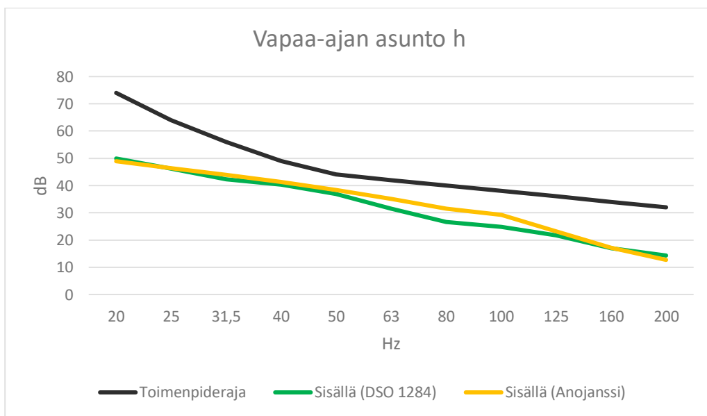
Kuva 12. Ympäristöministeriön ohjeistuksen mukainen pienitaajuisen melun laskenta sekä sosiaali- ja terveysministeriön toimenpiderajat vapaa-ajan asunnossa h.
