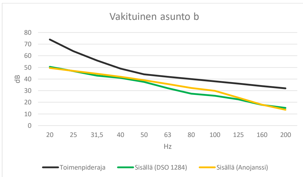
Kuva 9. Ympäristöministeriön ohjeistuksen mukainen pienitaajuisen melun laskenta sekä sosiaali- ja terveysministeriön toimenpiderajat vakituksessa asunnossa b.
