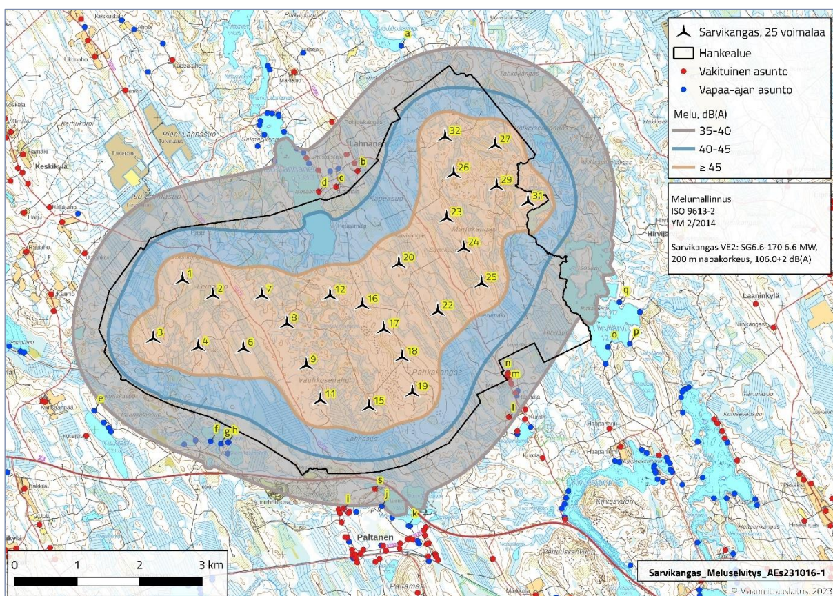
Kuva 3. Sarvikankaan tuulivoimapuiston melumallinnus (VE2). 19 havainnointipistettä on merkitty kuvaan kirjaimilla (a-s).
