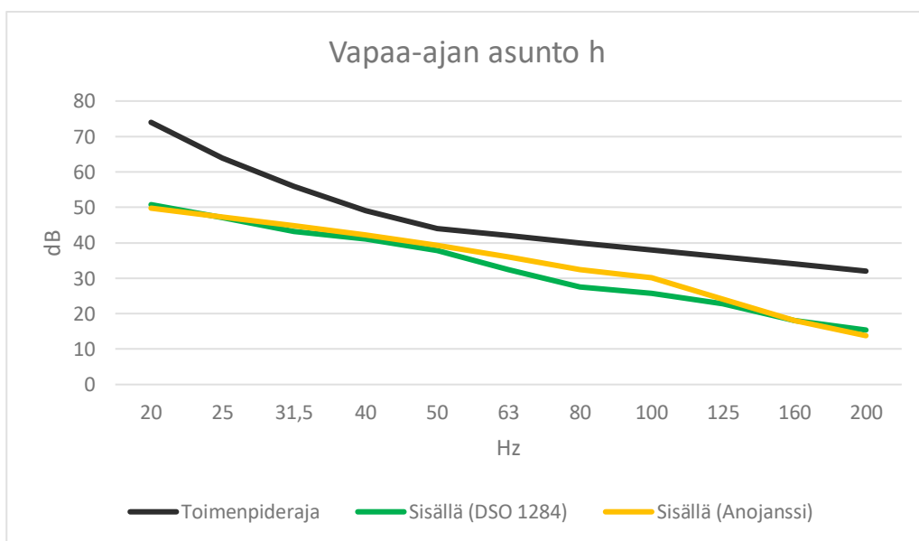
Kuva 6. Ympäristöministeriön ohjeistuksen mukainen pienitaajuisen melun laskenta sekä sosiaali- ja terveysministeriön toimenpiderajat vapaa-ajan asunnossa h.
