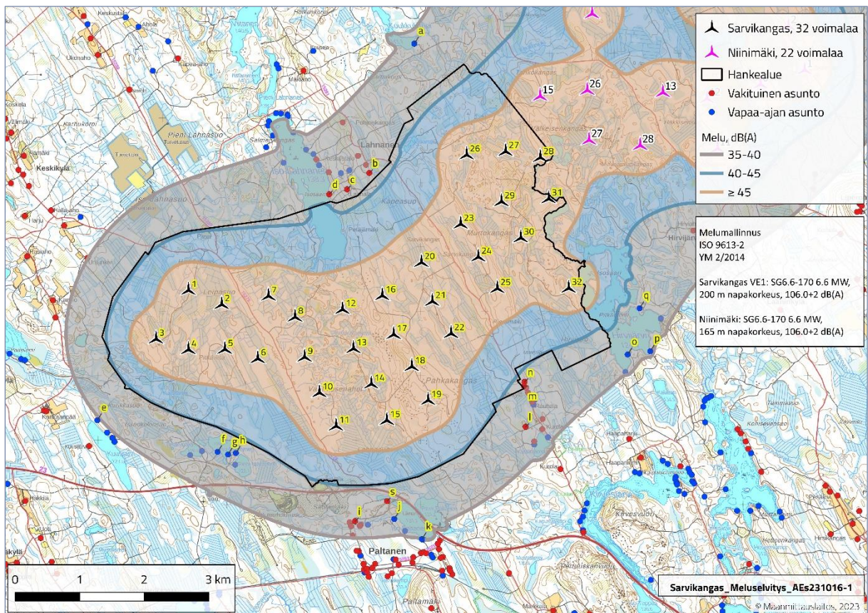
Kuva 2. Sarvikankaan tuulivoimapuiston (VE1) ja naapuripuisto Niinimäen yhteisvaikutusten melumallinnus. 19 havainnointipistettä on merkitty kuvaan kirjaimilla (a-s).
