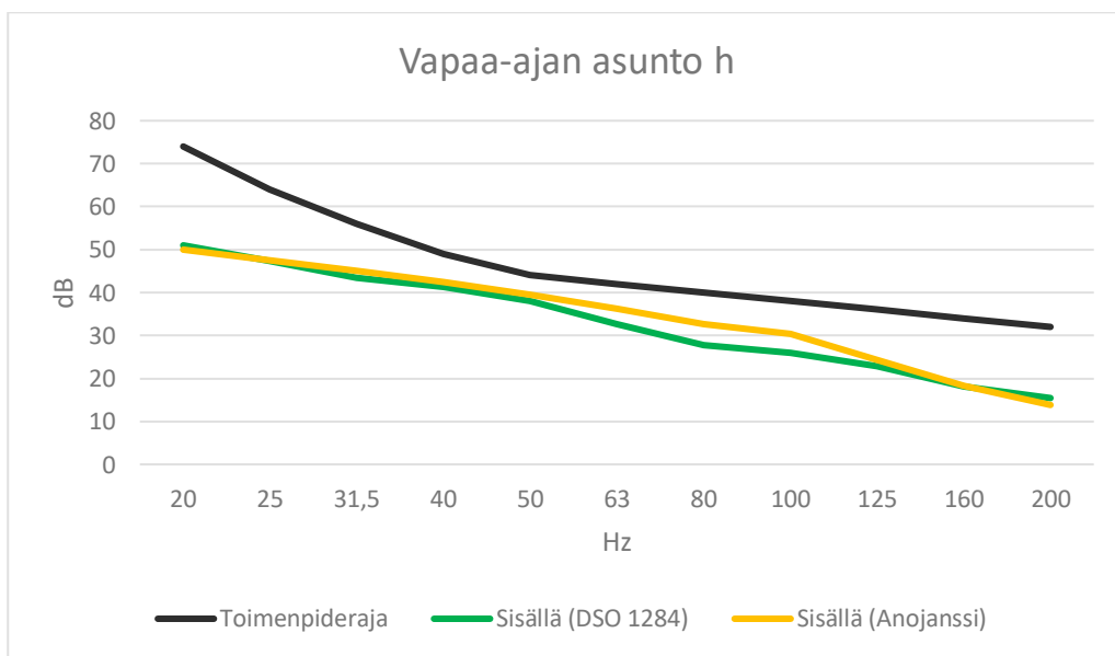
Kuva 8. Ympäristöministeriön ohjeistuksen mukainen pienitaajuisen melun laskenta sekä sosiaali- ja terveysministeriön toimenpiderajat vapaa-ajan asunnossa h.
