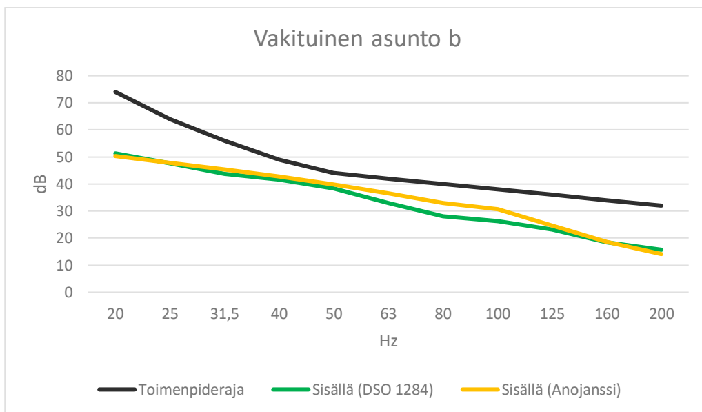
Kuva 11. Ympäristöministeriön ohjeistuksen mukainen pienitaajuisen melun laskenta sekä sosiaali- ja terveysministeriön toimenpiderajat vakituksessa asunnossa b.
