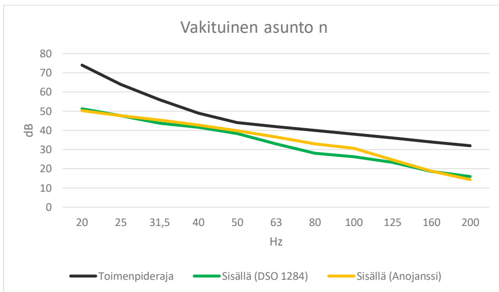
Kuva 5. Ympäristöministeriön ohjeistuksen mukainen pienitaajuisen melun laskenta sekä sosiaali- ja terveysministeriön toimenpiderajat vakituksessa asunnossa n.
