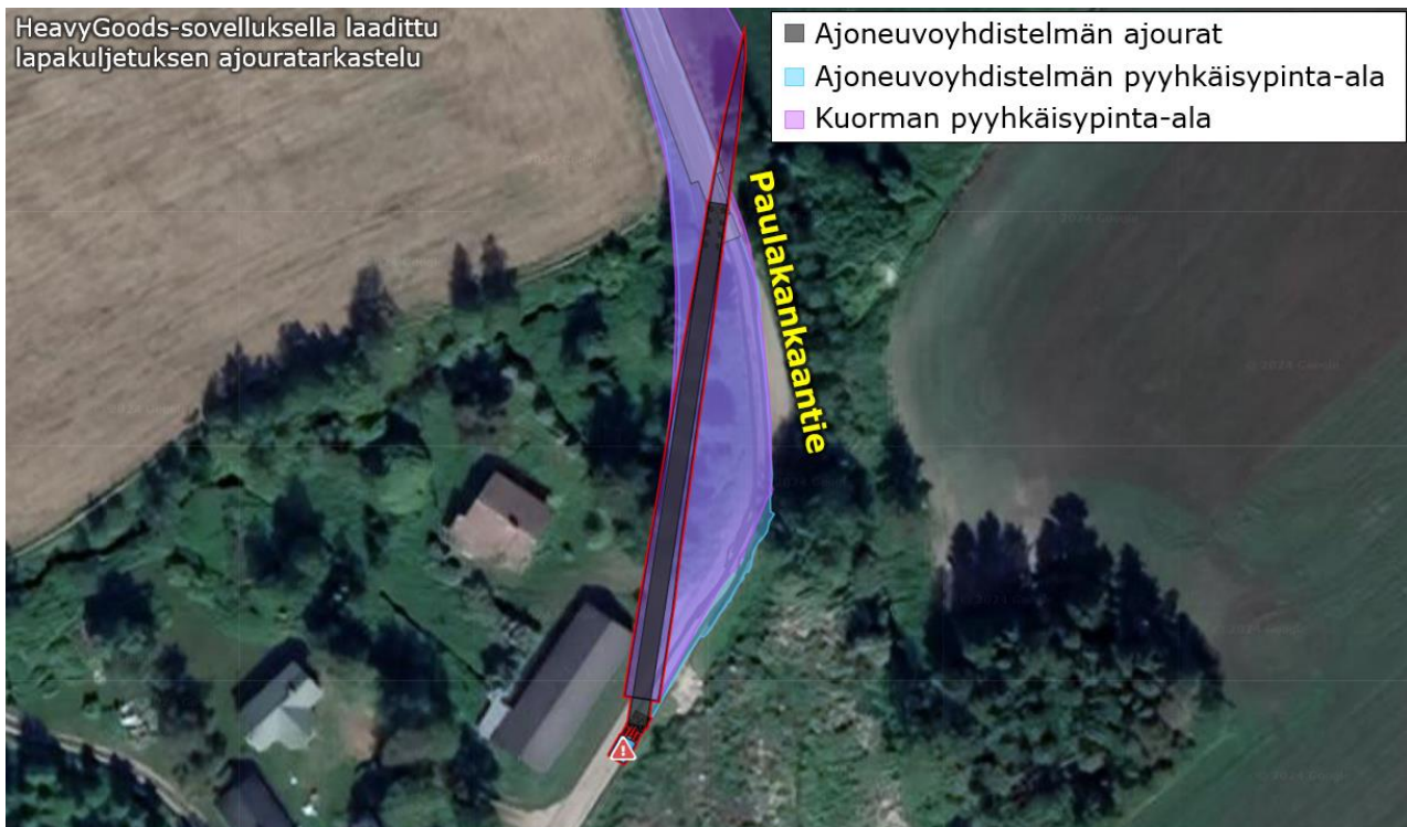
Kuva 13: Havainnollistava kuva lapakuljetuksen tilantarpeesta Paulakankaantiellä olevassa mutkassa. Nykyinen tielinjaus kulkee lapakuljetuksen kääntymisen kannalta liian läheltä tien länsipuolella sijaitseva rakennusta.
