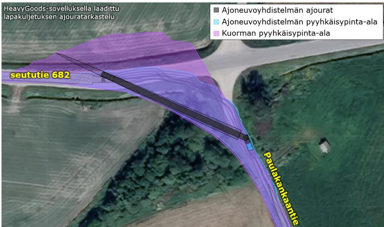
Kuva 10: Havainnollistava kuva lapakuljetuksen tilantarpeesta seututien 682 ja Paulakankaantien liittymässä.
