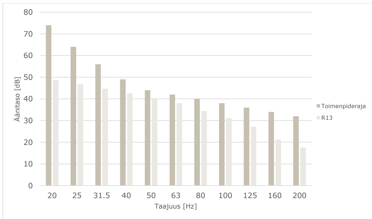
Kuva 7: Matalataajuisen sisämelun tasot reseptorin R13 kohdalla, kun mallinuksissa huomioidaan Tielammen suunnitelma VE2 sekä Iso-Petäjämäen voimalat.
