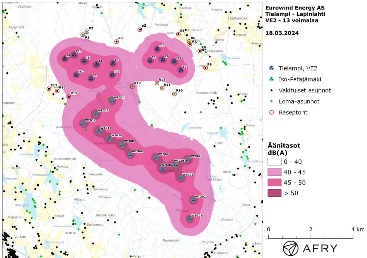
Kuva 6: Keskiäänitasot LAeq, kun mallinuksissa huomioidaan Tielammen suunnitelma VE2 ja Iso-Petäjämäen voimalat.
