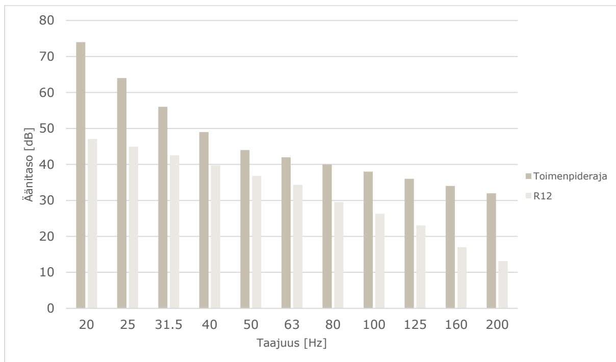
Kuva 5: Matalataajuisen sisämelun tasot reseptorin R12 kohdalla.
