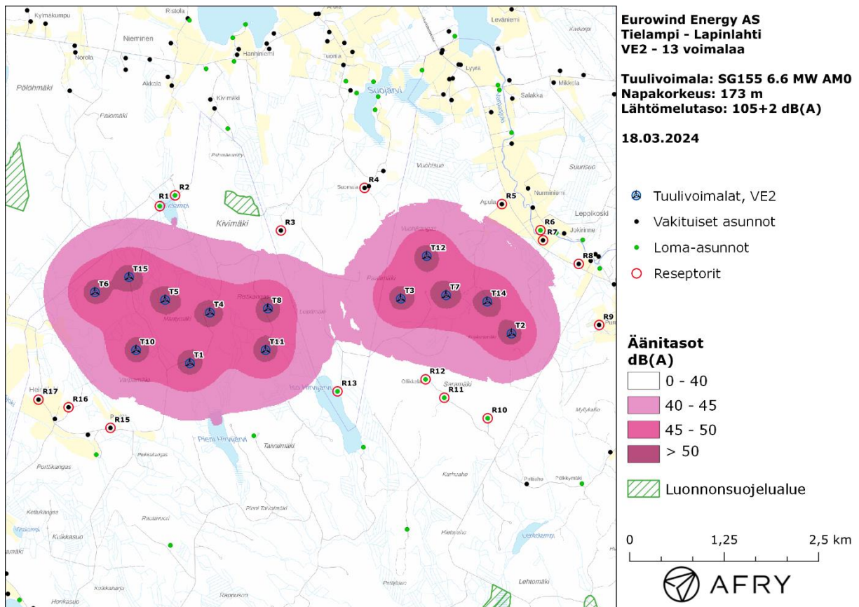
Kuva 4: Keskiäänitasot L_{Aeq} Tielammen tuulivoimapuiston hankealueella.
