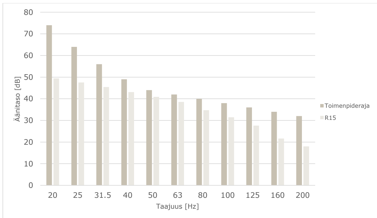
Kuva 7: Matalataajuuden sisämelun tasot reseptorin R15 kohdalla, kun mallinuksissa huomioidaan Tielammen suunnitelma VE1 sekä Iso-Petäjämäen voimalat.
