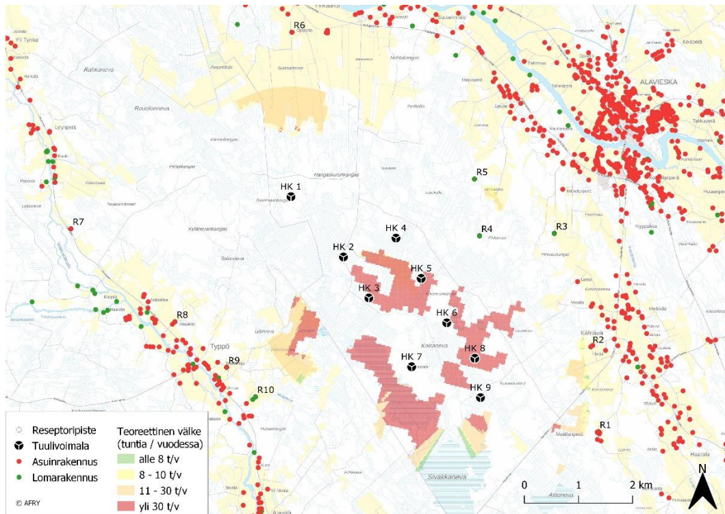
Kuva 4-1. Välkkeen teoreettinen määrä tunteina vuodessa (aurionpaistehavaintoja ei ole huomioitu) Hangaskurunkankaan yhdeksän voimalan sijoitussuunnitelmalla, kun puuston vähentävä vaikutus on huomioitu. Mallinnus on tehty tuulivoimaloilla, joiden napakorkeus on 200 m ja roottorin halkaisija 200 m.
