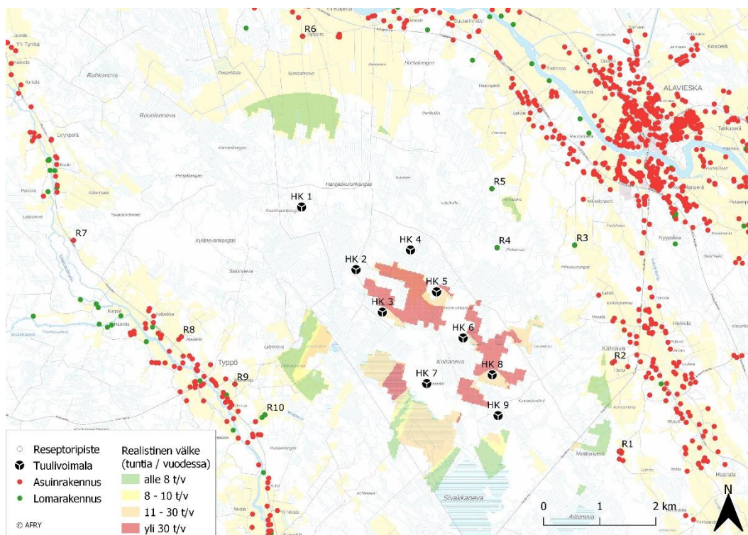
Kuva 4-2. Väikkeen realistinen määrä tunteina vuodessa (aurionpaistehavainnot on huomioitu) Hangaskurunkankaan yhdeksän voimalan sijoitussuunnitelmalla, kun puuston vähentävä vaikutus on huomioitu. Mallinnus on tehty tuulivoimaloilla, joiden napakorkeus on 200 m ja roottorin halkaisija 200 m.
