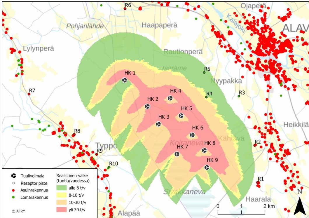
Kuva 3-2. Välkkeen realistinen määrä tunteina vuodessa (aurionpaistehavainnot otettu huomioon) Hangaskurunkankaan yhdeksän voimalan sijoitusuunnitelmalla. Mallinnus on tehty tuulivoimaloilla, joiden napakorkeus on 200 m ja roottorin halkaisija 200 m.
