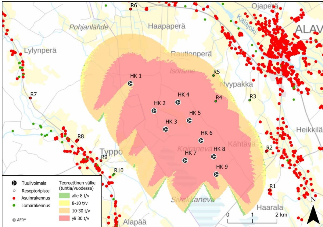
Kuva 3-1. Välkkeen teoreettinen määrä tunteina vuodessa (aurionpaistehavaintoja ei ole huomioitu) Hangaskurunkankaan yhdeksän voimalan sijoitus suunnitelmalla. Mallinnus on tehty tuulivoimaloilla, joiden napakorkeus on 200 m ja roottorin halkaisija 200 m.
