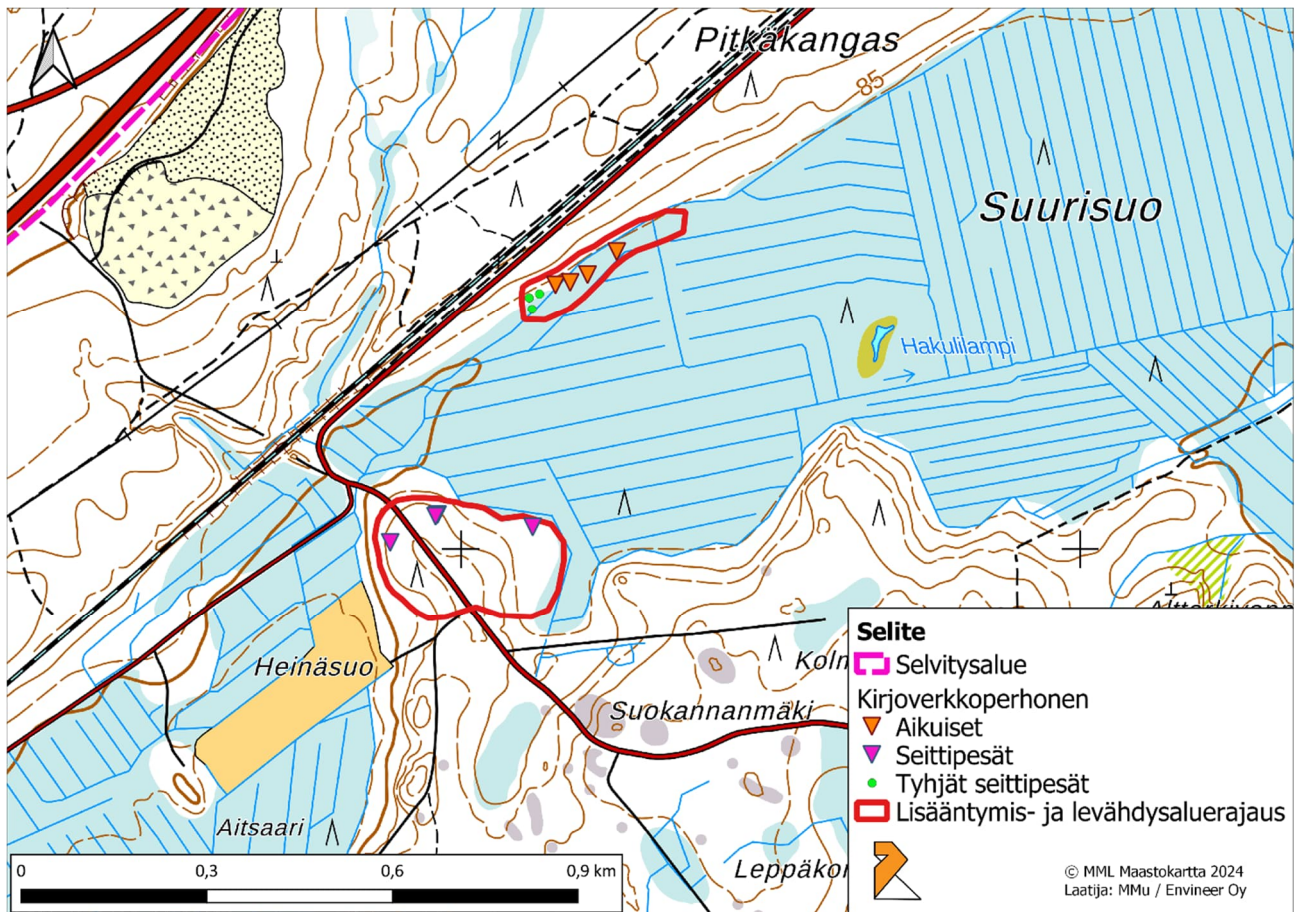
Kuva 18. Havaitut aikuiset (21.6.2023) kirjoverkkoperhosen, seittipesät (31.8.2023) sekä lisääntymis- ja levähdysalueen rajaus. Keskimmäisen asutun seittipesähavainnon kohdalla on kaksi erillistä pesää.
