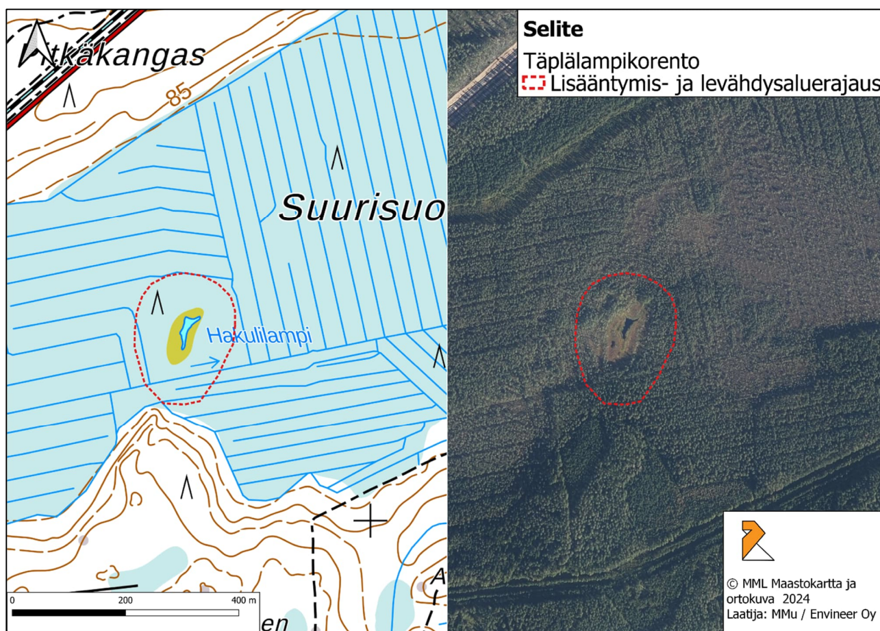
Kuva 22. Täplälampikorenon lisääntymis- ja levähdysaluearajaus maastokartta- ja ortokuvapohjalla.
