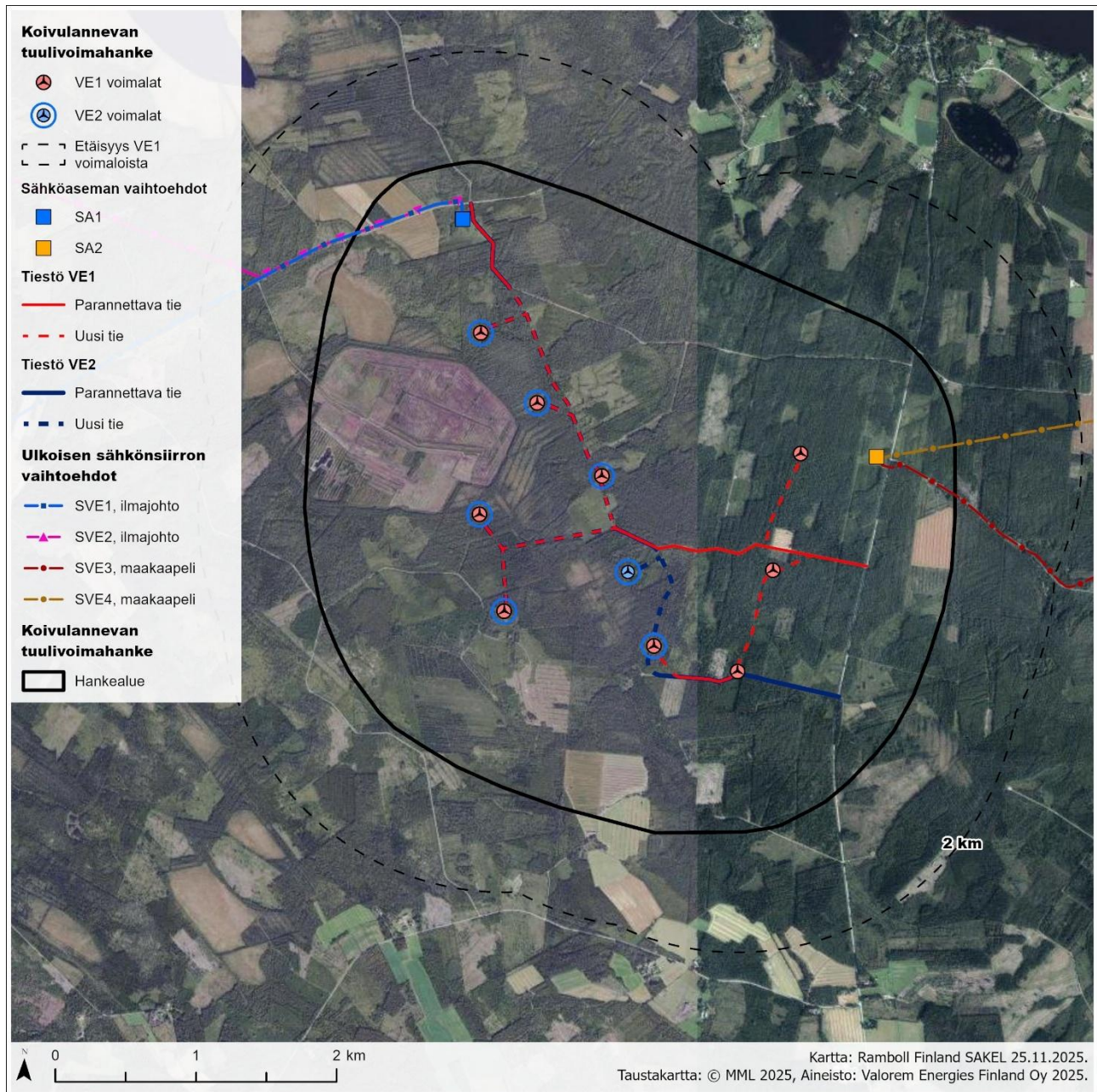
Kuva 2-4. Hankealueen raja, voimaloiden sijoitus suunnitelma ja huoltotiestö vaihtoehdoissa VE1 ja VE2, sekä sisäisen sähköaseman vaihtoehdot SA1 ja SA2 ilmakuvalla.
