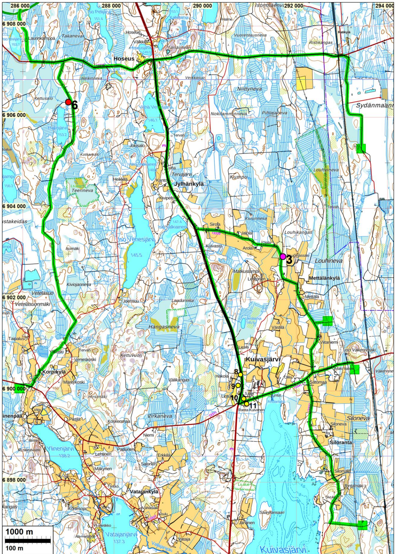
Vaihtoehtoiset maakaapelilinjat vihreällä ja niiden päihin rakennettavat sähköasemat neliöin.
