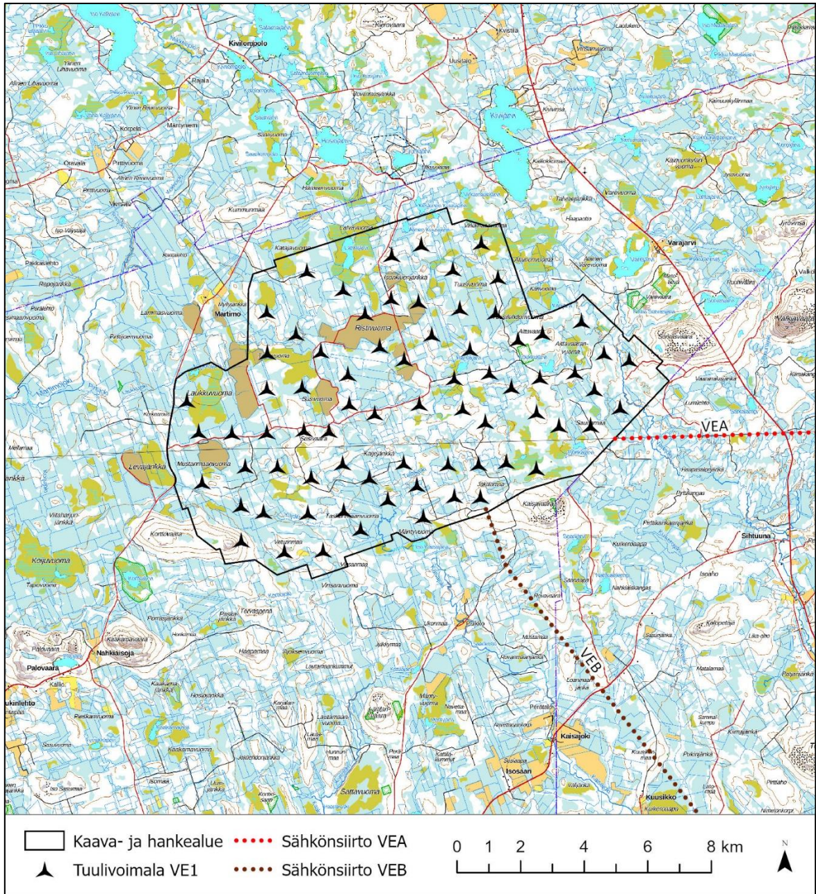
Kuva 2.1. Kaava- ja hankealueen rajaus. Kuvassa on esitetty alustava voimaloiden sijoittelu ja voimajohtoreittivaihtoehdot.
