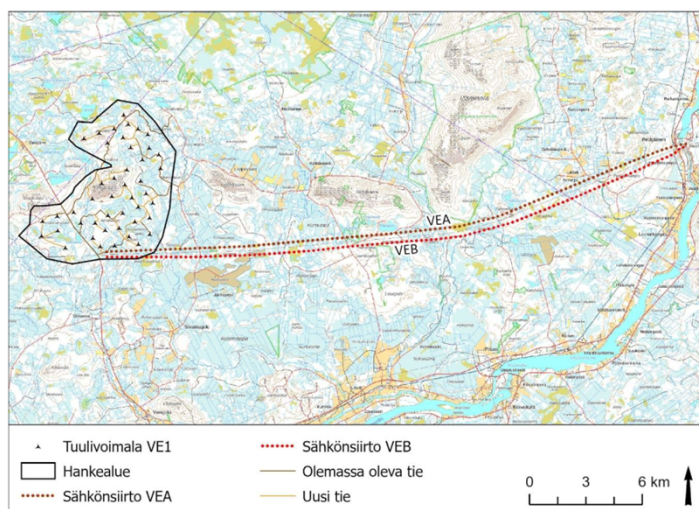
Kuva 1. Sähkönsiirron vaihtoehdot (lähde: yva-ohjelma).
