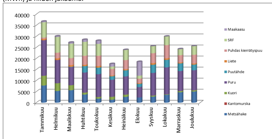
Kuva 1. Hämeenkyrön Voima Oy:n voimalaitoksen vuonna 2024 käyttämät polttoaineet (MWh) ja niiden jakauma.
