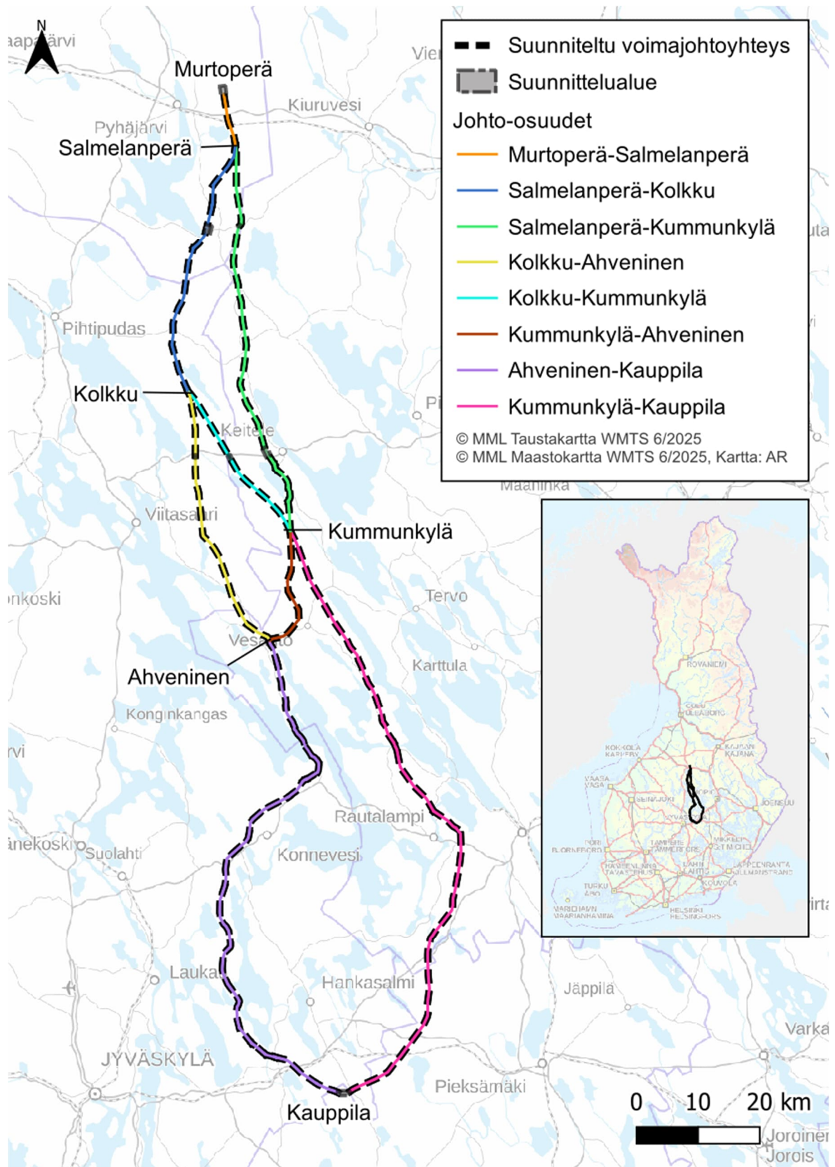
Kuva 1. Suunnitellut voimajohtoyhteysvaihtoehdot Murtoperän ja Kauppilan välillä.
