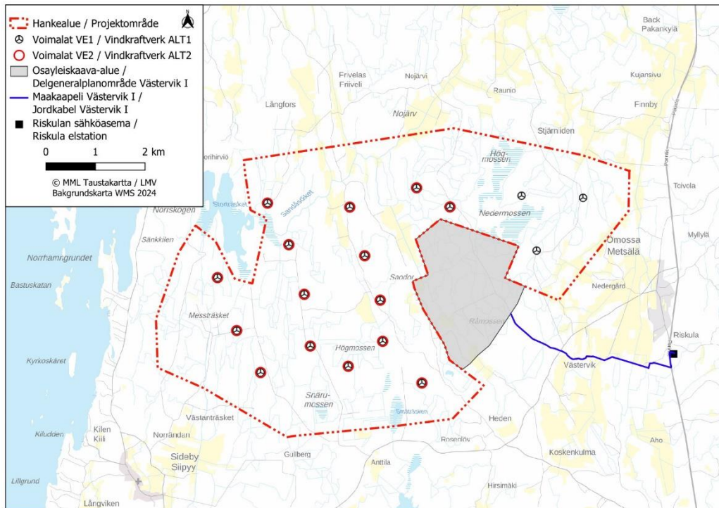
Kuva 1. YVA-menettelyssä tarkasteltavat vaihtoehdot VE1 ja VE2 sekä hankkeeseen suunniteltu sähkönsiirto.
