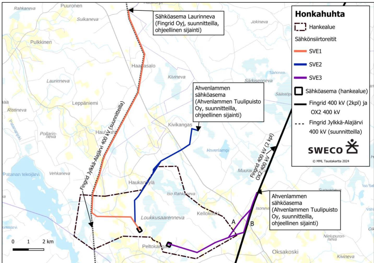
Kuva 2. Hankkeessa suunnitellut sähkönsiirron reittivaihtoehdot.
