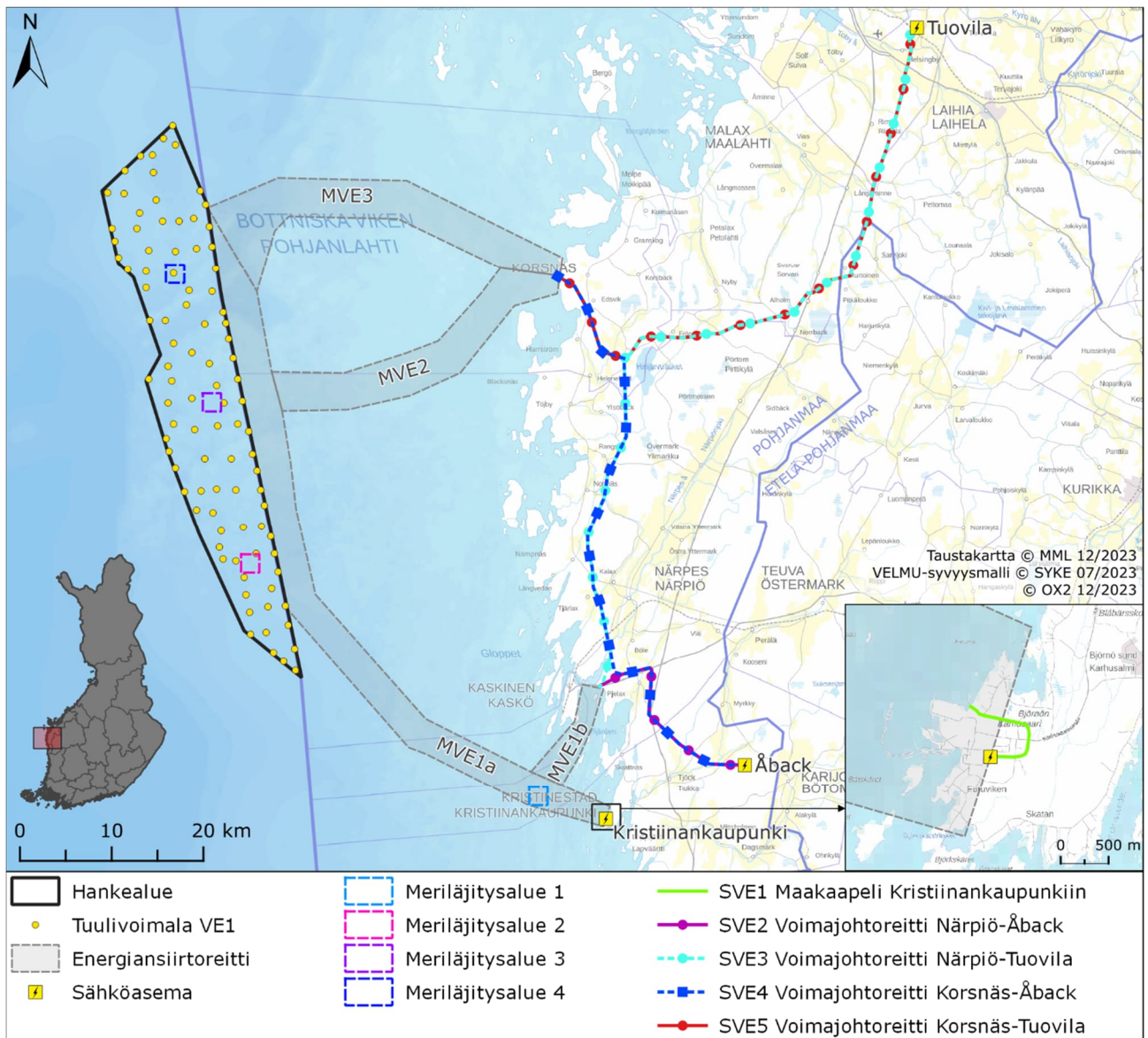
Kuva 1. Tyrsken merituulivoimapaiston hankealue (VE1, 95 voimalaa), potentiaaliset meriläjitäysalueet ja merikaapeleiden/vetypuutkien tutkimuskäytävät MVE1a, MVE1b, MVE2 ja MVE3 sekä sähkönsiirtoreitit mantereella (lähde: OX2 Finland Oy, Tyrsken merituulivoimapaiston YVA-ohjelma).
