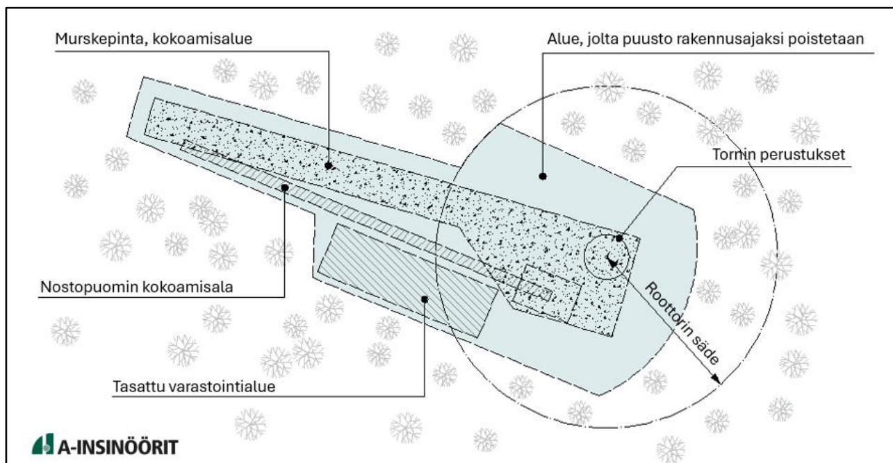
Kuva 16. Tyypillinen tuulivoimalan kokoamis- ja pystytysalue. (A-Insinöörit)
