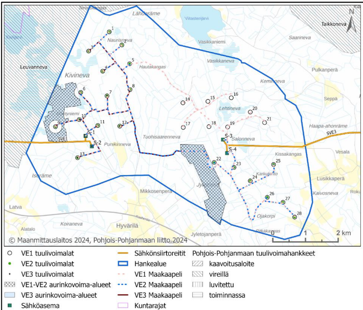
Kuva 27. Hankealueelle suunnitellut maakaapelit. VE2 maakaapelin hankealueen keskiosan itä-länsilinja sijoittuu noin 30 m olemassa olevan voimajohtolinjan pohjoispuolelle. Lukuun ottamatta tätä osuutta, kaikki maakaapelit on suunniteltu sijoittumaan uusien tai olemassa olevien teiden luiskaan. Kartalla ei ole teitä luettavuuden parantamiseksi.
