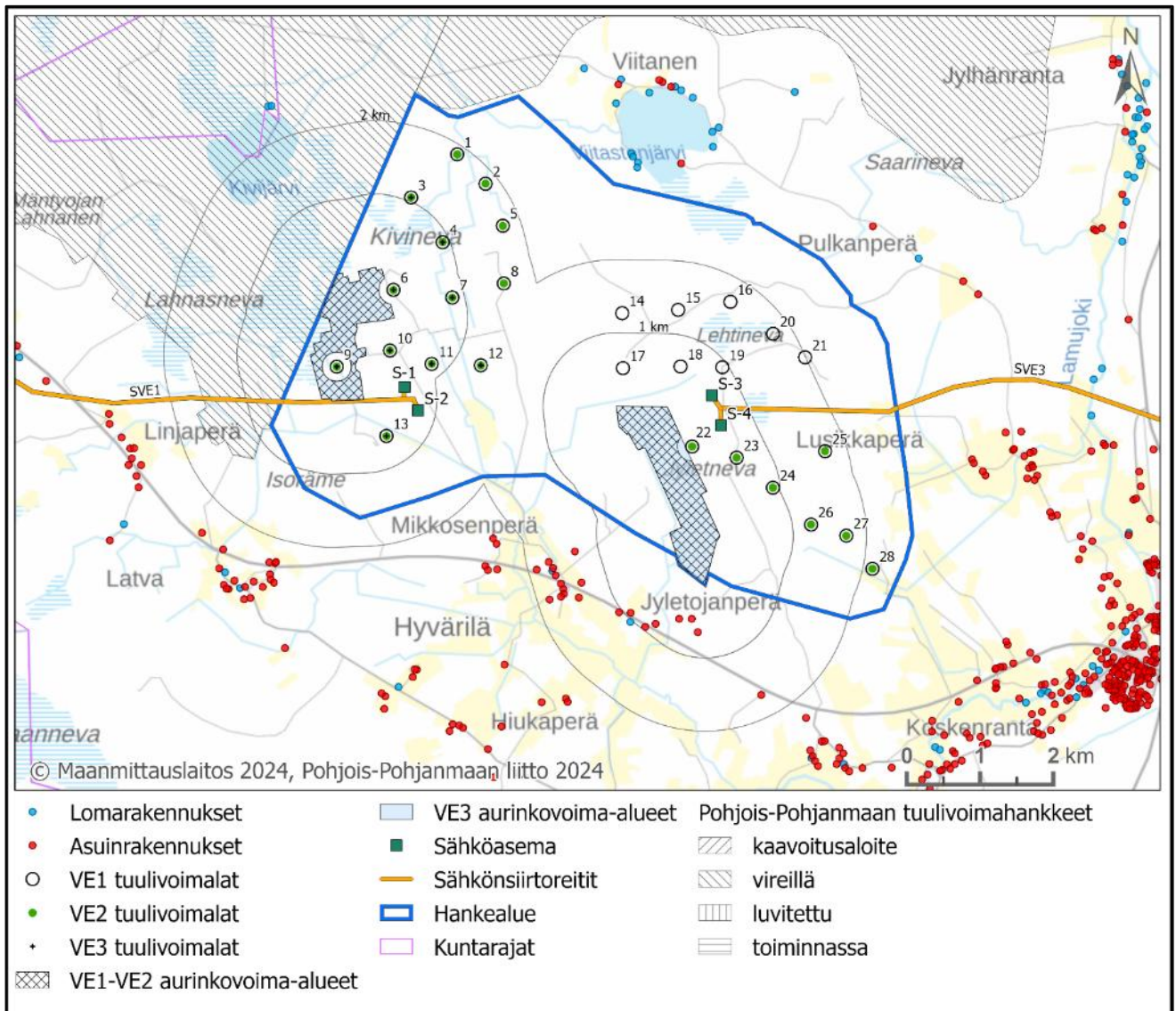
Kuva 155. Asuin- ja lomarakennusten sijoittuminen hankealueen ympäristössä pienempimittakaavaisella kartalla esitettynä. Kartalla on esitetty etäisyysvyöhykkeet aurinkovoimaloista suurimman aurinkovoimavaihto-ehdon VE3 mukaisesti. Asuin- ja vapaa-ajan rakennuksia on yhtä paljon VE1-VE3 etäisyysvyöhykkeillä kuin VE3 etäisyysvyöhykkeillä.
