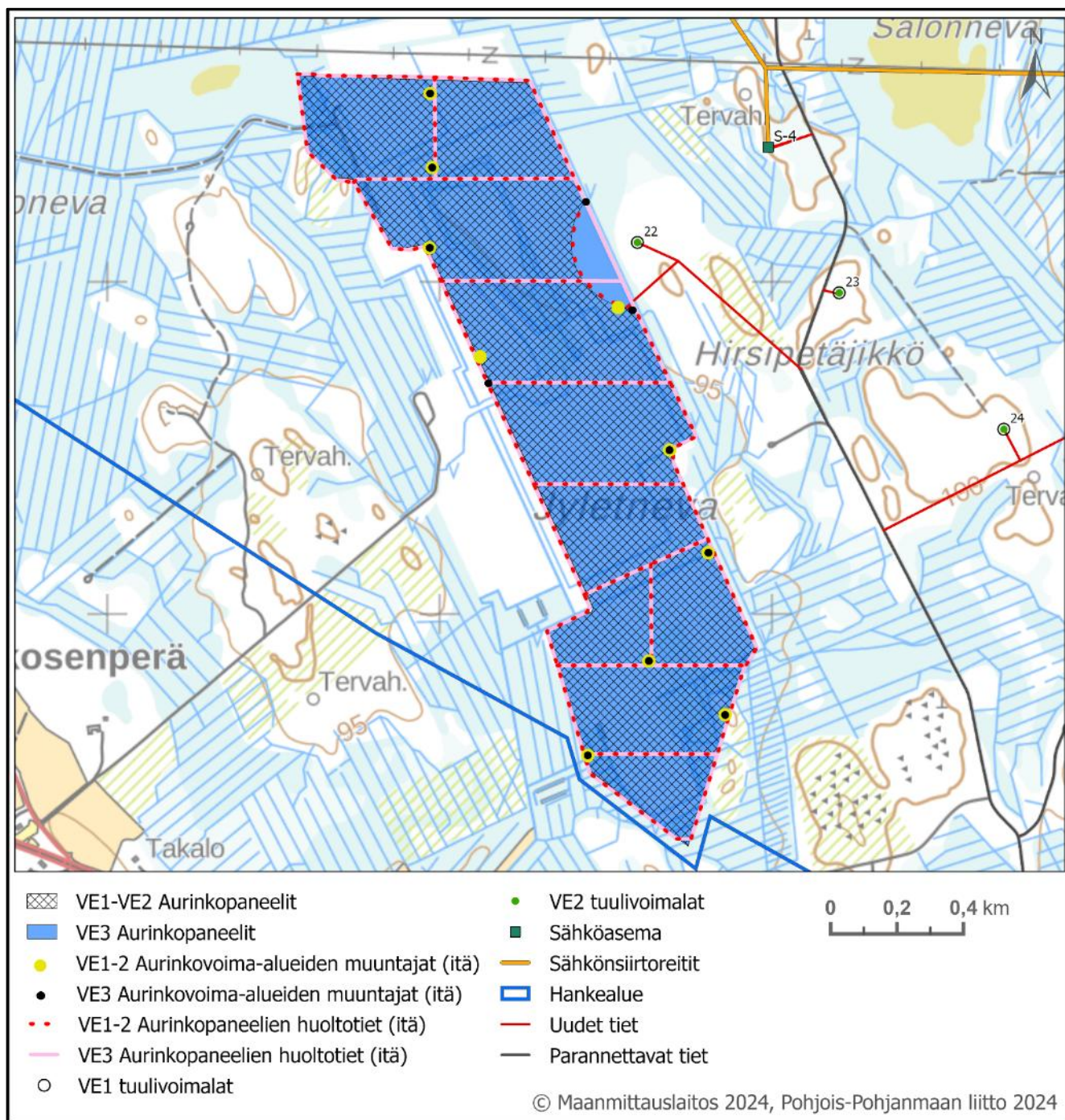
Kuva 24. Itäinen aurinkopaneelialue, sen huoltotiet ja muuntajat alueella. Vaihtoehtoisissa VE1-VE2 tuulivoimala 22 pienentää aurinkopaneeleille käytettävissä olevaa aluetta.
