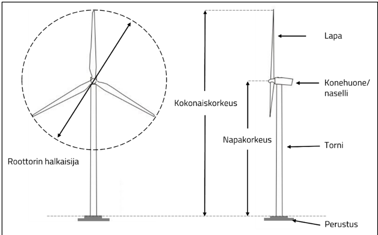
Kuva 12. Tuulivoimalan perusrakenne ja sen osat (Etha 2023).
