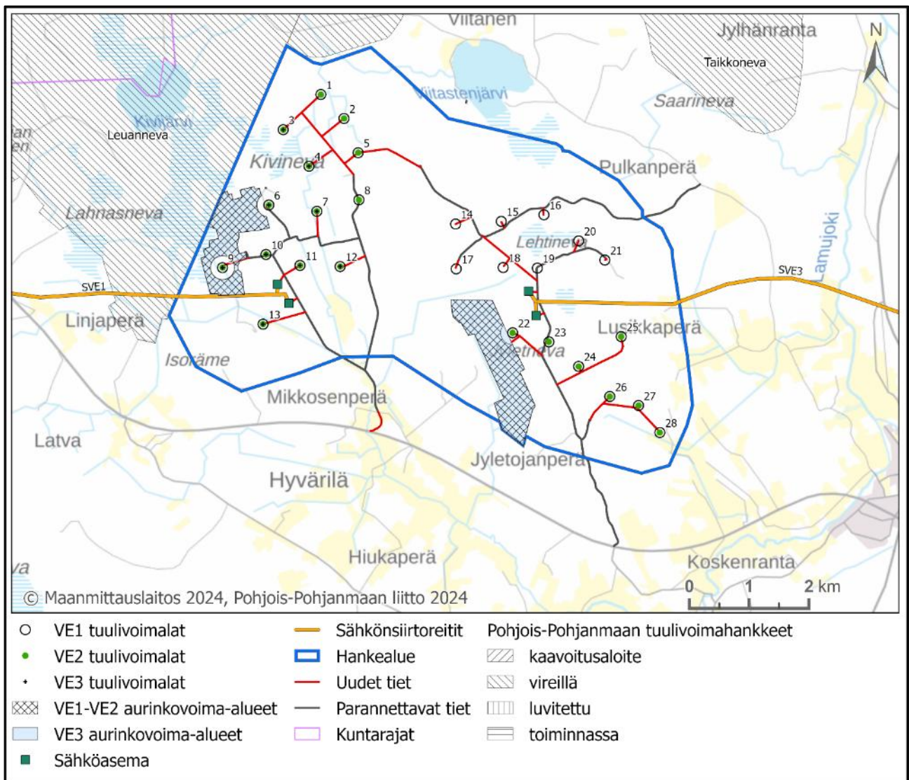
Kuva 116. Hankealue, sähkönsiirtoreitti, tuuli- ja aurinkovoimasijainnit sekä alueen uudet ja levennettävät tiet.
