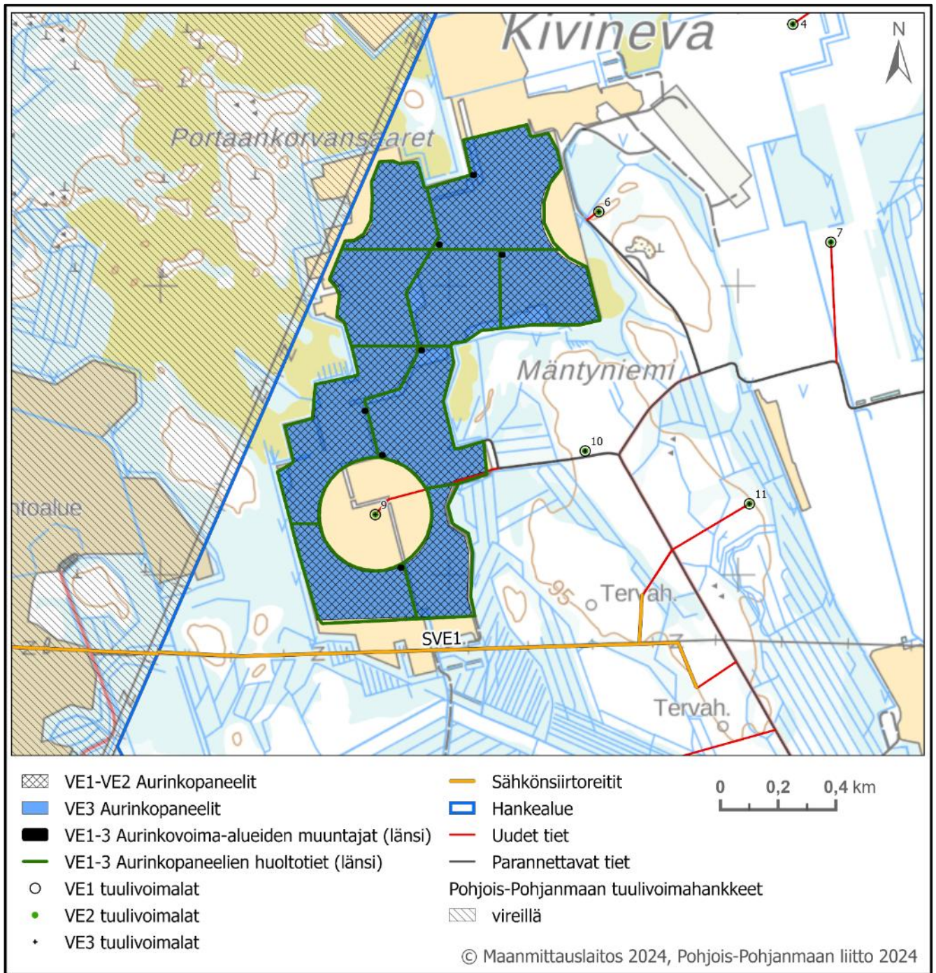
Kuva 23. Läntinen aurinkopaneelialue, sen huoltotiet ja muuntajat. Vaihtoehtojen välillä ei ole eroa.
