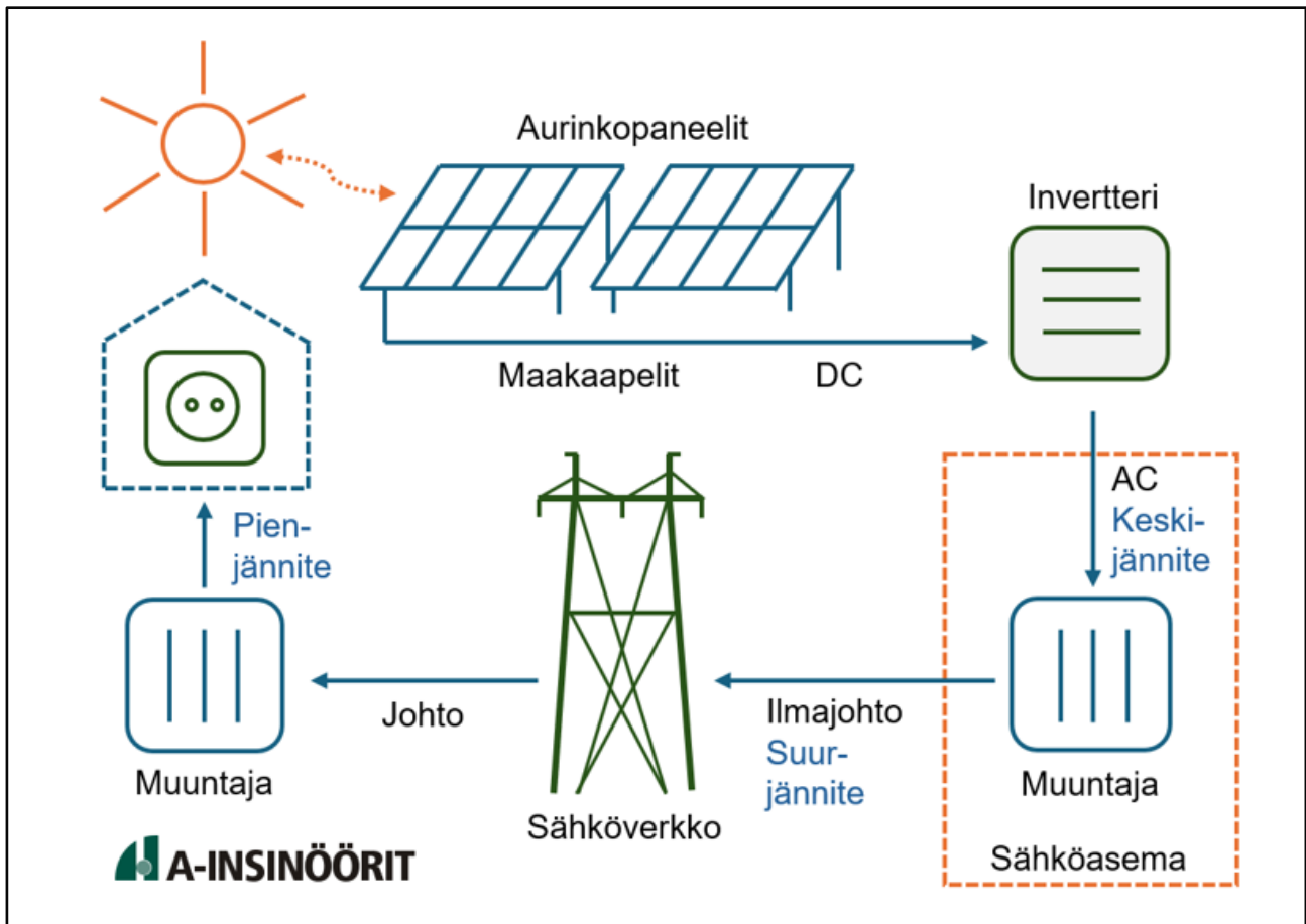
Kuva 18. Periaatekuva aurinkopaneelien vaatimista sähkönsiirtorakenteista.
