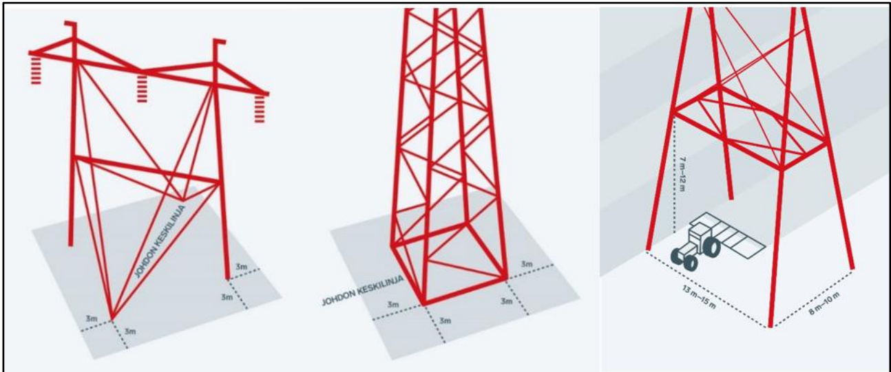
Kuva 36. Periaatekuva pylväsalaista. Vasemmassa kuvassa on harustettu kaksijalkainen portaaliypyläs, keskellä vaapaasti seisova pylväs ja oikealla peltopylväs (Lähde: Fingrid 2020).
