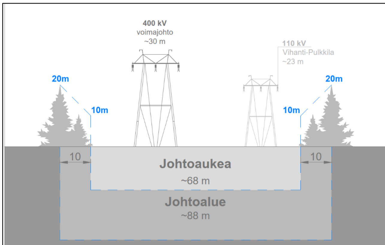
Kuva 33. Periaatekuva johtoalueesta, kun 400 kV voimajohto sijoitetaan olemassa olevan Vihanti-Pulkkila 110 kV voimajohtolinjan viereen. Johtoaukean molemmilla puolilla sijaitsee 10 metrin levyinen reunavyöhyke, jossa puuston kasvua rajoitetaan.
