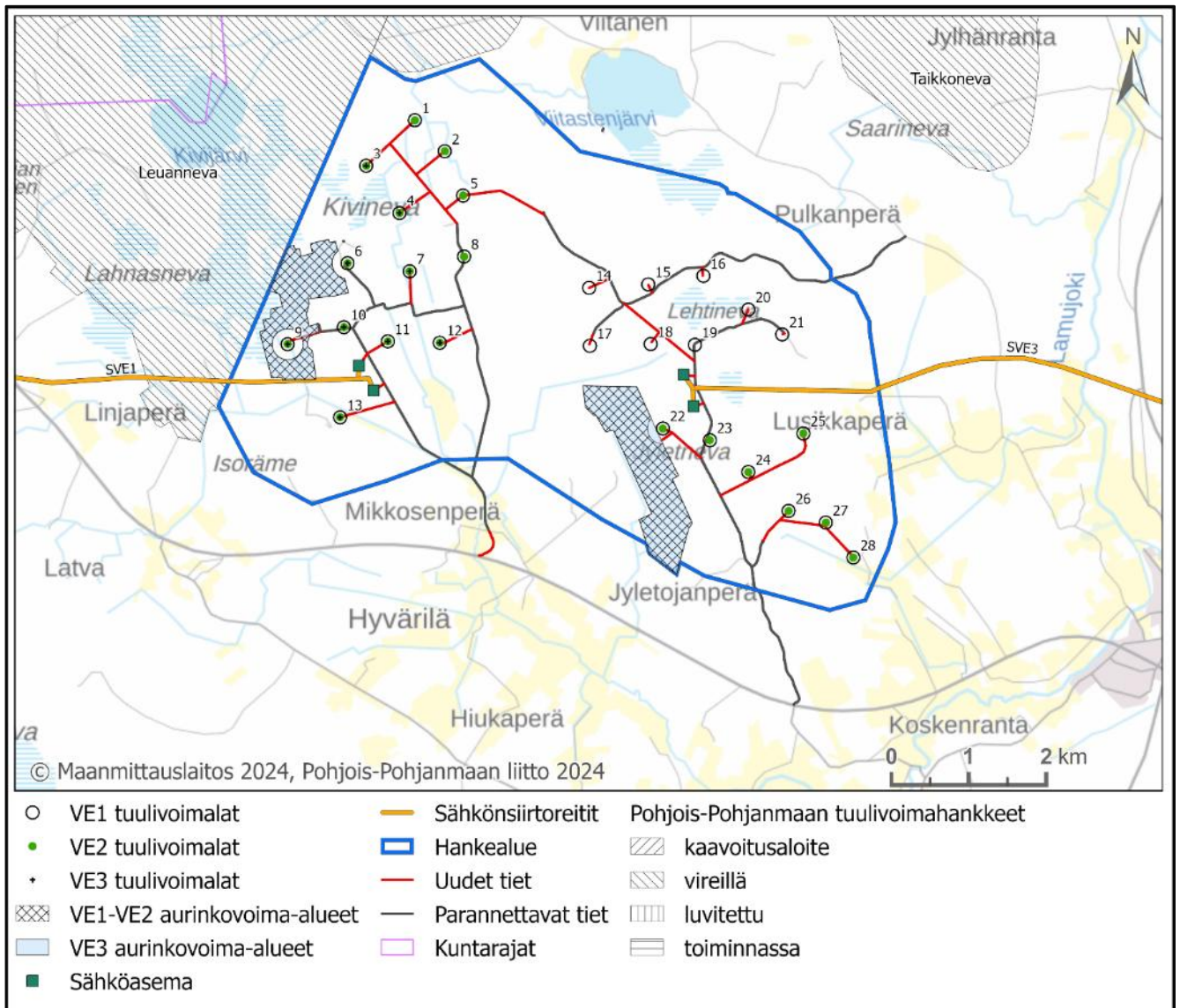
Kuva 2. Hankealue, tuuli- ja aurinkovoima-alueet sekä alueen uudet ja levennettävät tiet. Vaihtoehdossa VE1 ovat mukana tuulivoimalat 1–28, VE2 voimalat 1–13 sekä 22–28 ja VE3 voimalat 3–4, 6–7 sekä 9–13.
