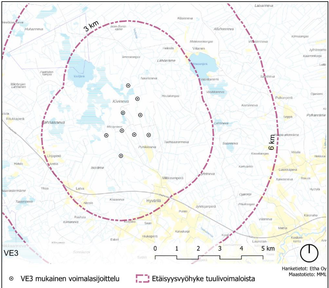
Kuva 114. VE3 mukainen voimalasijoittelu.
