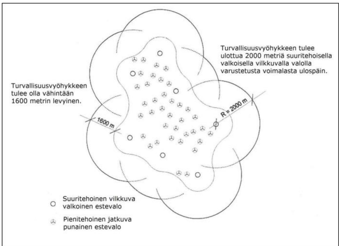
Kuva 15. Esimerkki tuulivoima-alueen lentoestevalojen ryhmittämisestä (Traficom), kun voimaloiden lapojen korkein pyyhkäisykohta on yli 150 m maanpinnasta.
