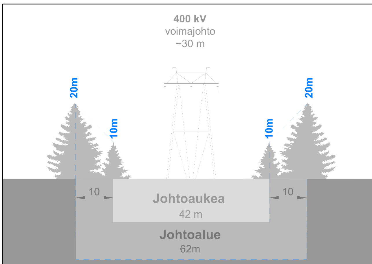
Kuva 34. Periaatekuva johtoalueesta, kun alueelle sijoittuu yksi 400 kV voimajohtolinja.
