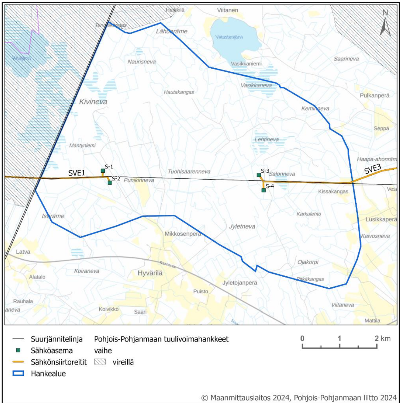
Kuva 32. SVE1 ja SVE3 vaihtoehtojen noin 170 m – 240 m pituinen osuus Vihanti-Pulkila suurjännitelinjalta hankealueen sisälle rakennettavalle sähköasemalle rakennetaan uuteen johtokäytävään.
