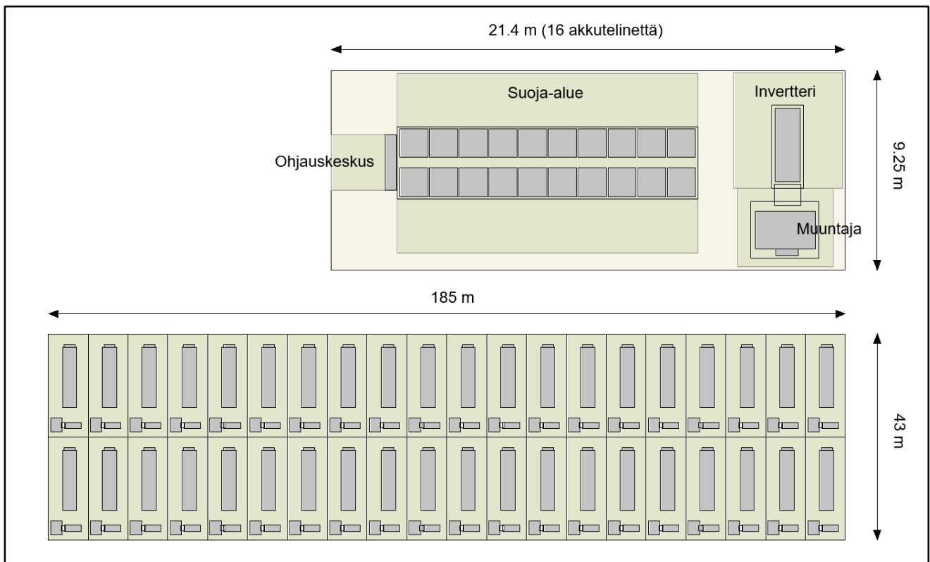
Kuva 30. Periaatekuva akkuvarastosta (A-insinöörit Suunnittelu Oy). Yläkuvassa näkyvät akkuvaraston osat. Alemmassa kuvassa on 40 ylemmässä kuvassa kuvattua 5 MWh:n moduulia, joista koostuu yhteensä 200 MWh:n akkuvarasto.
