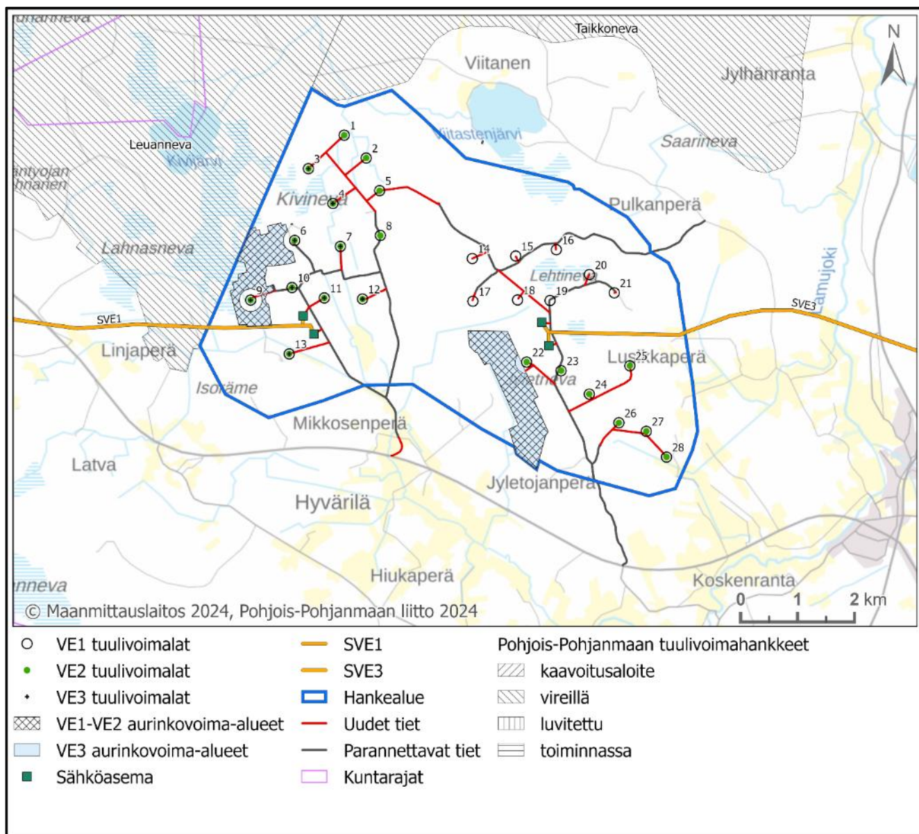
Kuva 26. Hankealueen suunniteltu tiestö.
