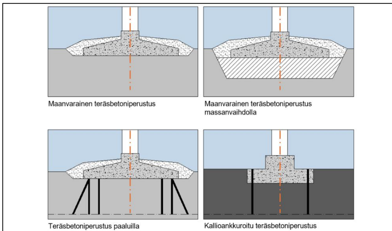
Kuva 13. Periaatekuva tuulivoimalan erilaisista perustamistavoista. (A-insinöörit)
