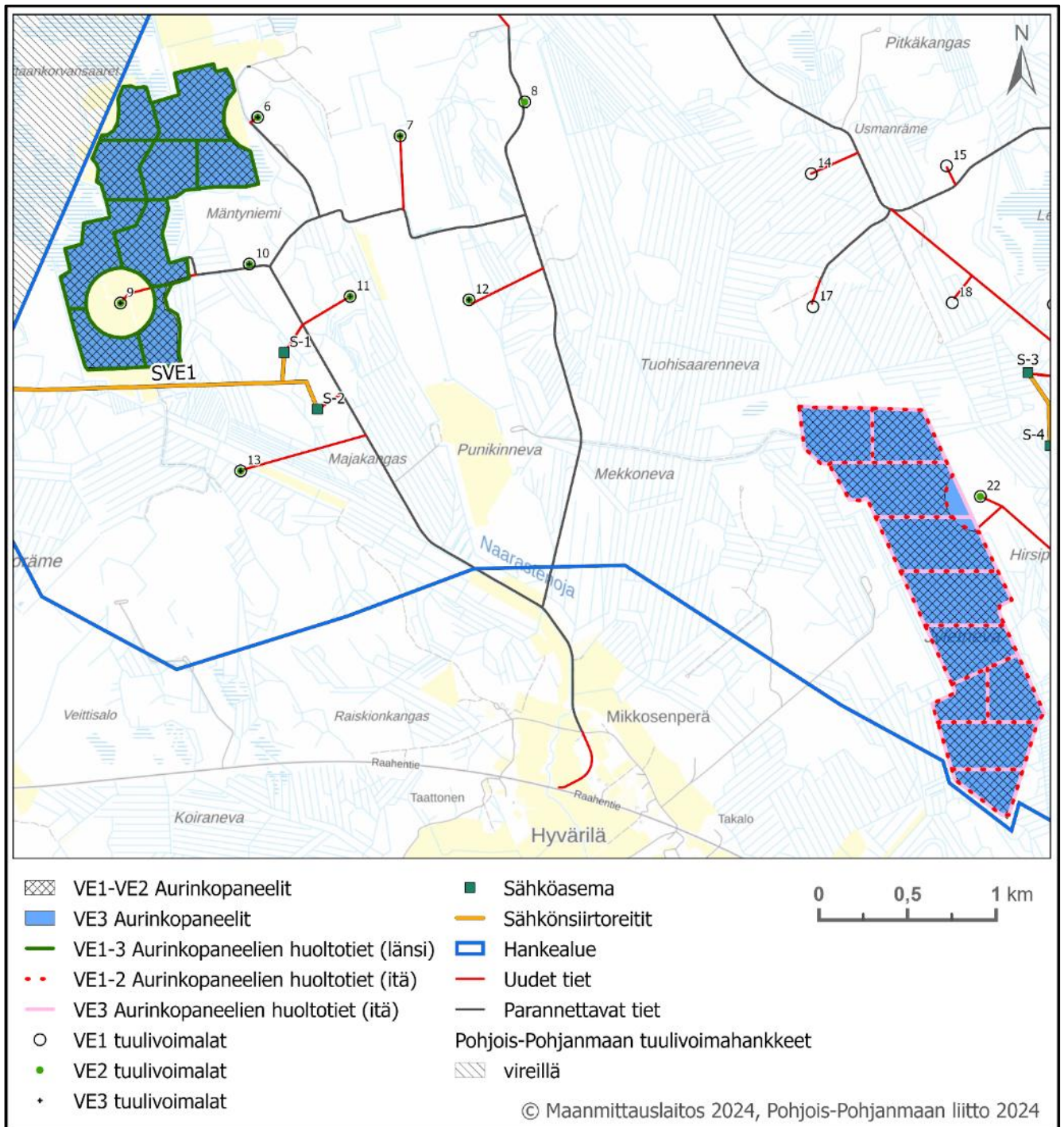
Kuva 22. Suunnitelma aurinkopaneelien ja niiden edellyttämien huoltoteiden sijoittamisesta.
