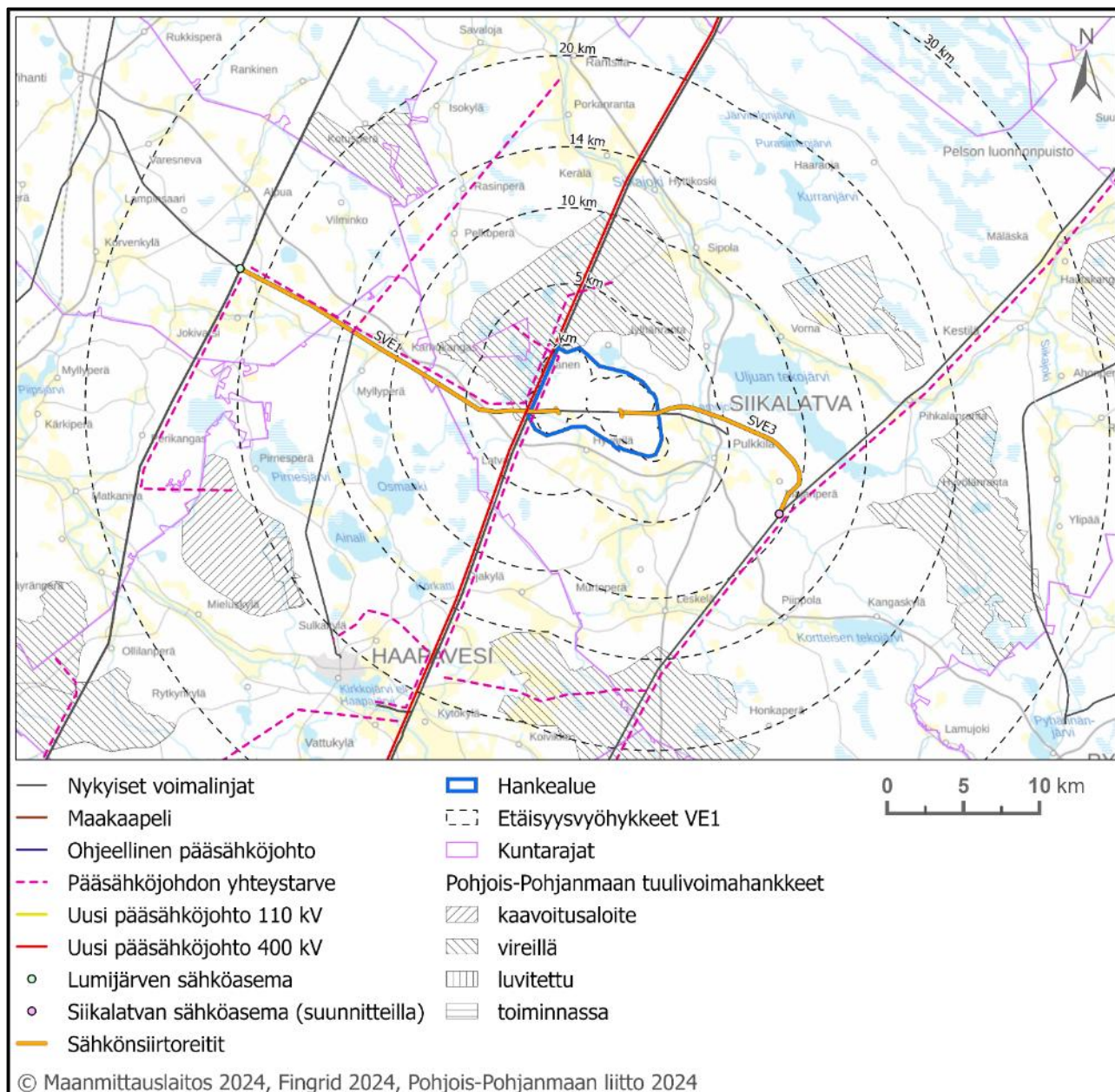
Kuva 10. Kivinevan sähkönsiirtovaihtoehdot sekä muut suunnitellut sähkönsiirtoreitit lähialueella (pääsähköjohdon yhteystarve). Etäisyysvyöhykkeet kartalla ovat etäisyyksiä VE1-voimaloista.
