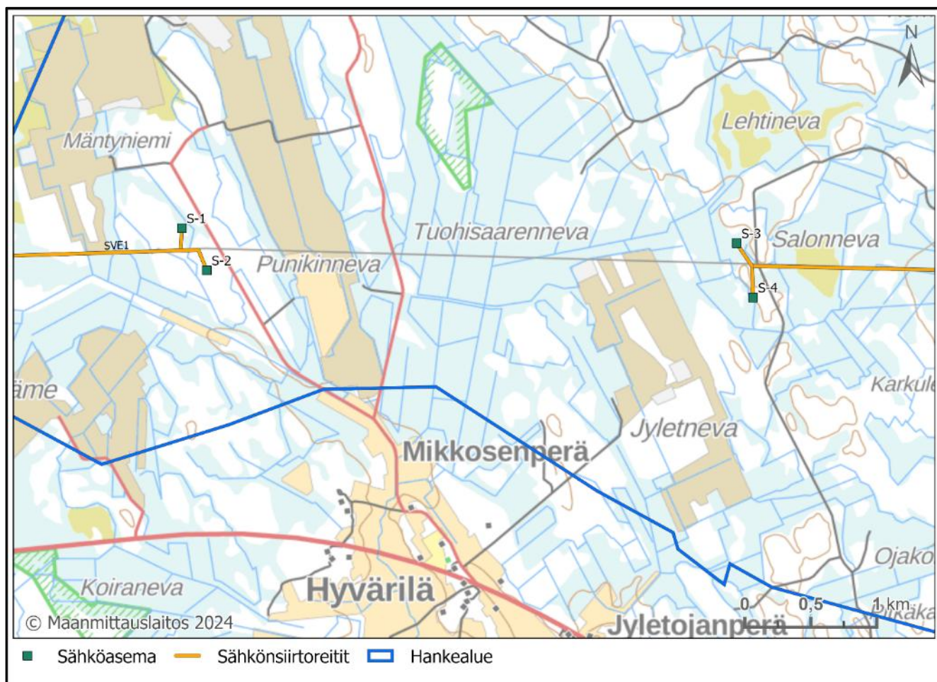
Kuva 5. Hankkeessa rakennettavan sähköaseman vaihtoehtoiset sijoituspaikat. Sähköaseman yhteyteen sijoitetaan myös akkuvarasto.
