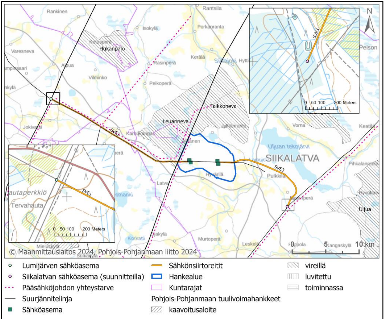
Kuva 4. Vaihtoehtoiset sähkönsiirtoreitit ja liityntäpisteet. Liityntäpisteistä Lumijärven sähköasemalle lännessä (SVE1) ja Siikalatvan sähköasemalle idässä (SVE3) on esitetty karttasuurennot. Kartalla näkyvät myös Pohjois-Pohjanmaan liiton aineistoissa tunnistetut pääsähköjohtojen yhteystarpeet.
