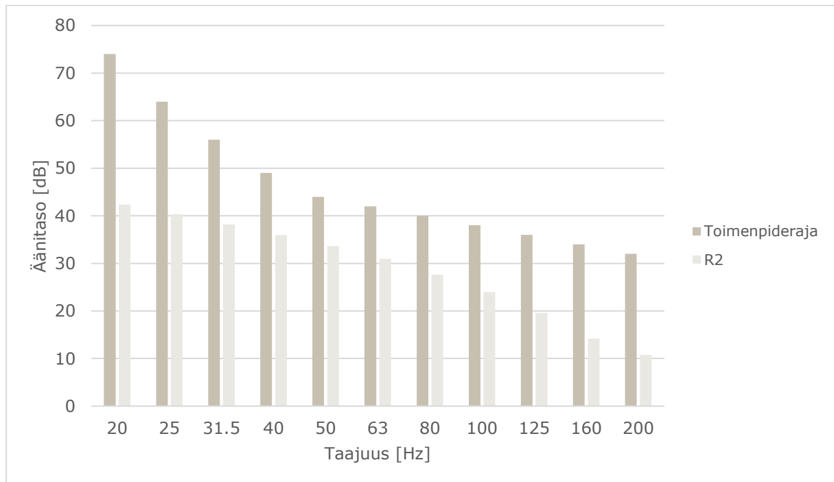
Kuva 5: Matalataajuisen sisämelun tasot reseptorin R2 kohdalla.
