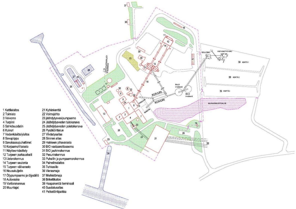
Kuva 2-7. Pyrolyysiprosessiin perustuvan bioöljylaitoksen alustava asemapiirros. Suurempi kuva selostuksen liitteessä 4.
