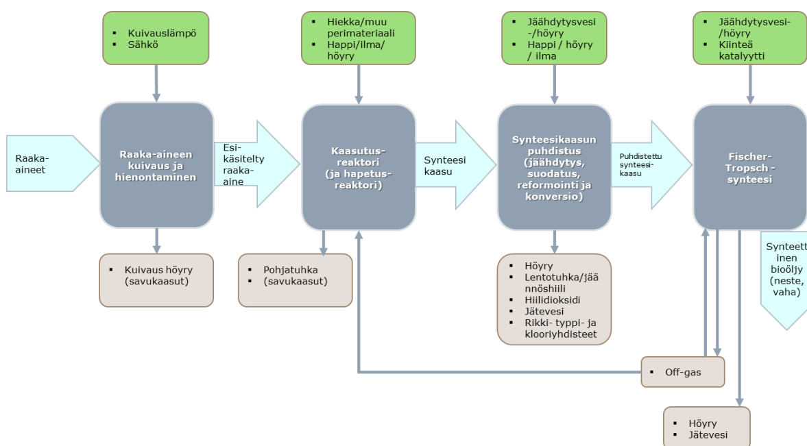
Kuva 2-8. Synteetiprosessi
