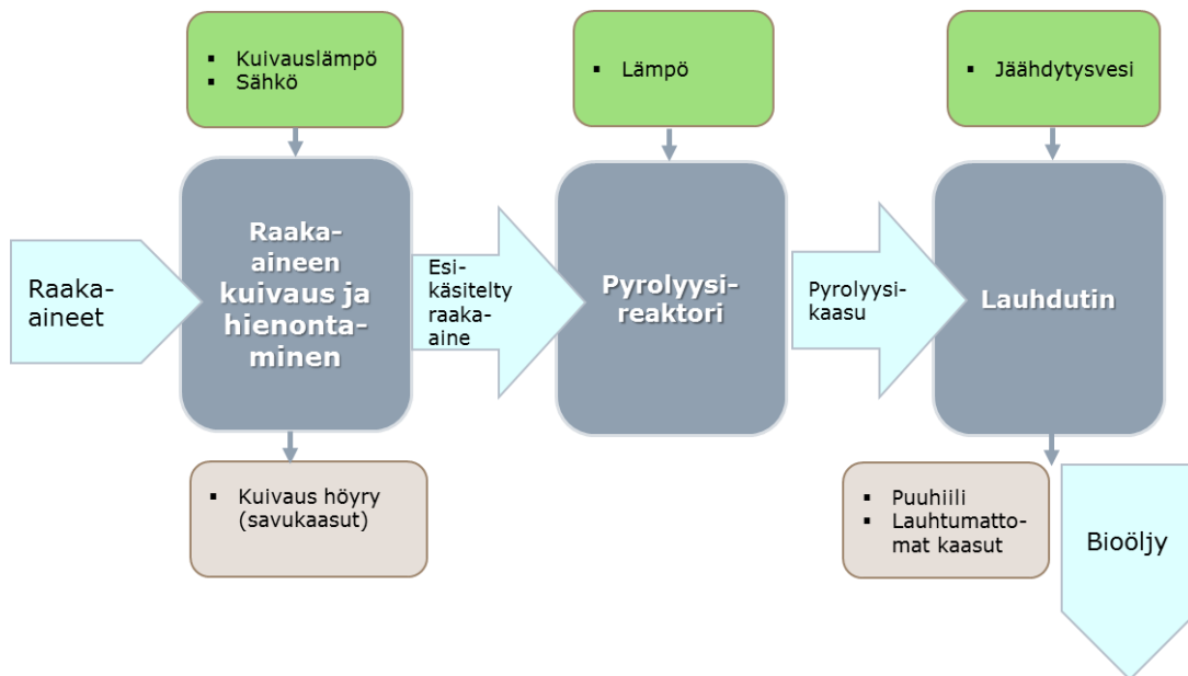
Kuva 2-6. Pyrolyysiprosessi.
