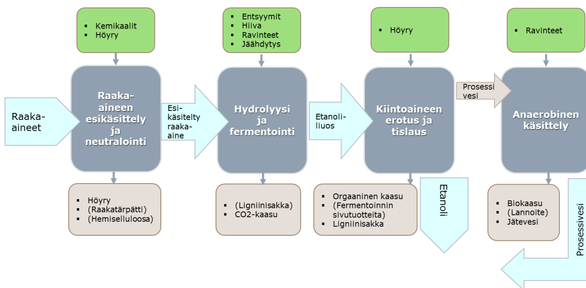
Kuva 2-4. Bioetanoliprosessi.
