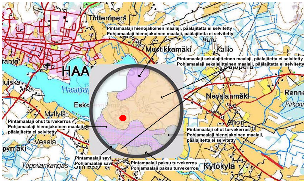
Kuva 5-28. Maalajit hankealueen lähiympäristössä luokiteltuna mukautettua rakennusteknistä luokittelua käyttäen. (Kuva sisältää Digitaalinen maaperäkarta 1:200 000 -aineistoa muokattuna © Geologian tutkimuskeskus 2013), hankealue esitetty punaisella pisteellä
