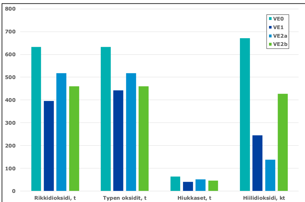
Kuva 5-26. Hanke- ja nollavaihtoehtojen voimalaitoksen savukaasupäästöjen määrät, t/a
