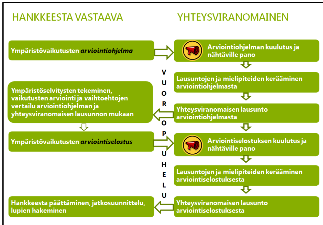
Kuva 3-1. YVA-menettelyn kulku.
