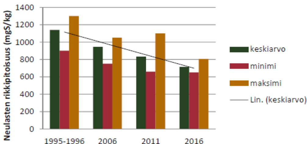
Kuva 5-25. Männyn neulasten rikkipitoisuuden kehitystrendi Haapavedellä (Lähde: Haapaveden kaupungin ilman bioindikaattoriseuranta vuonna 2016, Enwin Oy, 29.9.2016)
