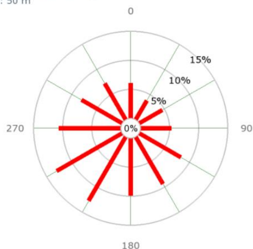
Kuva 5-24. Laskennallisesti määritetyt tuulen suuntien suhteelliset osuudet (%) 50 metrin korkeu- dessa Haapavedellä. (Ilmatieteen laitos)
