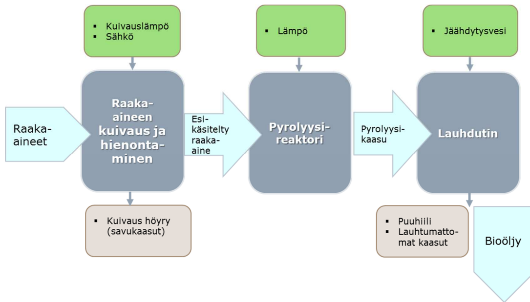
Kuva 4-5. Pyrolyysiprosessi.
