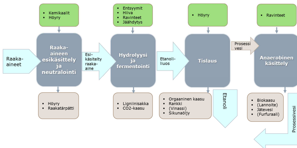
Kuva 4-4. Bioetanoliprosessi.
