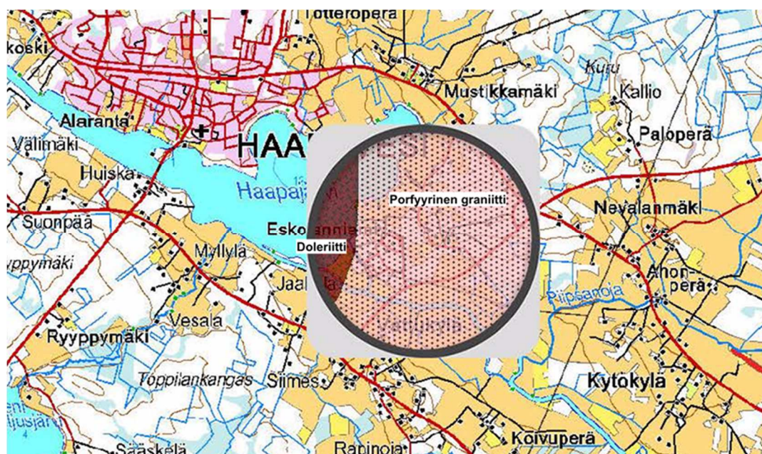
Kuva 6-6. Kallioperän kivilajit hankealueen lähiympäristössä. (Kuva sisältää Digitaalinen kallioperäkartta 1:200 000 -aineistoa muokattuna © Geologian tutkimuskeskus 2013)
