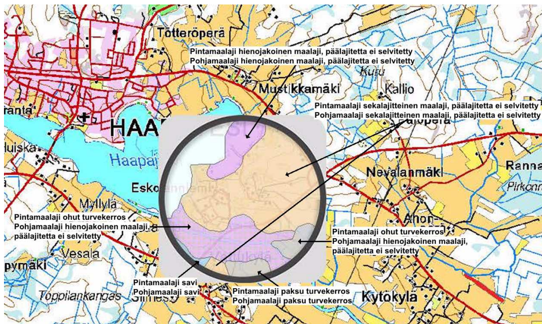
Kuva 6-7. Maalajit hankealueen lähiympäristössä luokiteltuna mukautettua rakennusteknistä luokit- telua käyttäen. (Kuva sisältää Digitaalinen maaperäkartta 1:200 000 -aineistoa muokattuna © Geologian tutkimuskeskus 2013)
