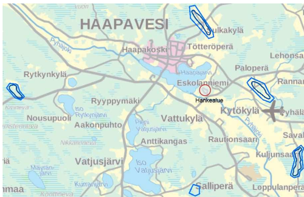
Kuva 6-8. Pohjavesialueet. (Lähde: Ympäristötietokarttapalvelu Karpalo, 19/9/2016)
