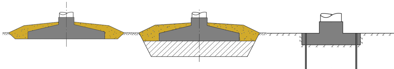
Kuva 2-11. Tuulivoimalat voidaan perustaa useilla eri tavoilla. Periaatekuvat maavaraisesta teräsbetoniperustuksesta, teräsbetoniperustuksesta massanvaihdon kanssa sekä kallioankkuroidusta teräsbetoniperustuksesta.
