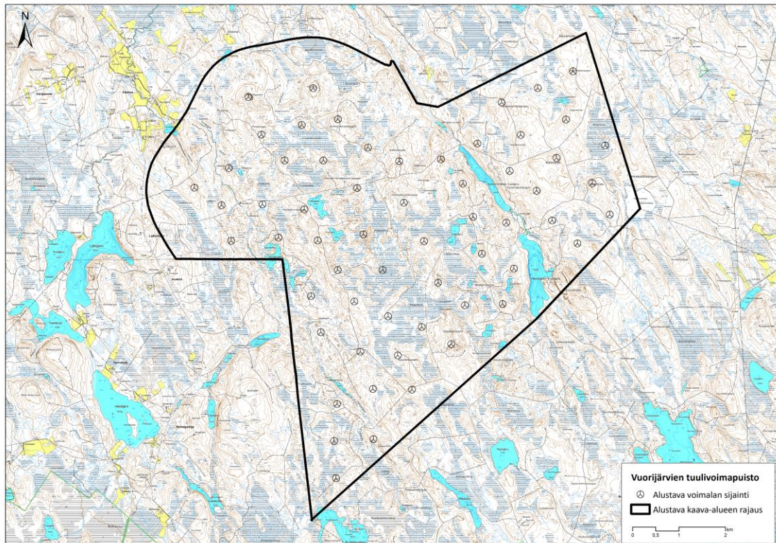
Kuva 2-4. Kannonkosken Vuorijärvien tuulivoimapauston alustava voimalasijoittelu.
