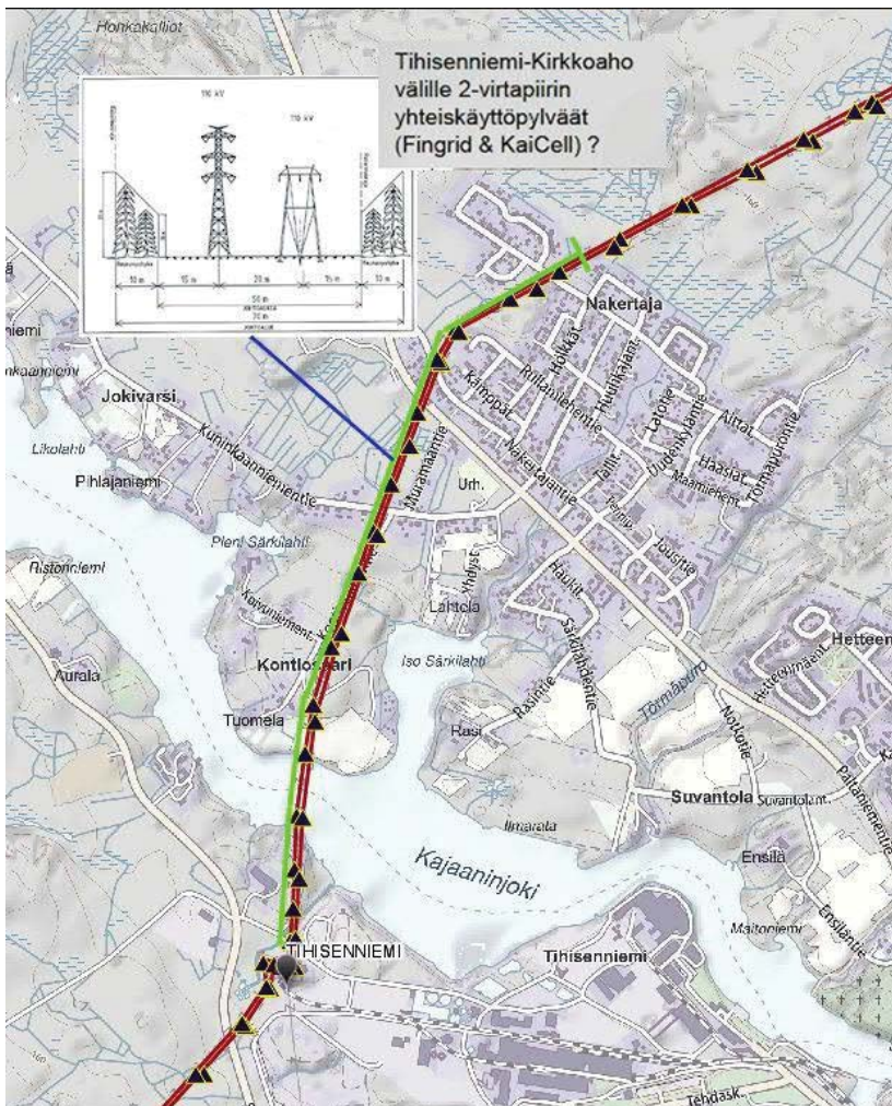
Kuva 9. Välille Nakertaja - Tihisenniemi: yhteiskäyttöpylväät.
