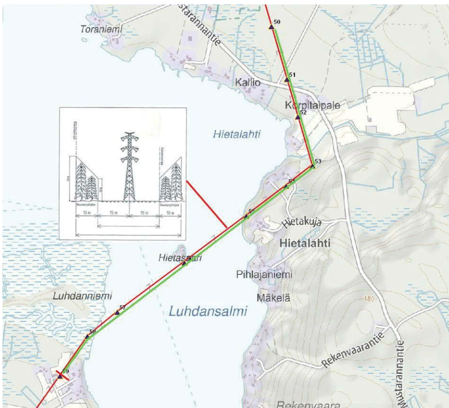
Kuva 5. Jormuanlahden ylitys: yhteiskäyttöpylväät.
