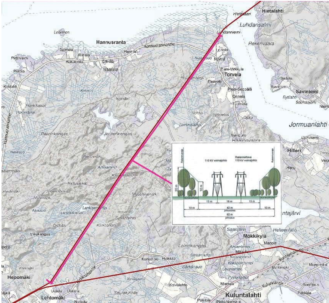
Kuva 6. Väliille Jormuanlahti – Lehtomäki: uusi voimajohto nykyisen johdon itäpuolelle.
