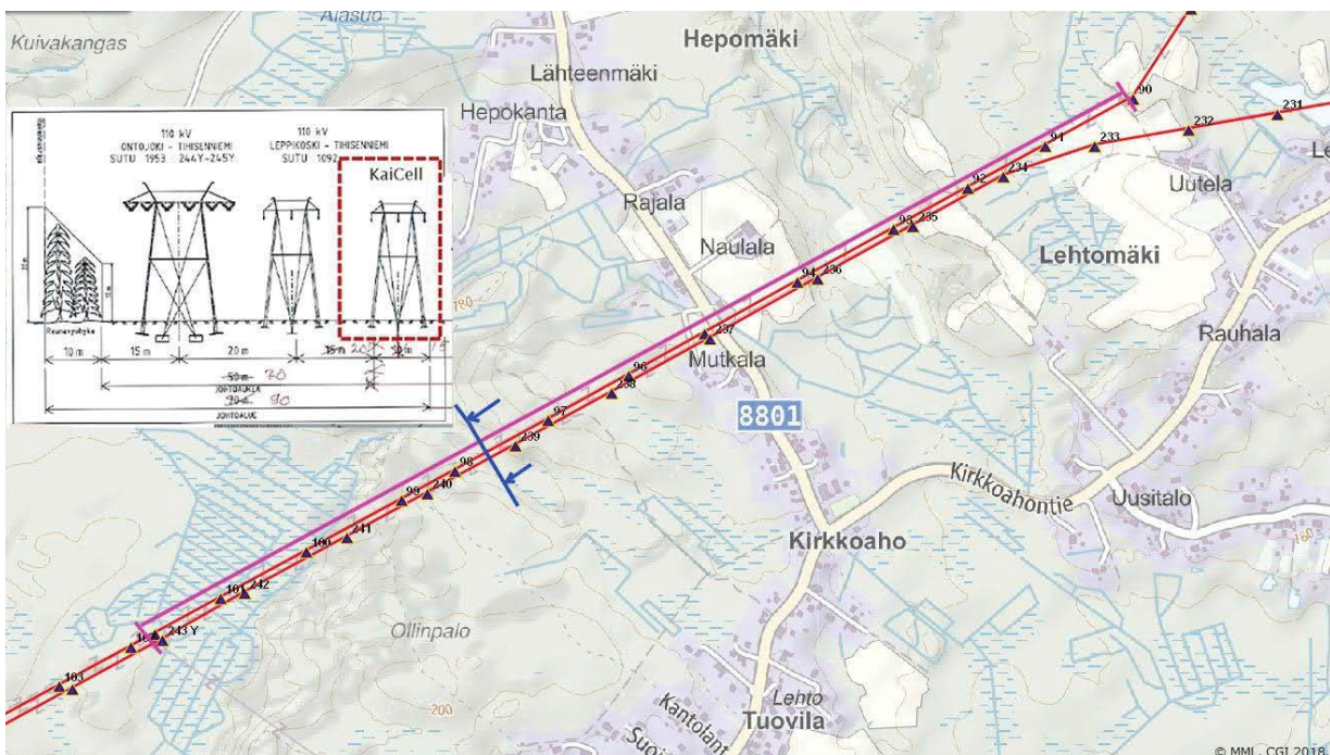
Kuva 7. Väliille Lehtomäki – Kirkkoaho: uusi voimajohto nykyisen johdon pohjoispuolelle.
