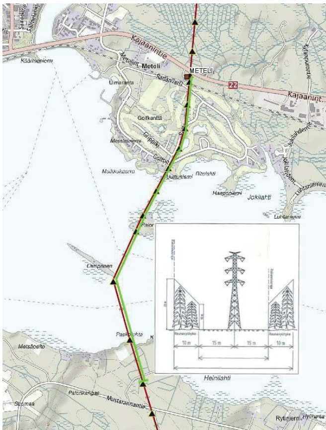
Kuva 2. Golfkentän ja Mieslahden ylitys: yhteiskäyttöpylväät.
