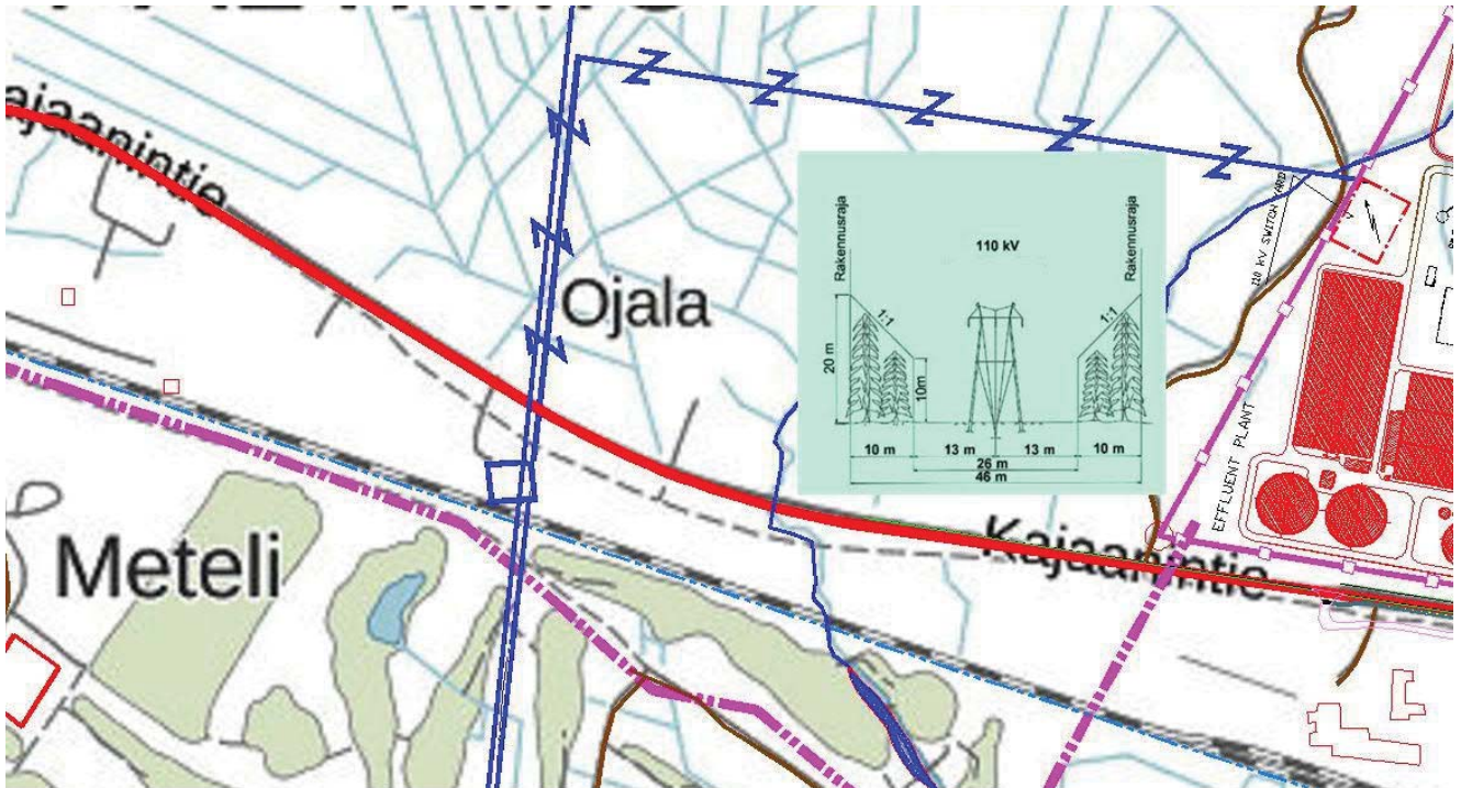
Kuva 1. Välille KAICell tehdasalue – Meteli: uusi voimajohto.
