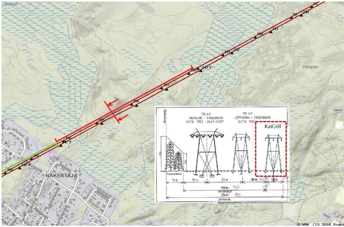
Kuva 8. Välille Kirkoaho - Nakertaja: uusi voimajohto nykyisen johdon pohjoispuolelle.
