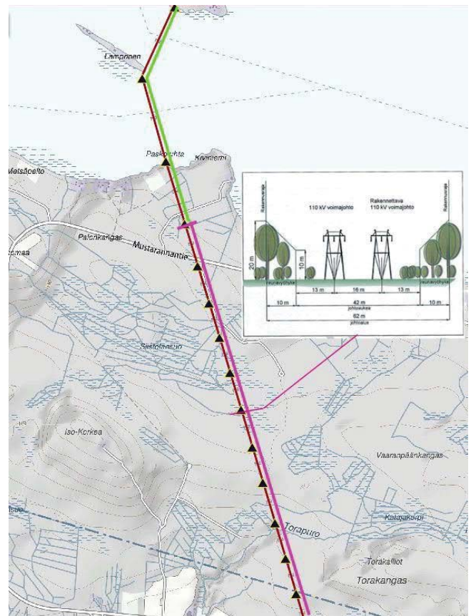
Kuva 3. Saviniemen ylitys: uusi voimajohto nykyisen johdon itäpuolelle:
