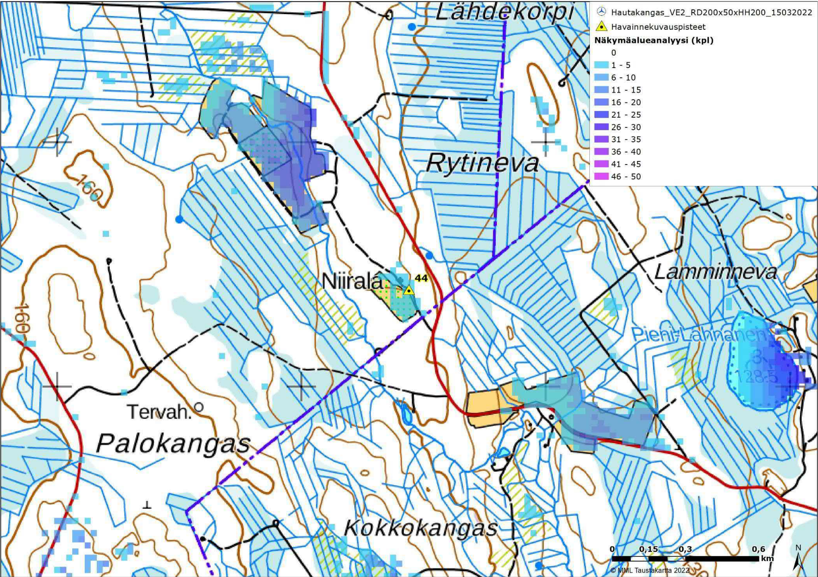
Kuva 78. Kuvauspaikka 44 ja näkymäalueanalyysi VE2. Voimalat sijaitsevat kuvauspisteestä lounaaseen - pohjoiseen päin.
