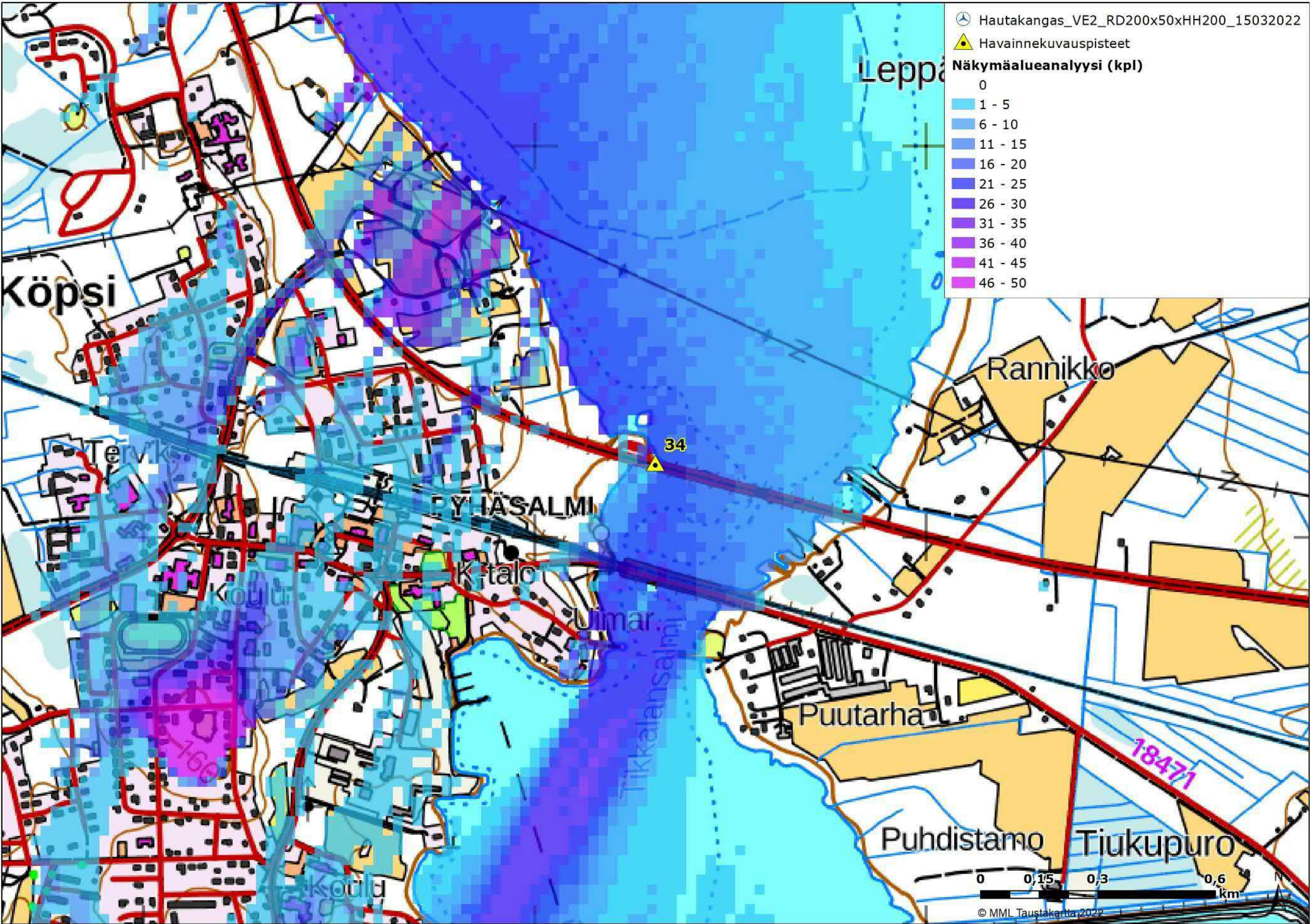
Kuva 36. Kuvauspaikka 34 ja näkymäalueanalyysi VE2. Voimalat sijaitsevat kuvauspisteestä pohjoiseen - koilliseen päin.
