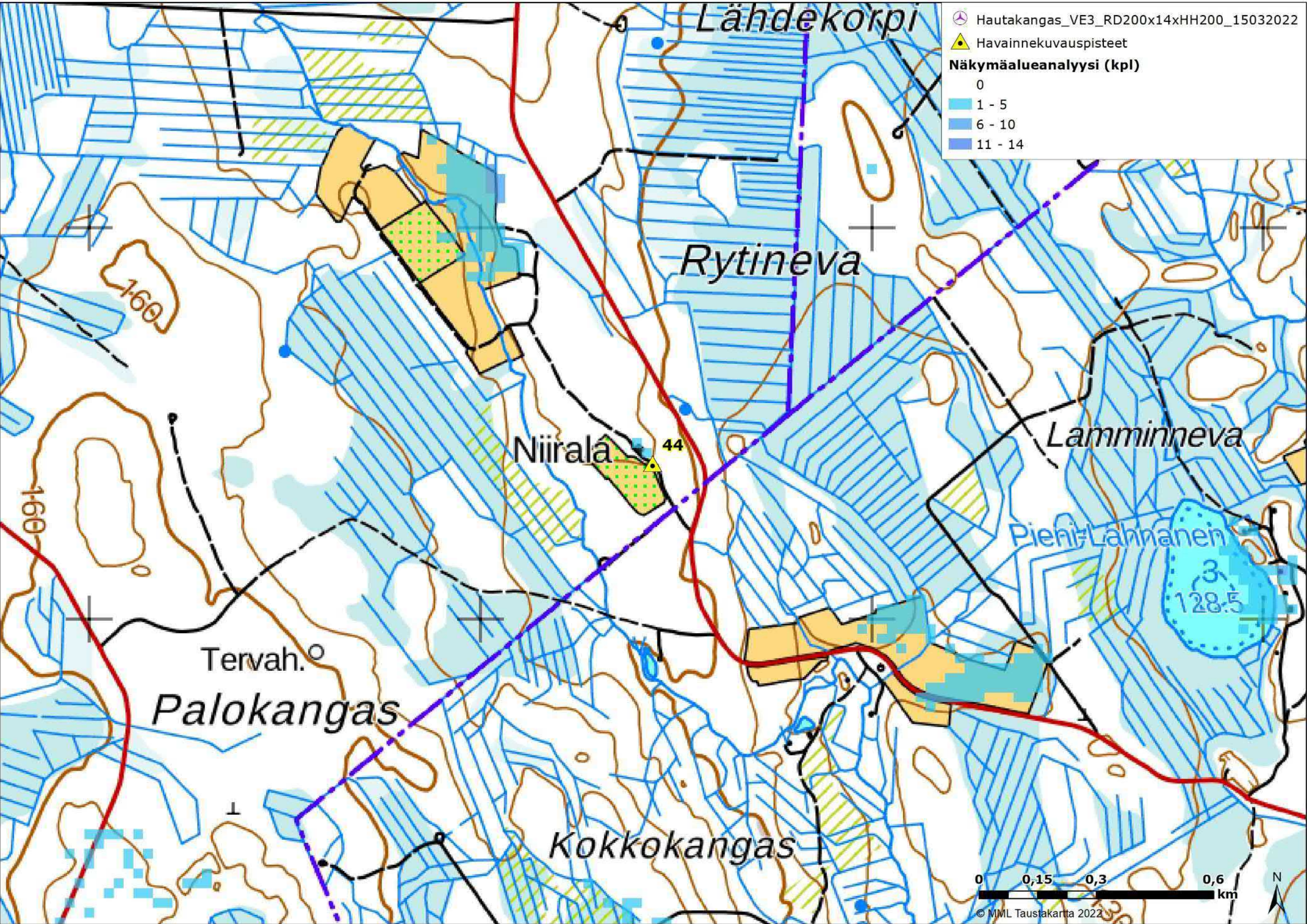
Kuva 81. Kuvauspaikka 44 ja näkymäalueanalyysi VE3. Voimalat sijaitsevat kuvauspisteestä lounaaseen päin.
