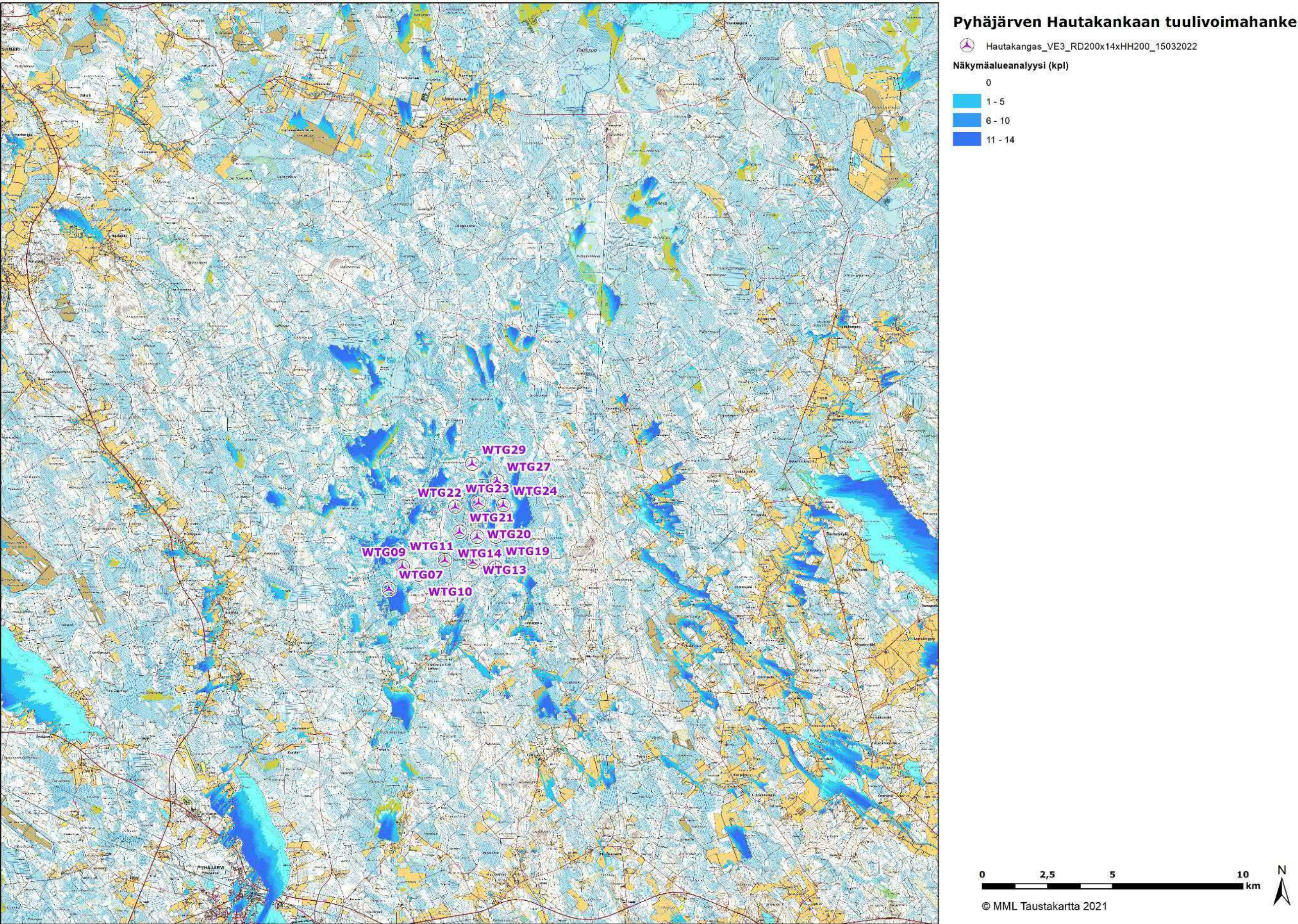
Kuva 3. Hautakankaan tuulivoimahankkeen vaihtoehdon 3 (VE3) näkymäalueanalyysin laskentatulokset voimaloiden napakorkeudella mallinnettuna. Voimaloiden napakorkeus on 200 m ja kokonaiskorkeus 300 m.
