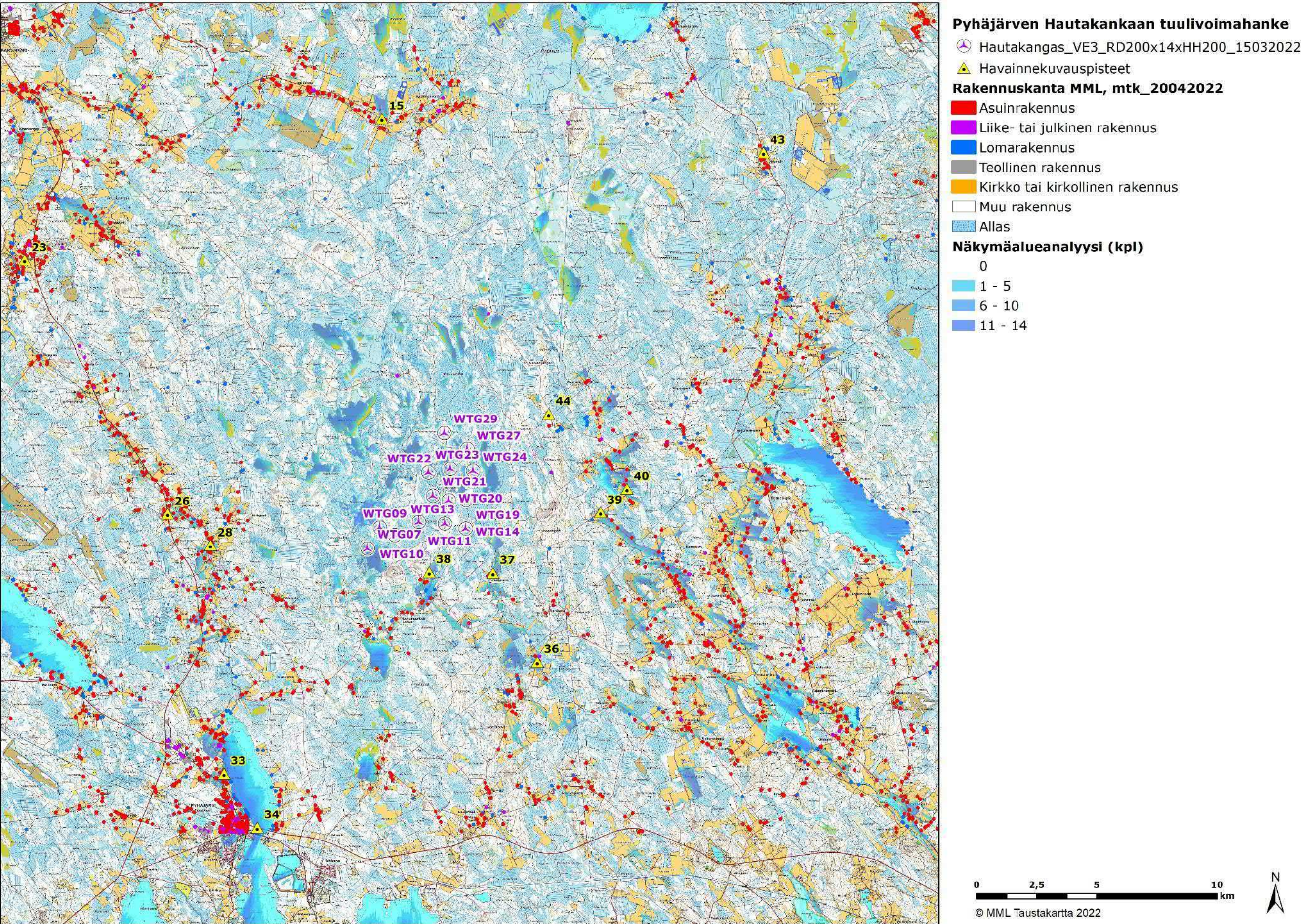
Kuva 5. Hautakankaan tuulivoimahankkeen vaihtoehdon 3 (VE3) näkymäalueanalyysin laskentatulokset, asutus ja kuvauspisteet (13 kpl).
