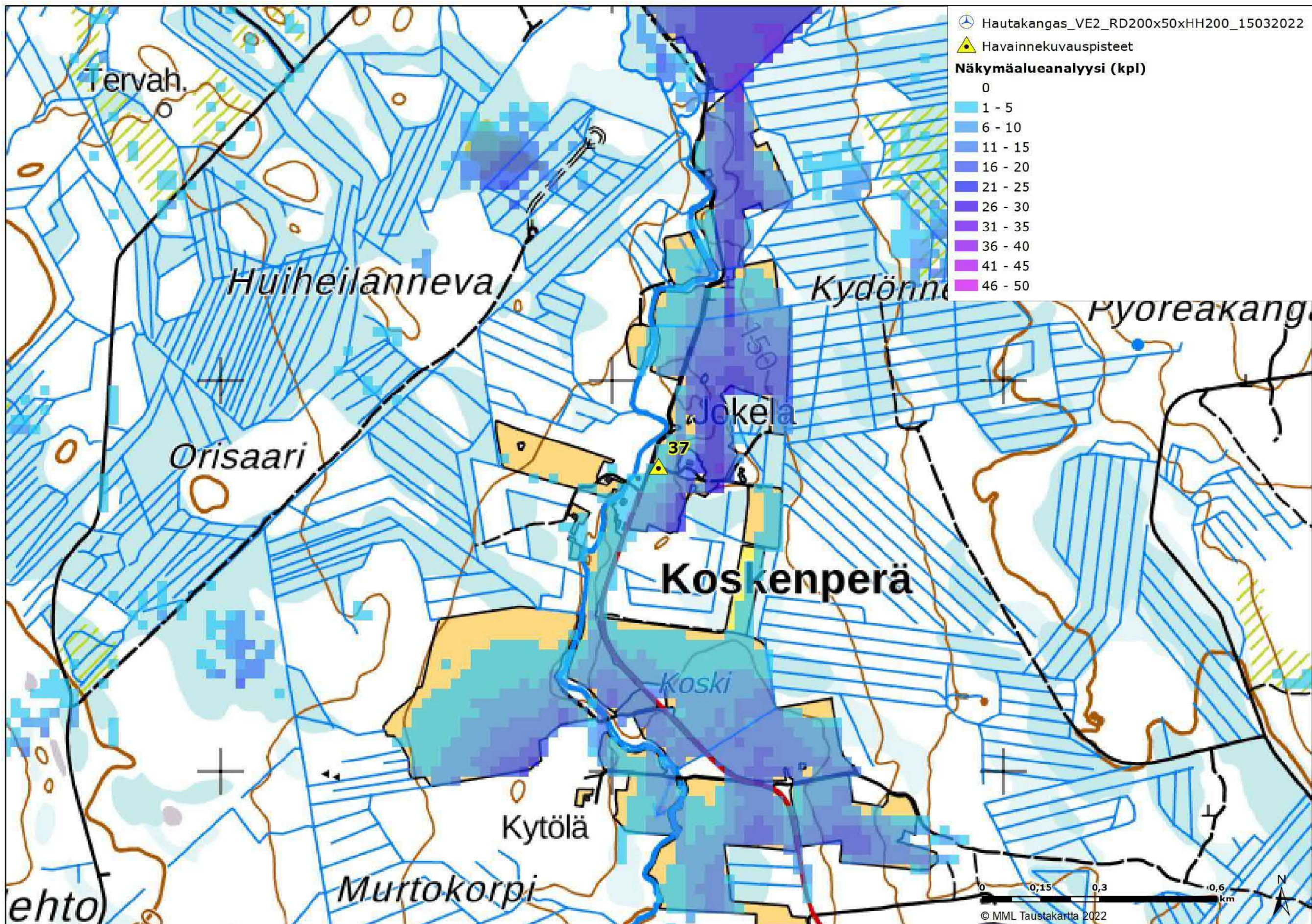
Kuva 48. Kuvauspaikka 37 ja näkymäalueanalyysi VE2. Voimalat sijaitsevat kuvauspaikasta luoteeseen - pohjoiseen päin.
