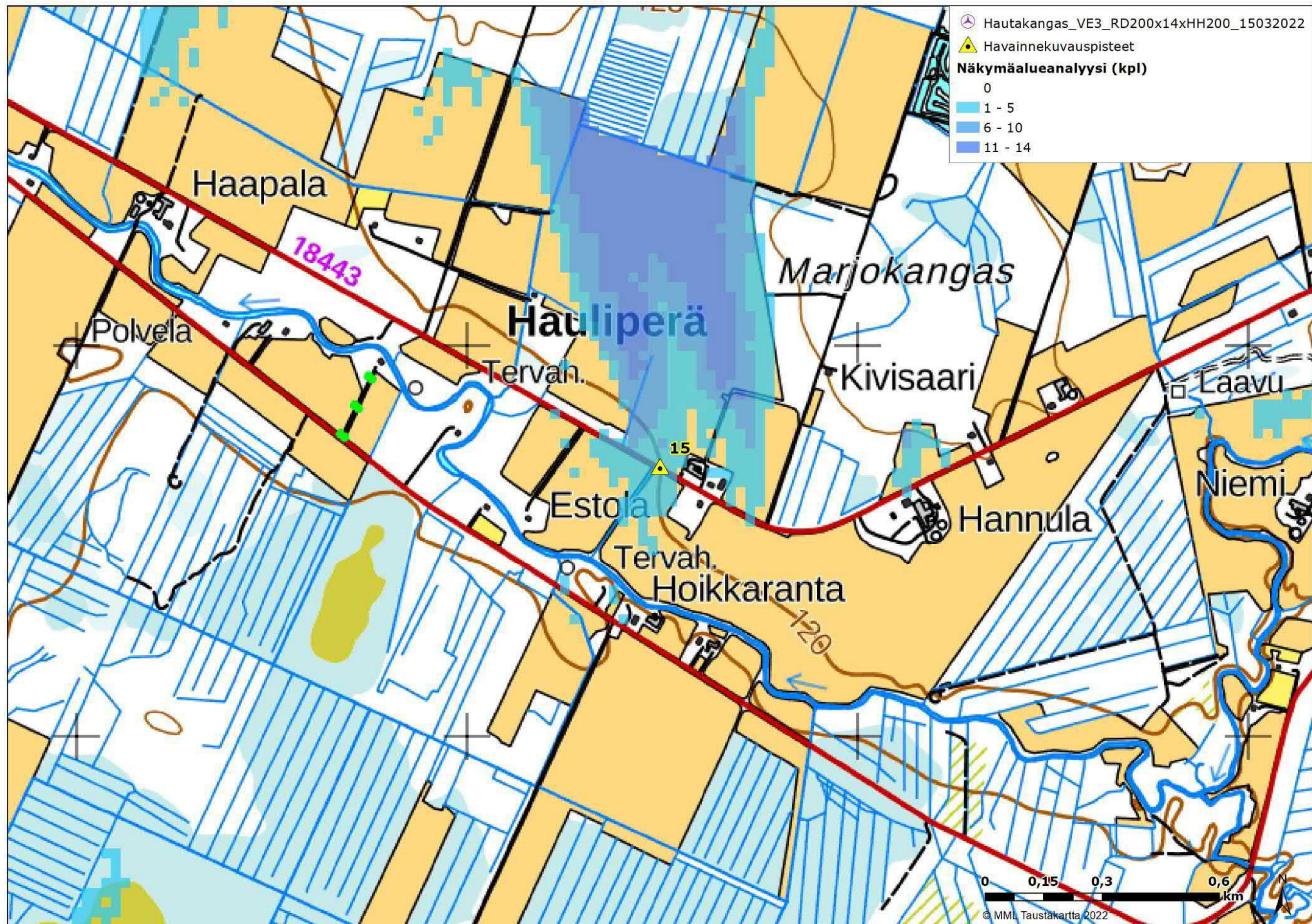
Kuva 9. Kuvauspaikka 15 ja näkymäalueanalyysi VE3. Voimalat sijaitsevat kuvauspaikkeen eteläpuolella.
