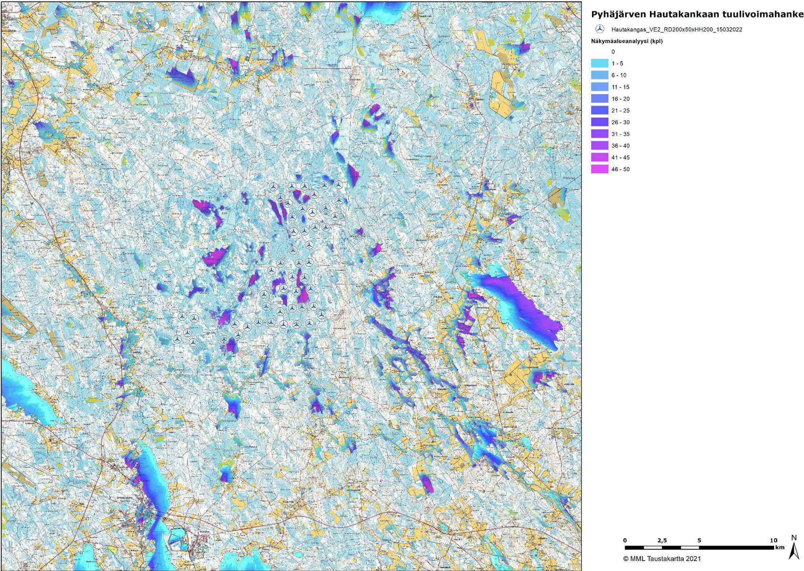
Kuva 1. Hautakankaan tuulivoimahankkeen vaihtoehdon 2 (VE2) näkymäalueanalyysin laskentatulokset voimaloiden napakorkeudella mallinnettuna. Voimaloiden napakorkeus on 200 m ja kokonaiskorkeus 300 m.
