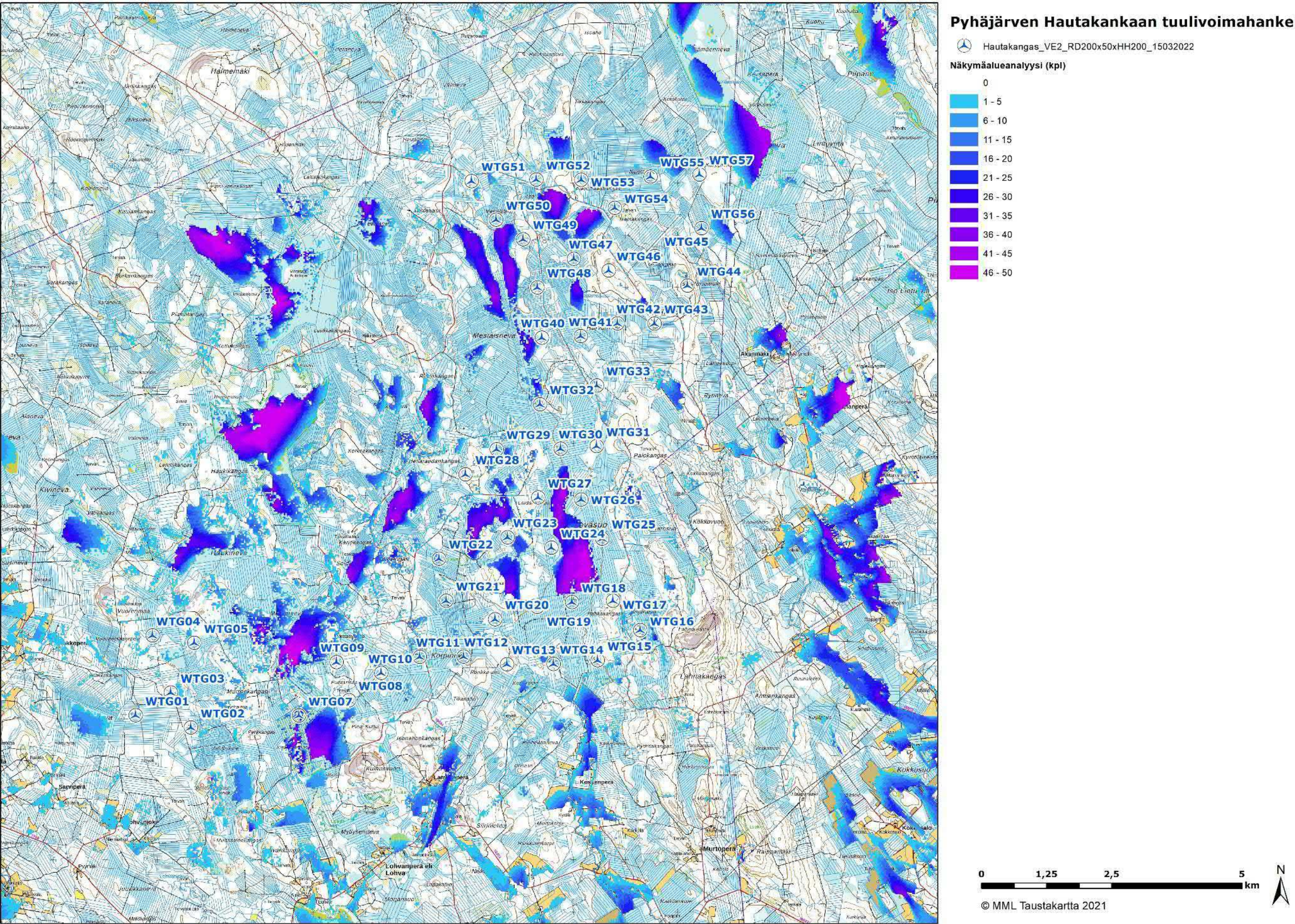
Kuva 2. Hautakankaan tuulivoimahankkeen vaihtoehdon 2 (VE2) voimaloiden numeroinnit lähialueelta.
