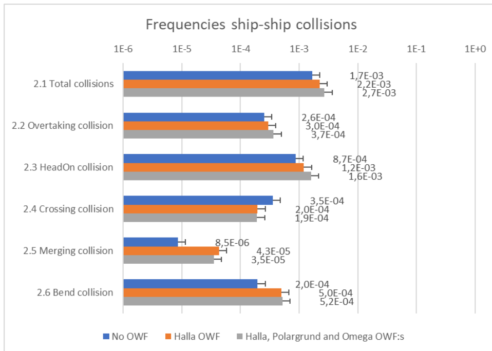
Kuva 15. Yhteentörmäystaajuus vuodessa (palkit ja numerot) Hallan ympärillä olevalla alueella logaritmisella asteikolla. Erilaisten yhteentörmäystyyppien todennäköisyys ilman merituulivoimapuistoa, jos Hallan merituulivoimapuisto otetaan käyttöön ja jos Hallan, Polargrundin ja Omegan merituulivoimapuistot kaikki otetaan käyttöön. Epävarmuuspalkit (mustat viivat) osoittavat esiintymistiheyttä tulevassa liikenneskenaariossa vuodelle 2060, jolloin alusten määrä on kasvanut 35 %. Katso toistumisjakso ja tarkemmat tiedot esiintymistiheydestä luvusta 1.3.3
