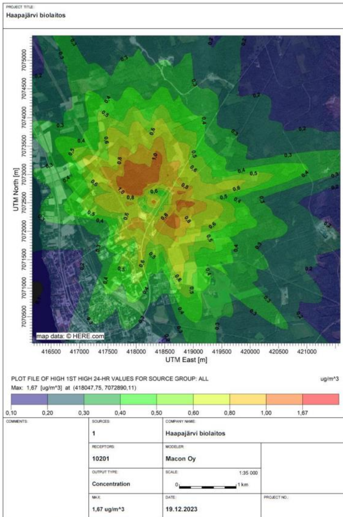
Kuva 31. Pölyn (PM 10 ) vuorokausikeskiarvopäästö Ouluntien teollisuusalueella (piippupäästöt). Raja-arvo 50 µg/m 3 ei ylity.
