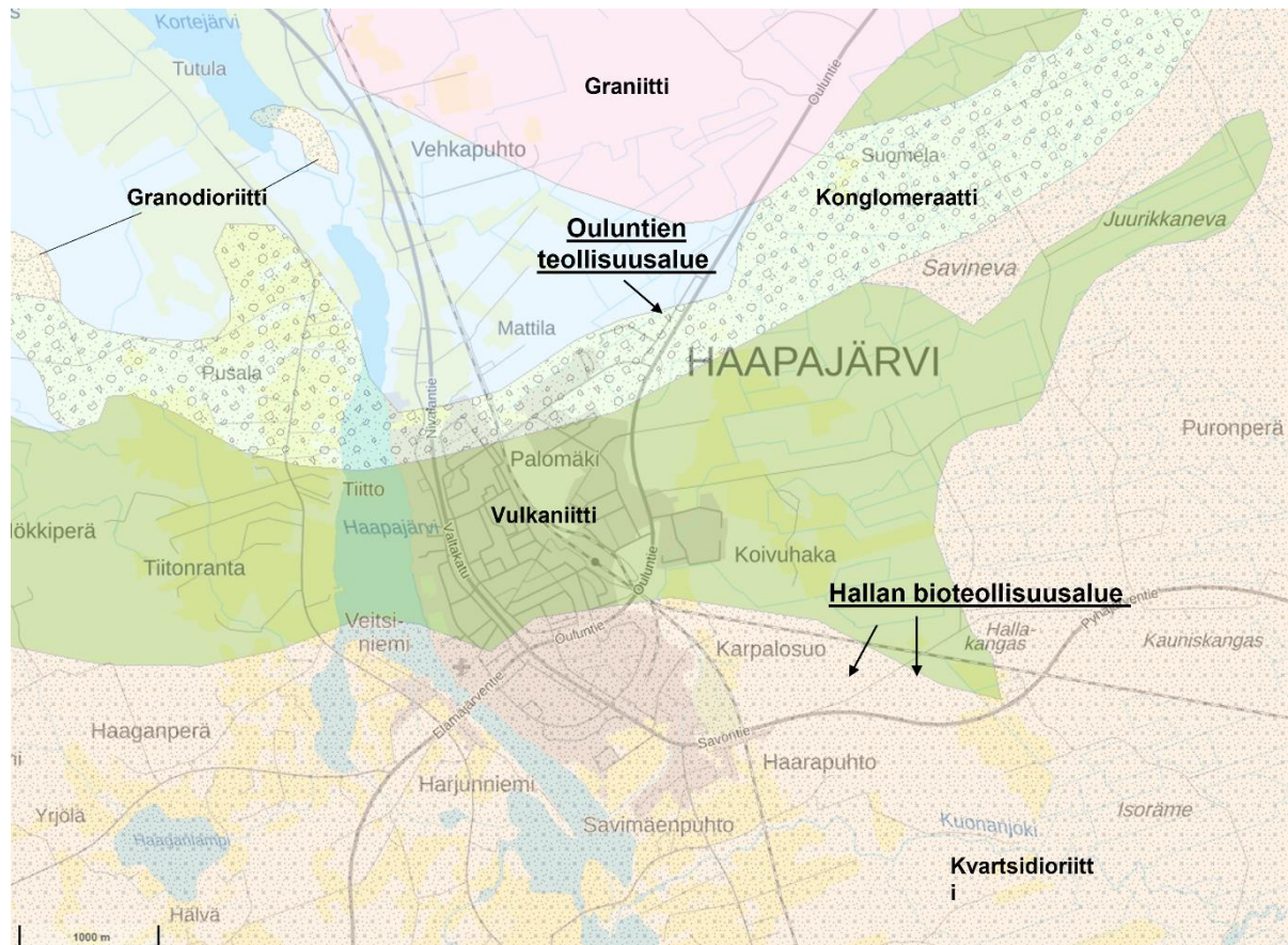
Kuva 59. Alueen kallioperä. 146
