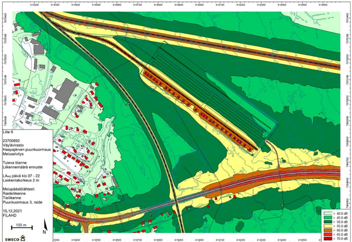
Kuva 30. Väyläviraston puunkuormaustalueen melumalli tulevasta melusta, kun puunkuormausta tapahtuisi lähimpänä asutusta (raiteella 3).
